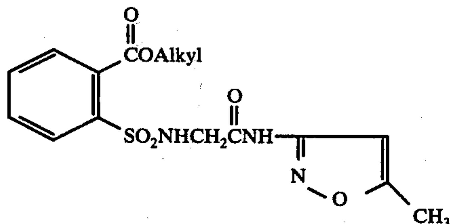
Alkyl 2-[[[(5-methyl-3-isoxazolyl)-amino]carbonyl]methyl)amino]sulfonyl}benzoate
