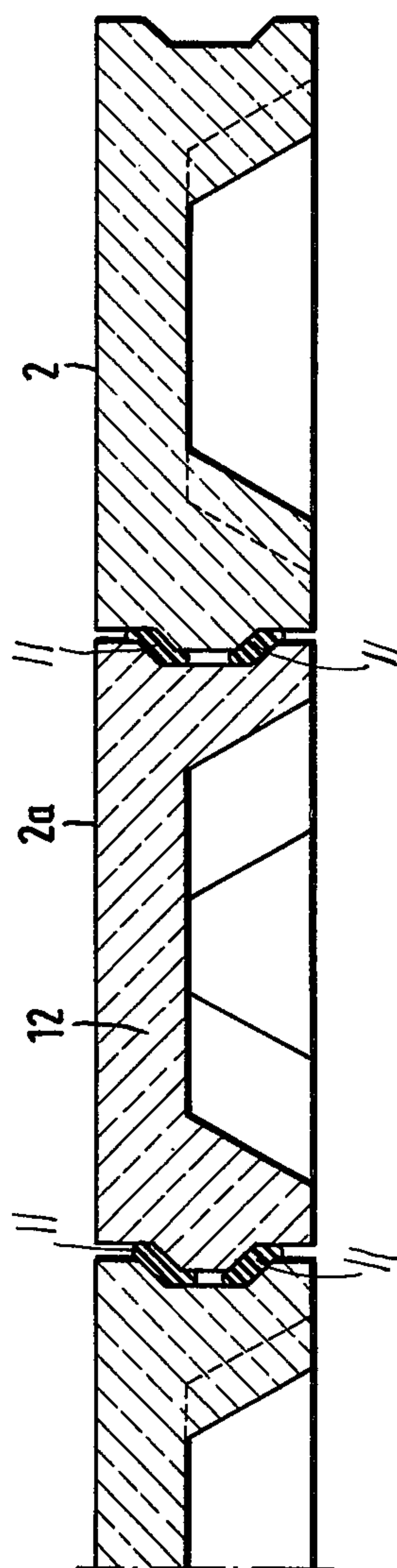
Fig. 5 (V-V)
