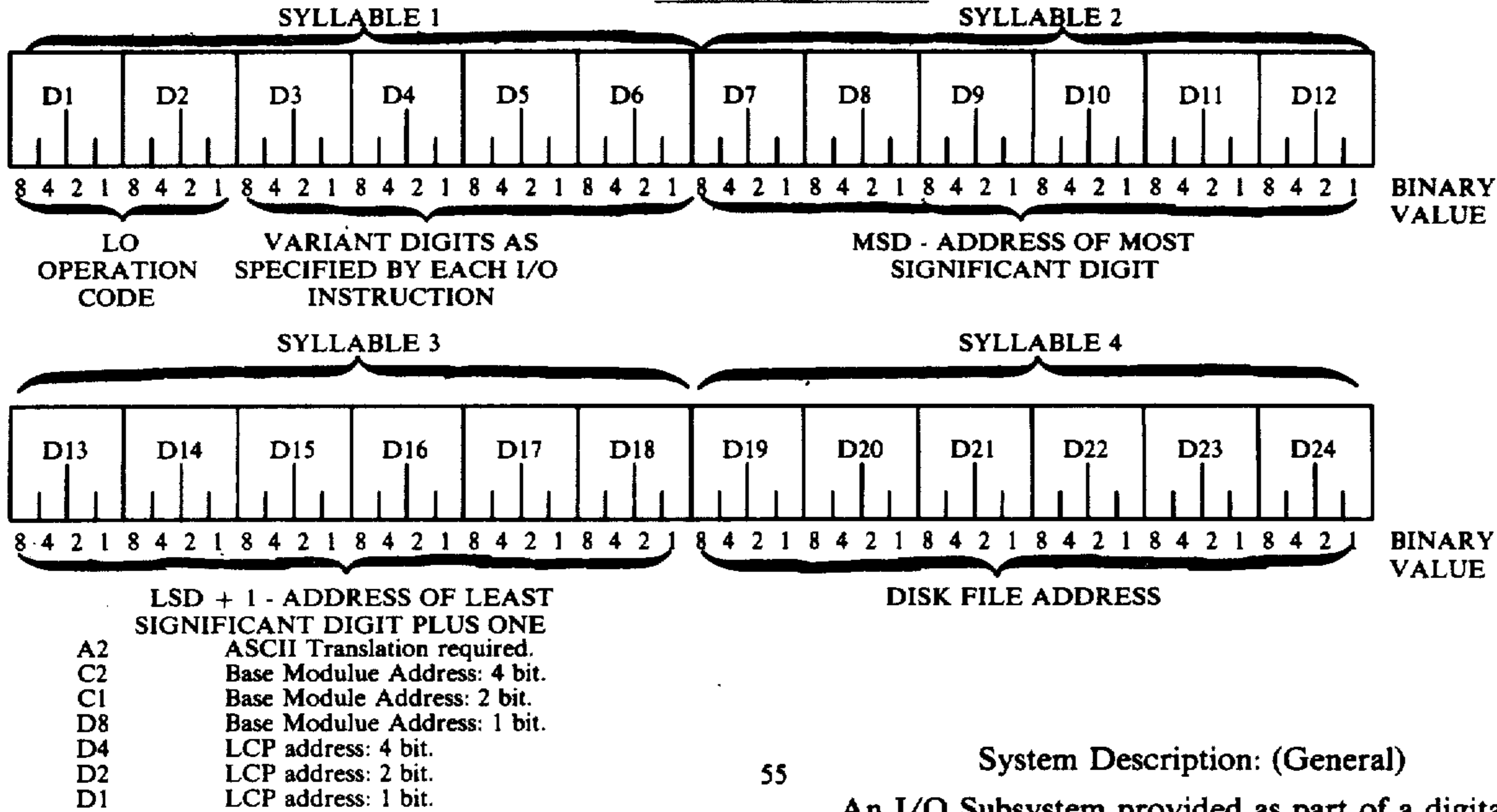
I/O Descriptor Format
