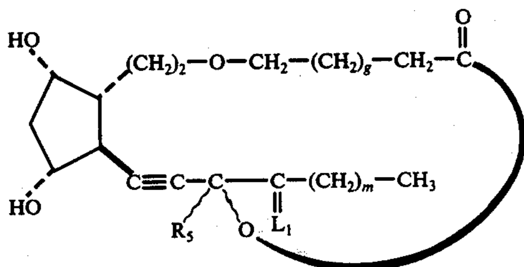
13,14-didehydro-5-oxa-PGF 1α -type, 1,15-lactones
