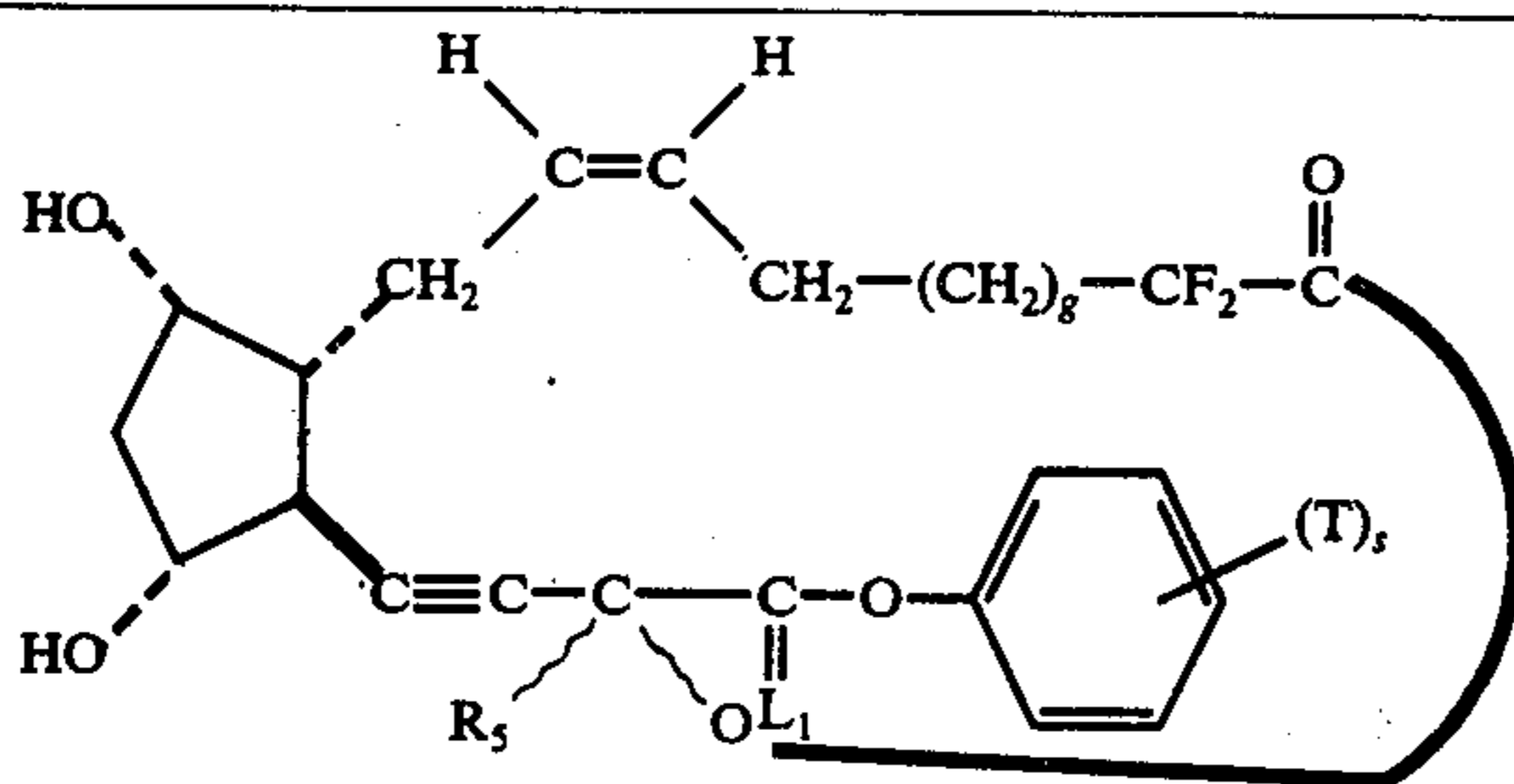
13,14-didehydro-2,2-difluoro-PGF 2α -type, 1,15-lactones
