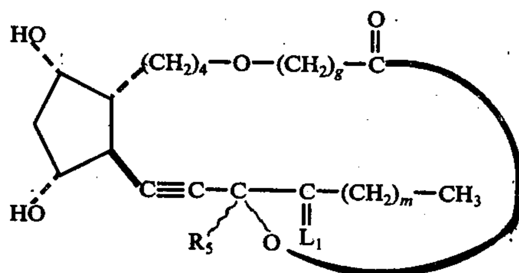
13,14-didehydro-3-oxa-PGF 1α -type, 1,15-lactones
