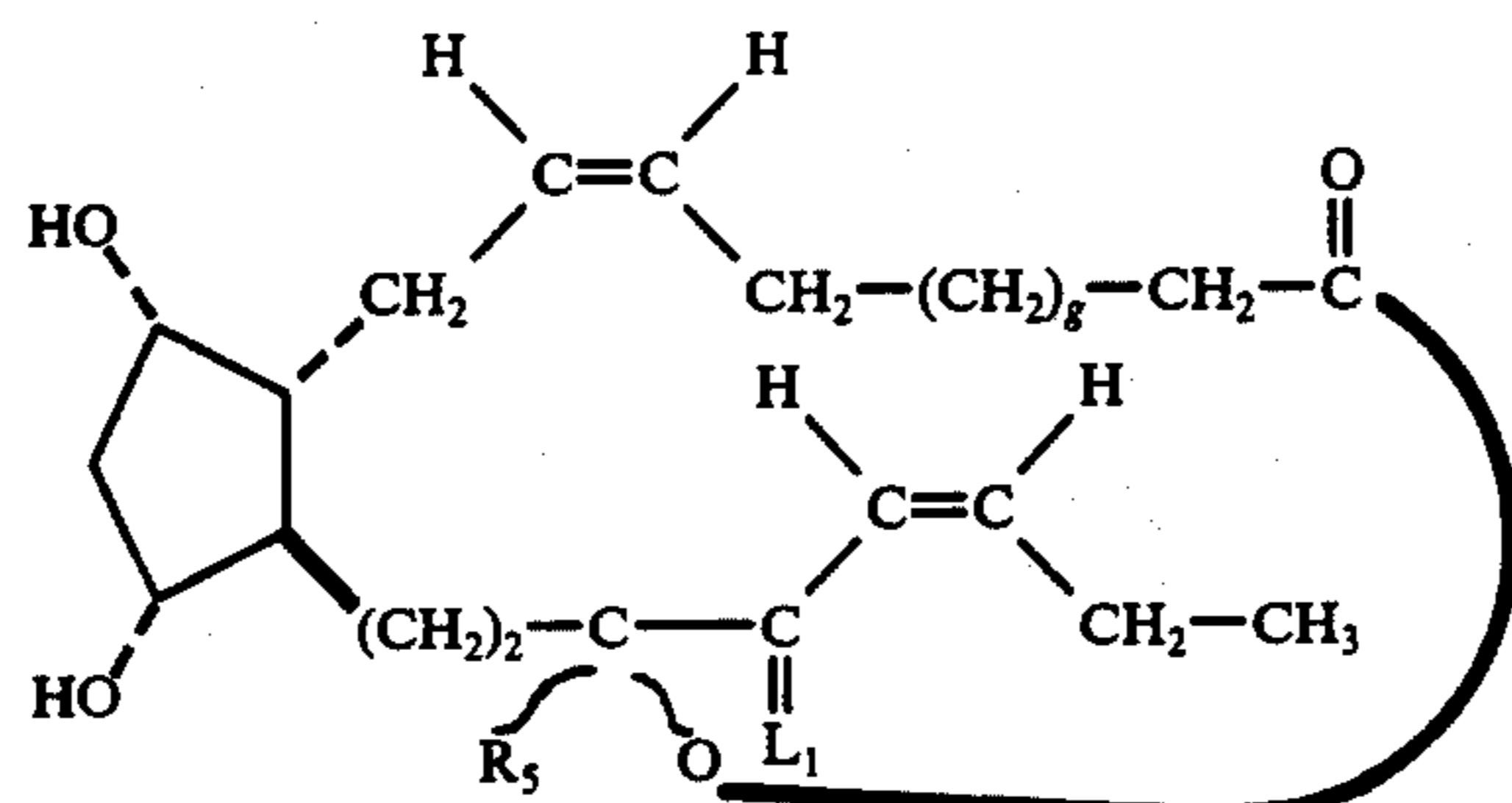
13,14-dihydro-PGF 3 \alpha -type, 1,15-lactones
