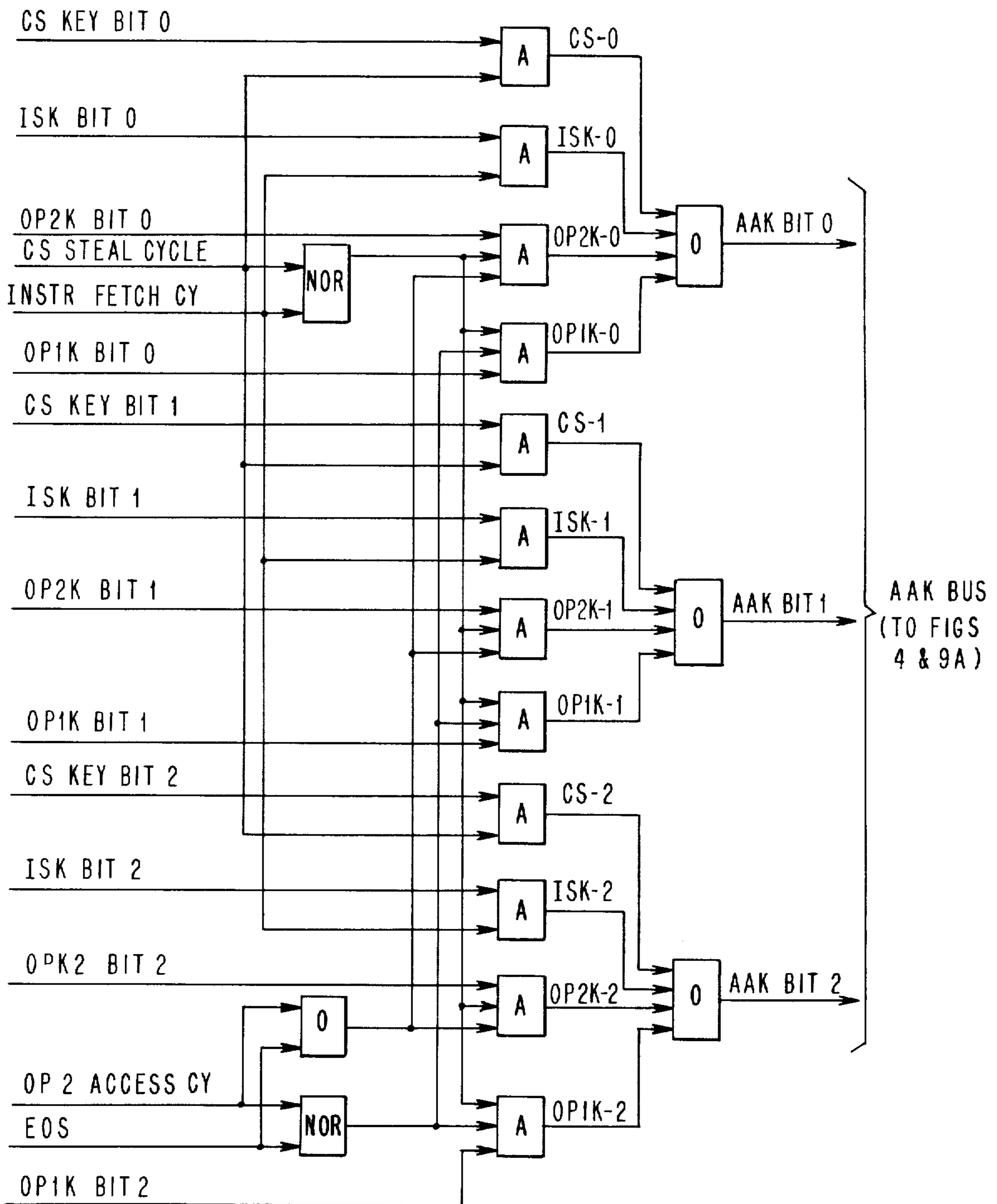
FIG. 3D (AAK SEL CIRCUITS 333)
