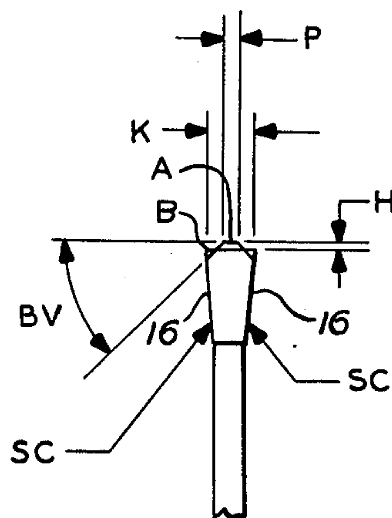
FIG. 3C
