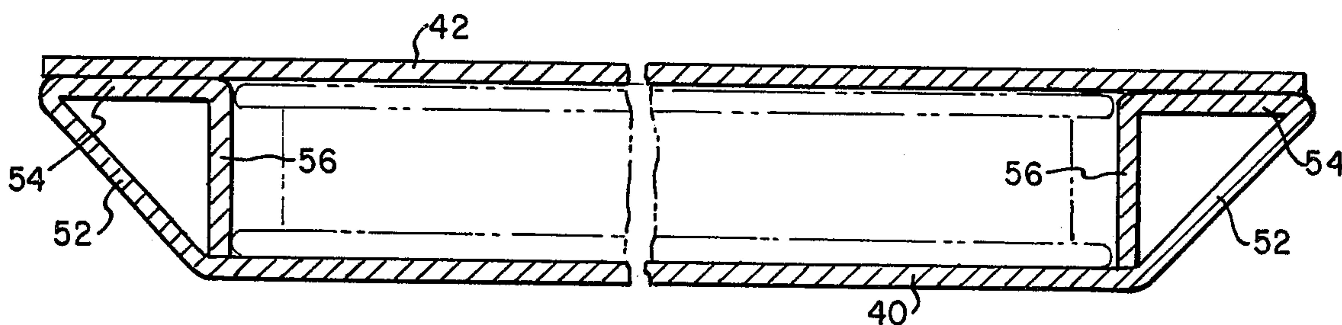
FIG. 10
