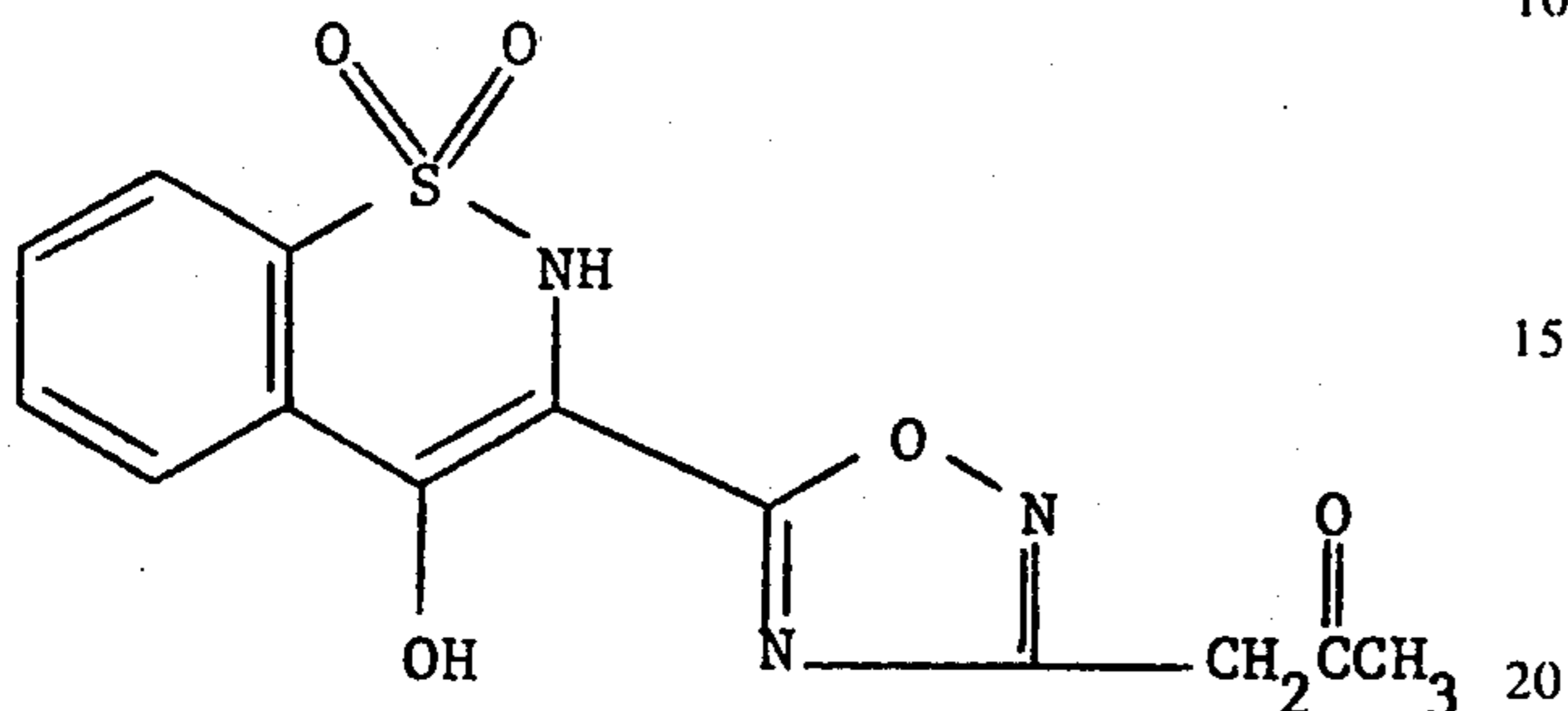
(V)
