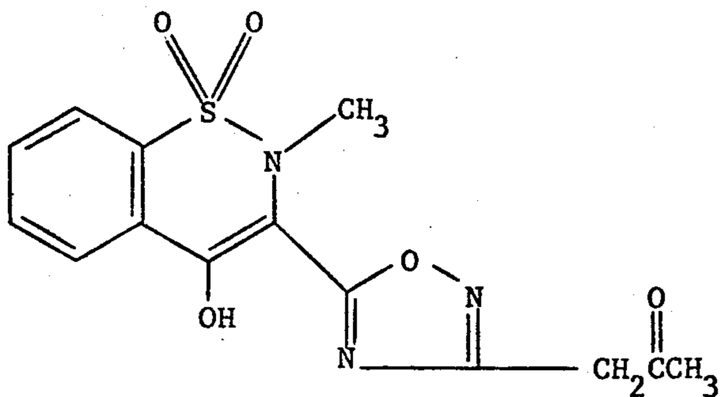
(VI)
