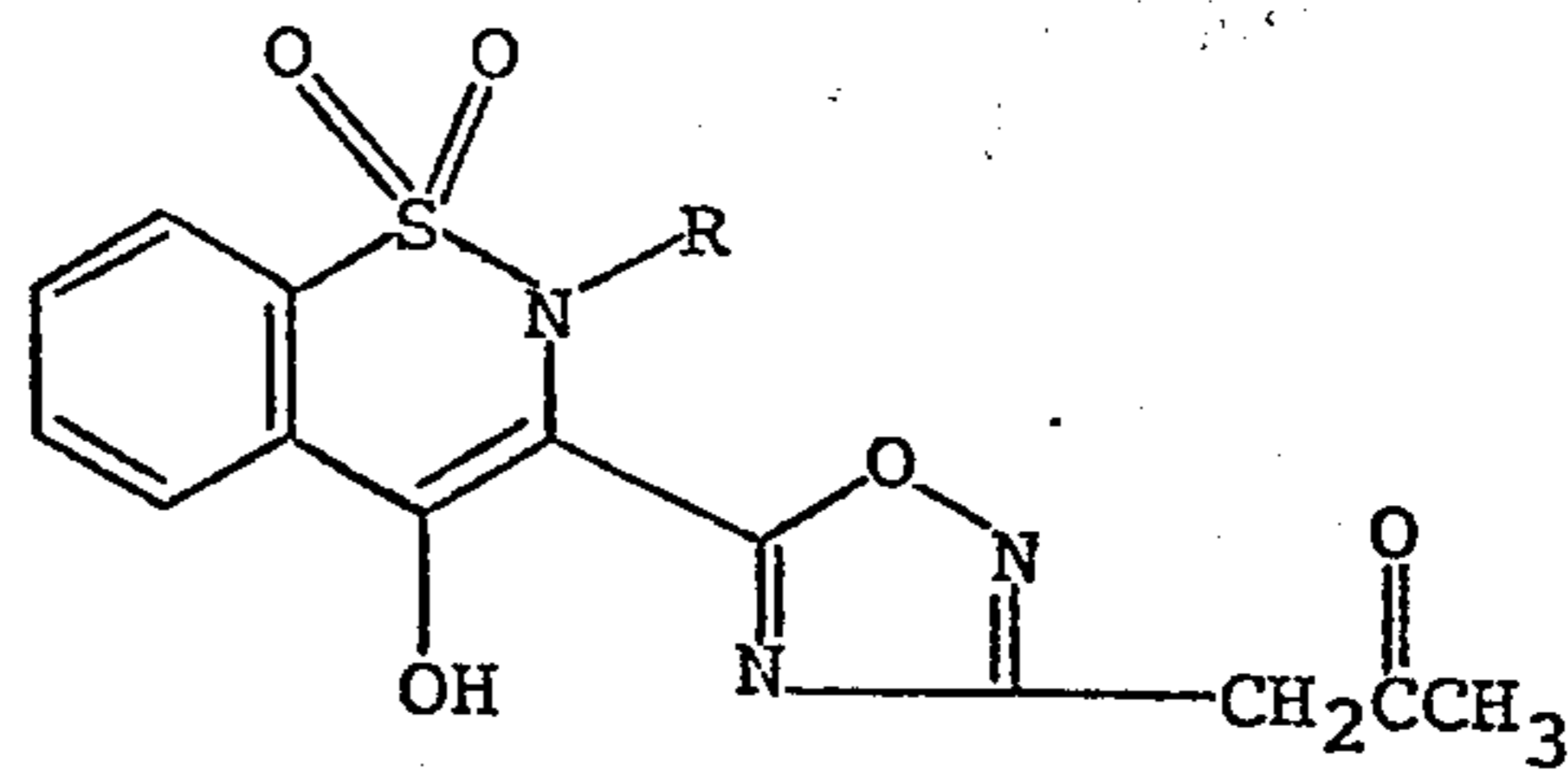
(VII)
