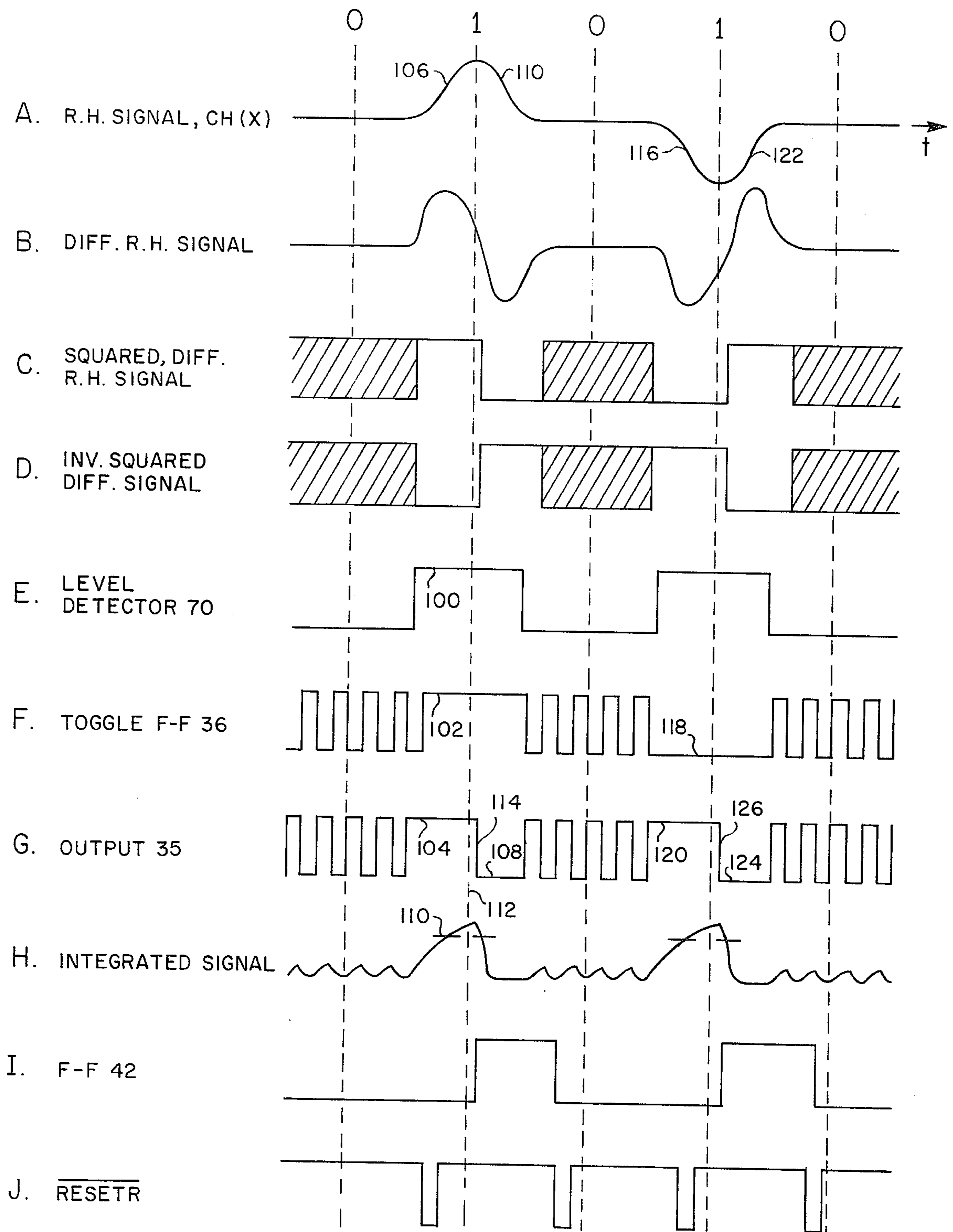
800 BPI NRZI
