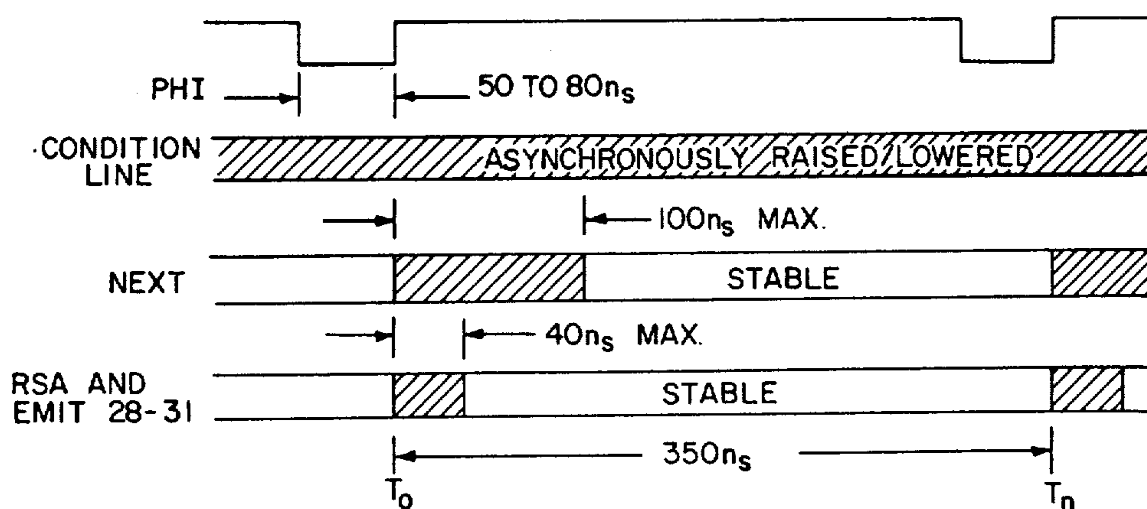
FIG. 25
