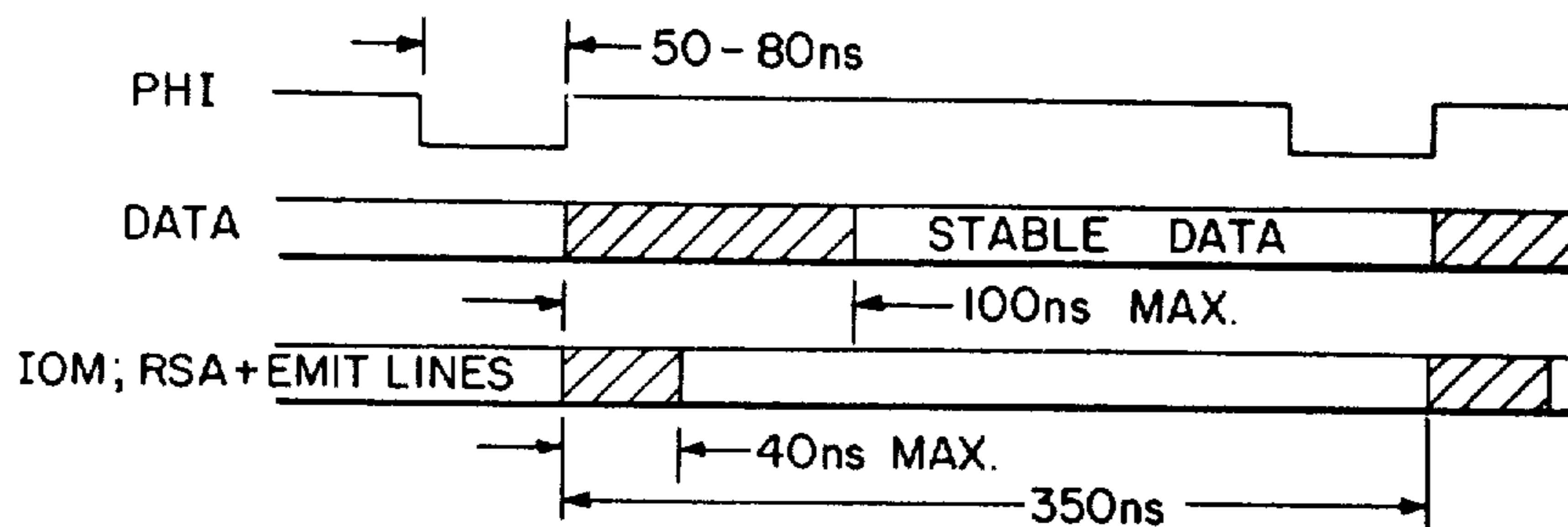
FIG. 18
