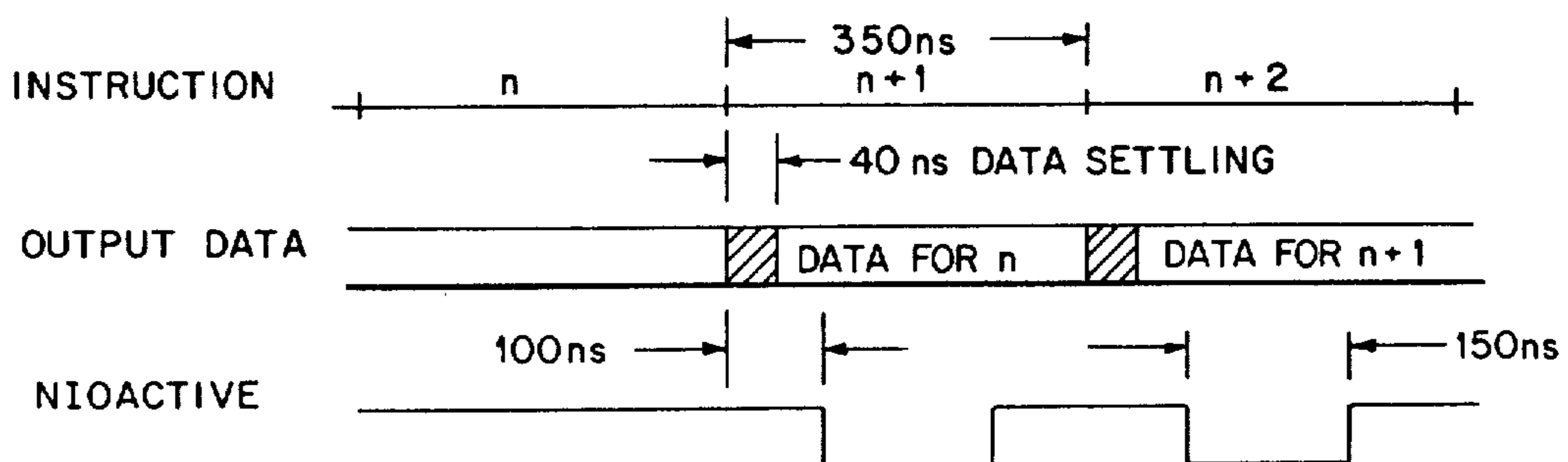
FIG. 37
