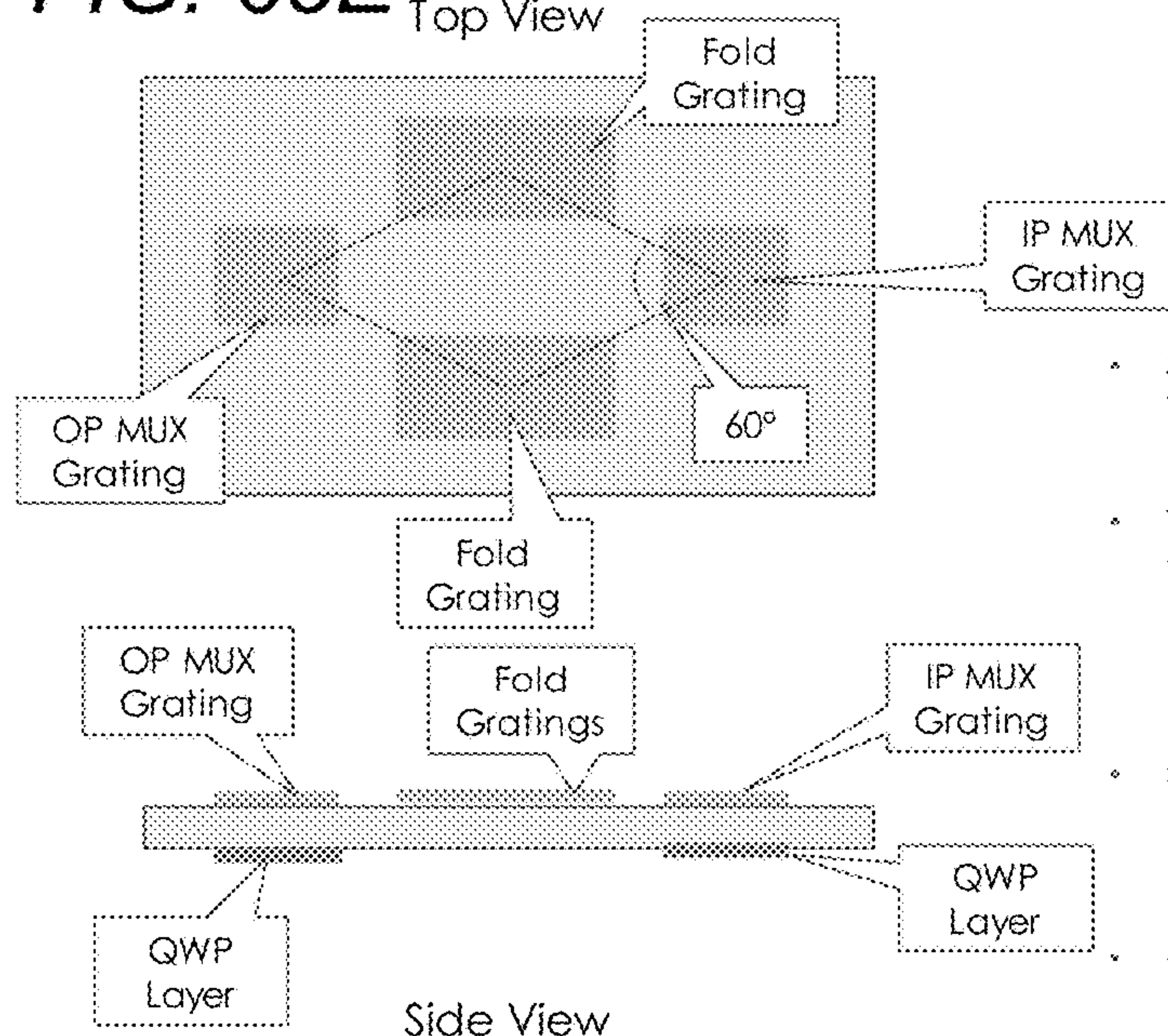
FIG. 65E Top View
