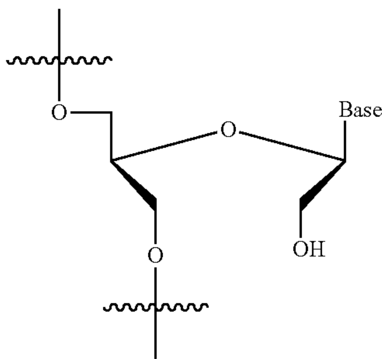
UNA
