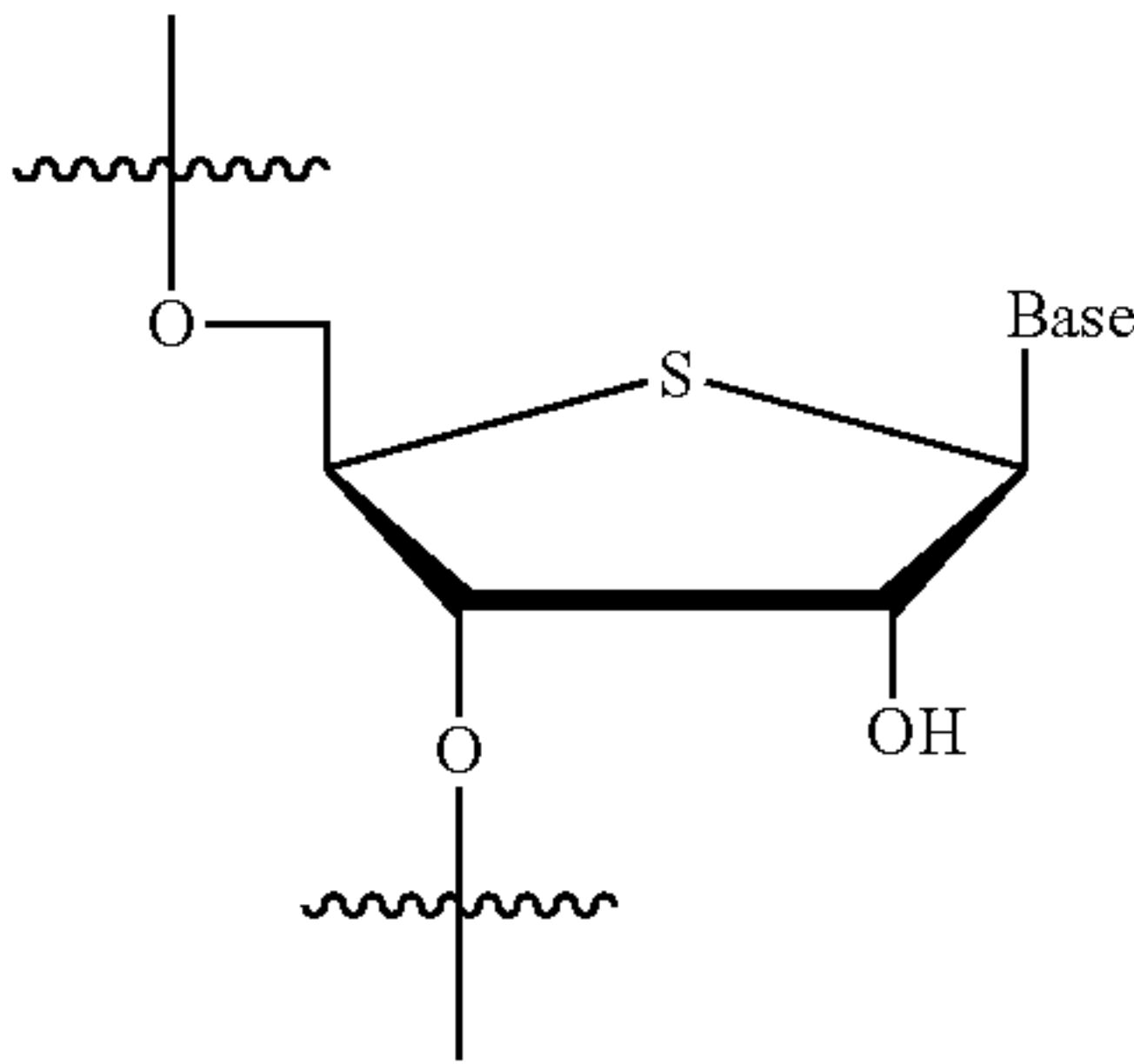
4'-S
