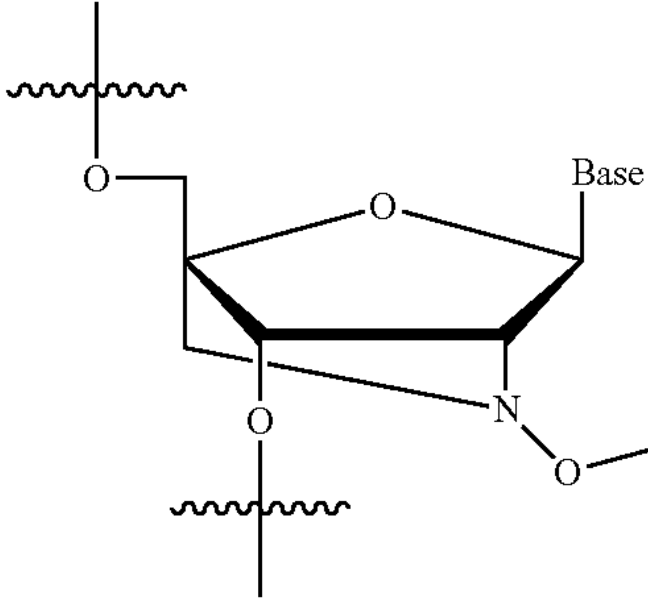
N-MeO-amino BNA
