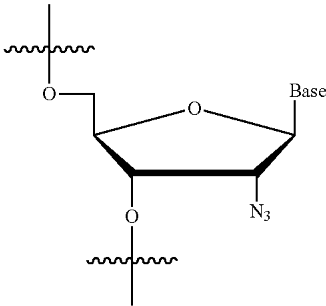
2'-azido
