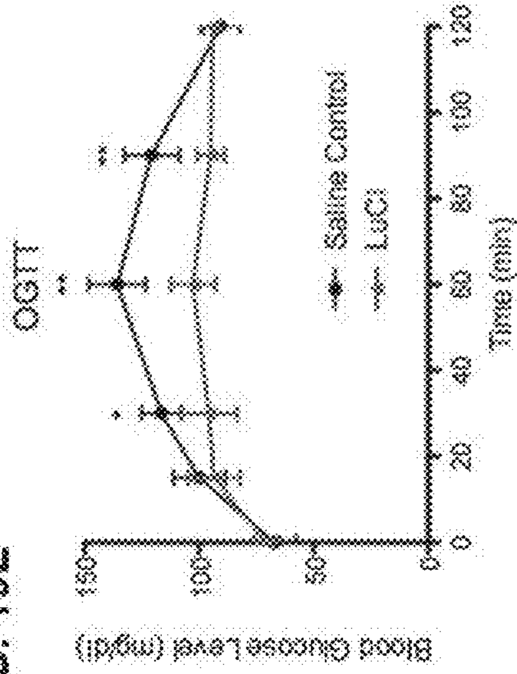
FIG. 19F
