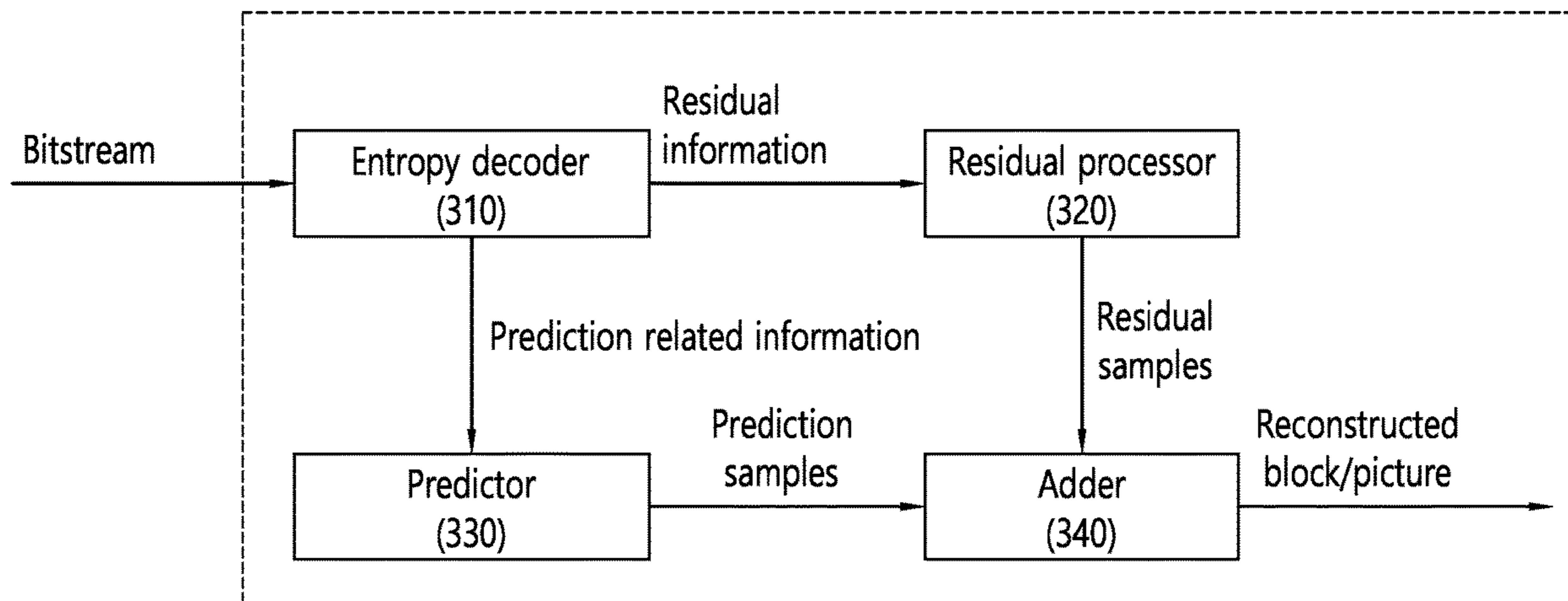
Decoding apparatus (300)
