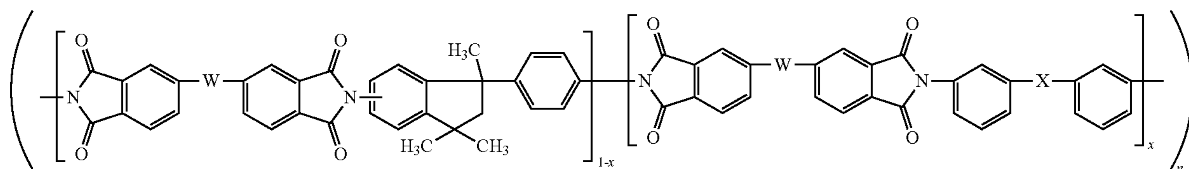
Structure Xa
