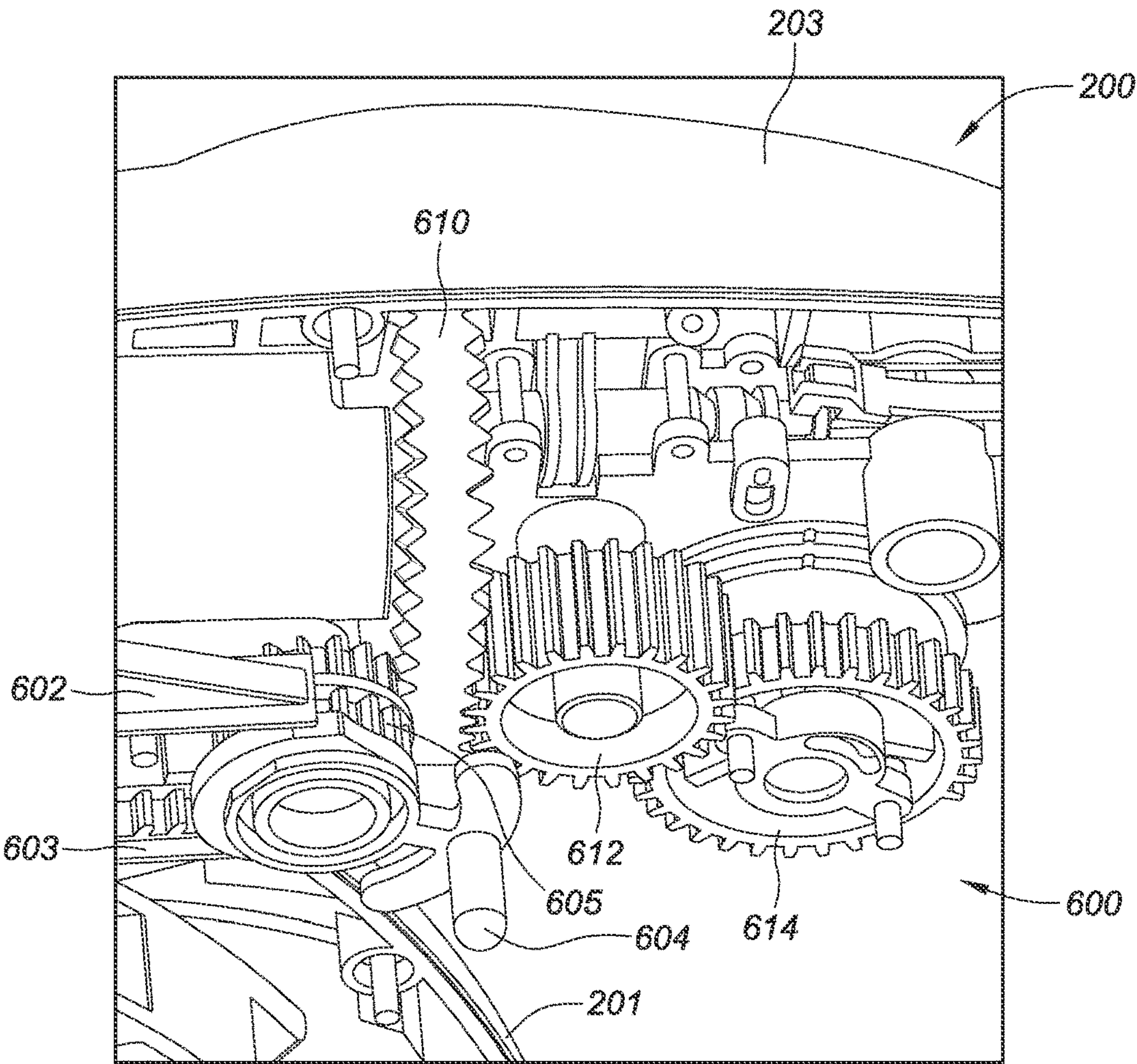
FIG. 6B
