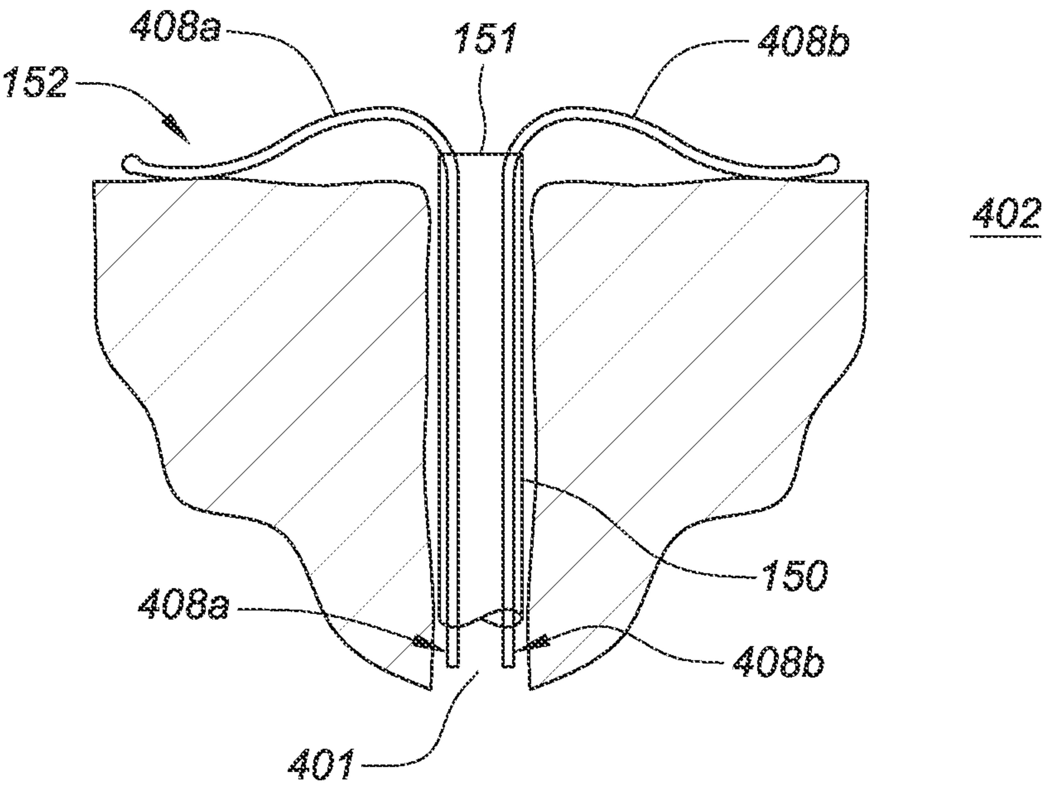
FIG. 4B
