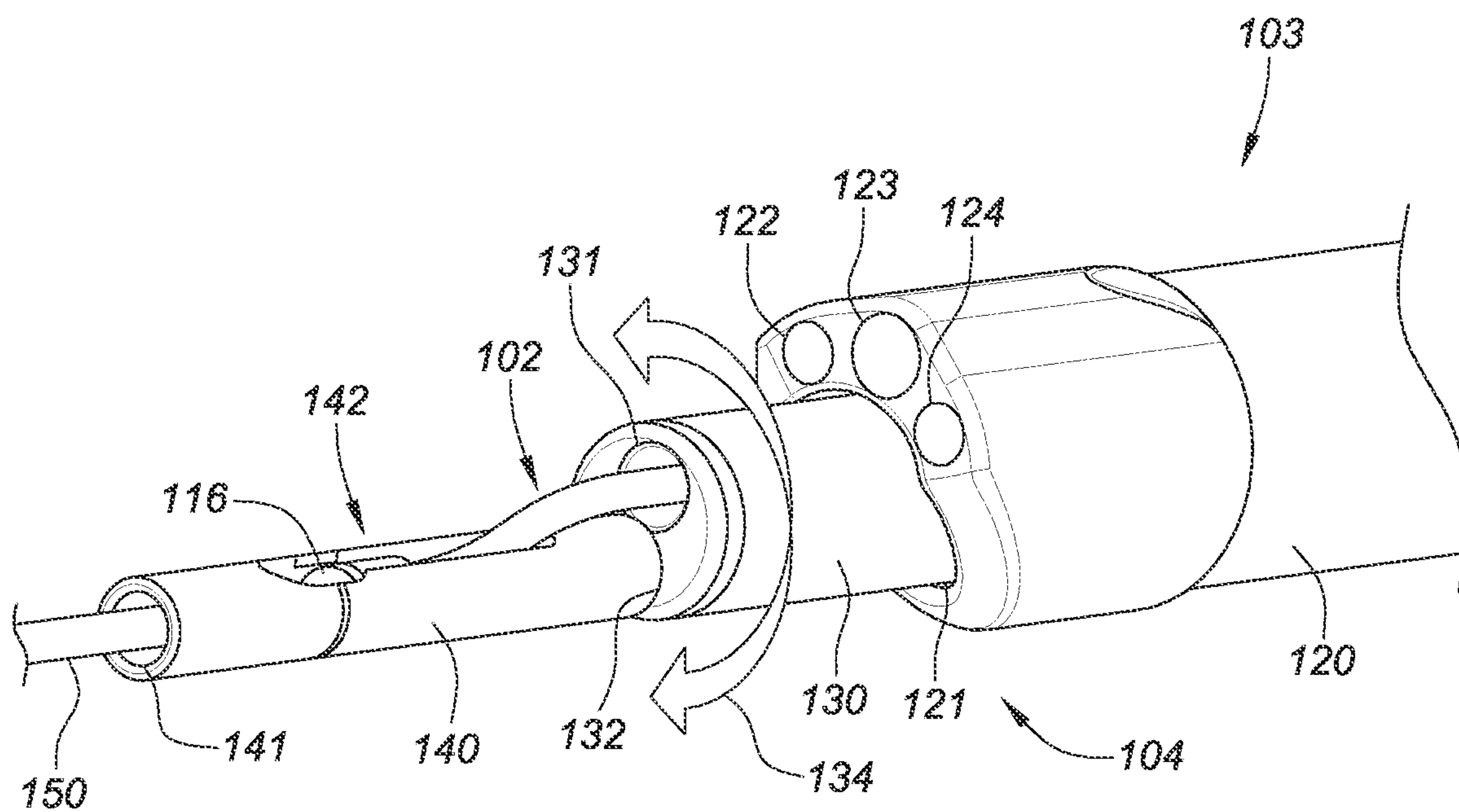
FIG. 2A
