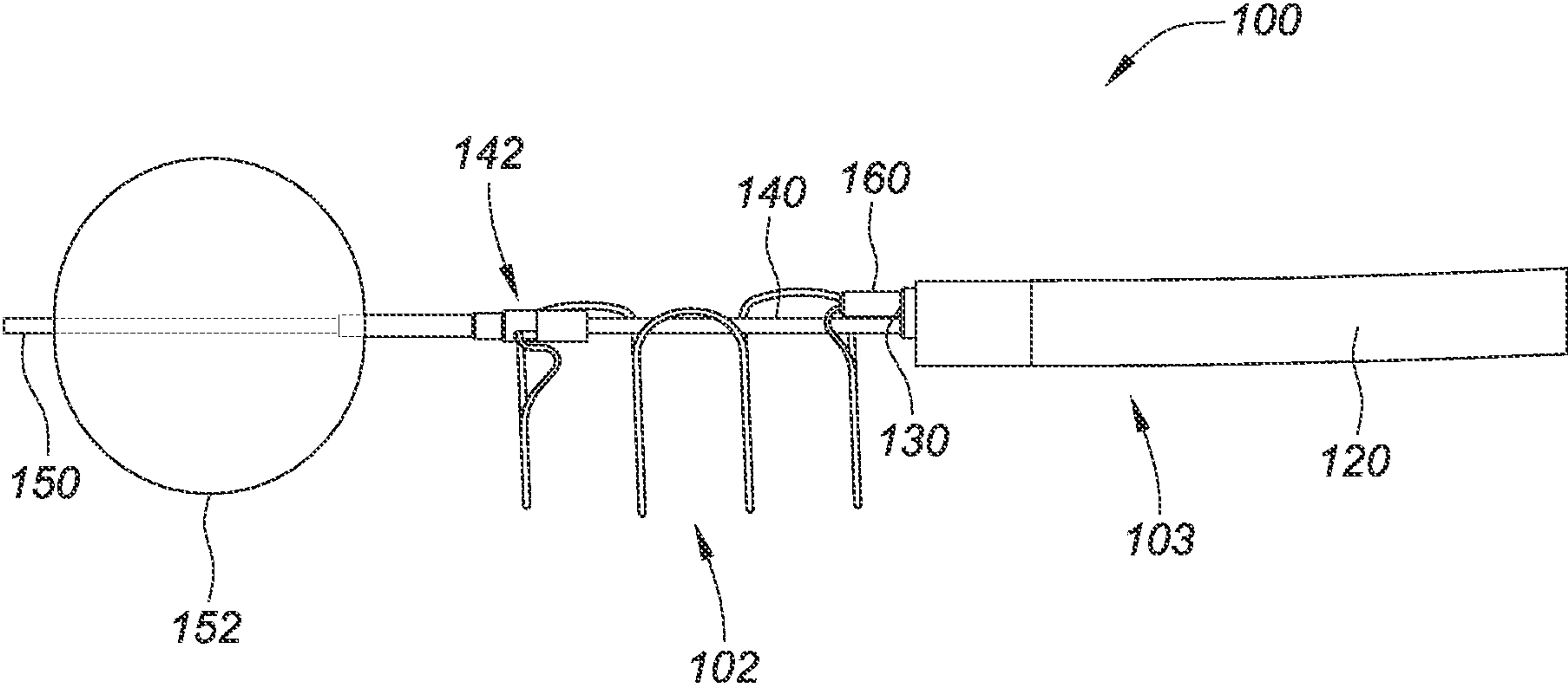
FIG. 2G
