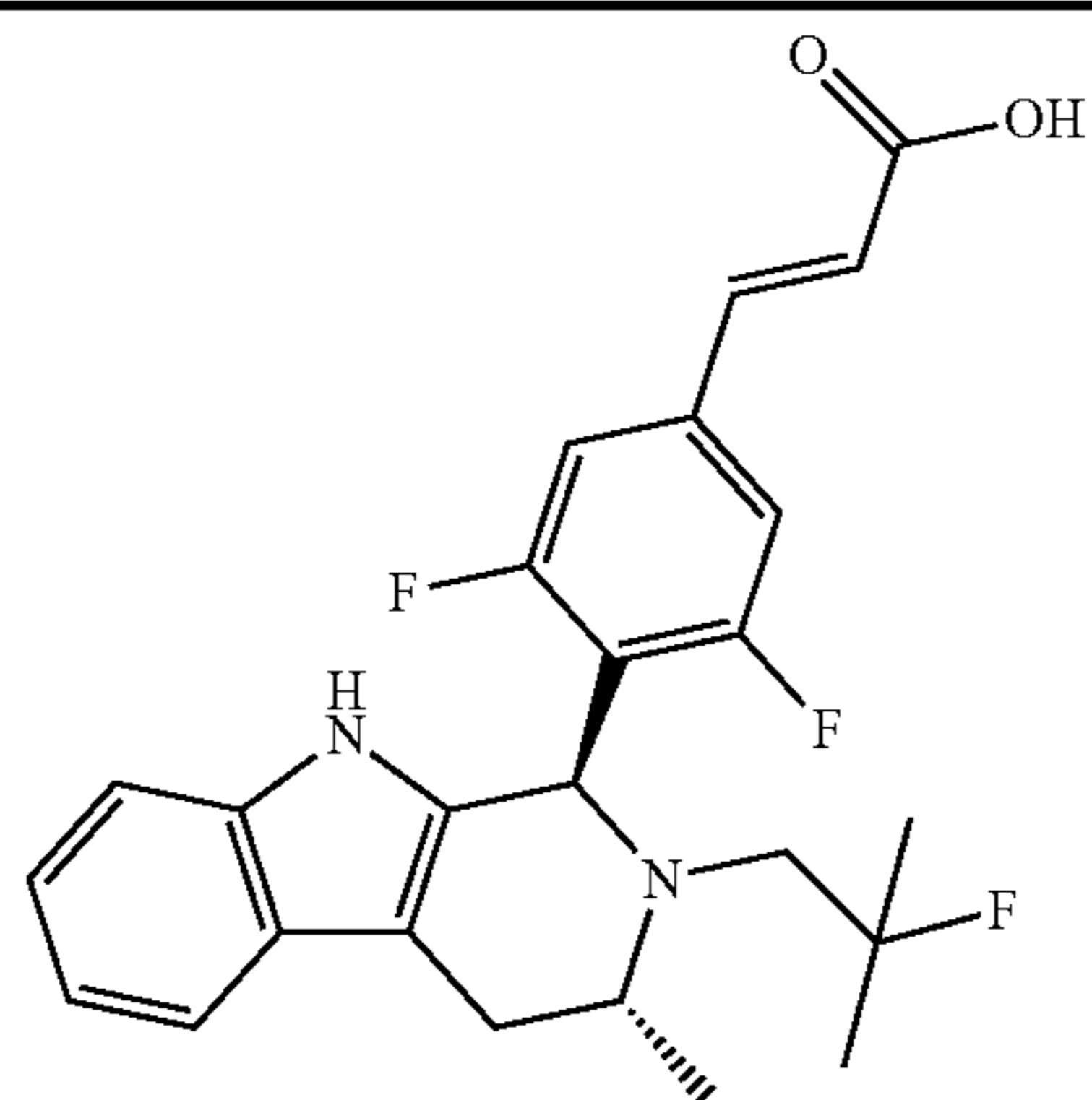
WO 2014/191726 Example 1 (AZD9496)
