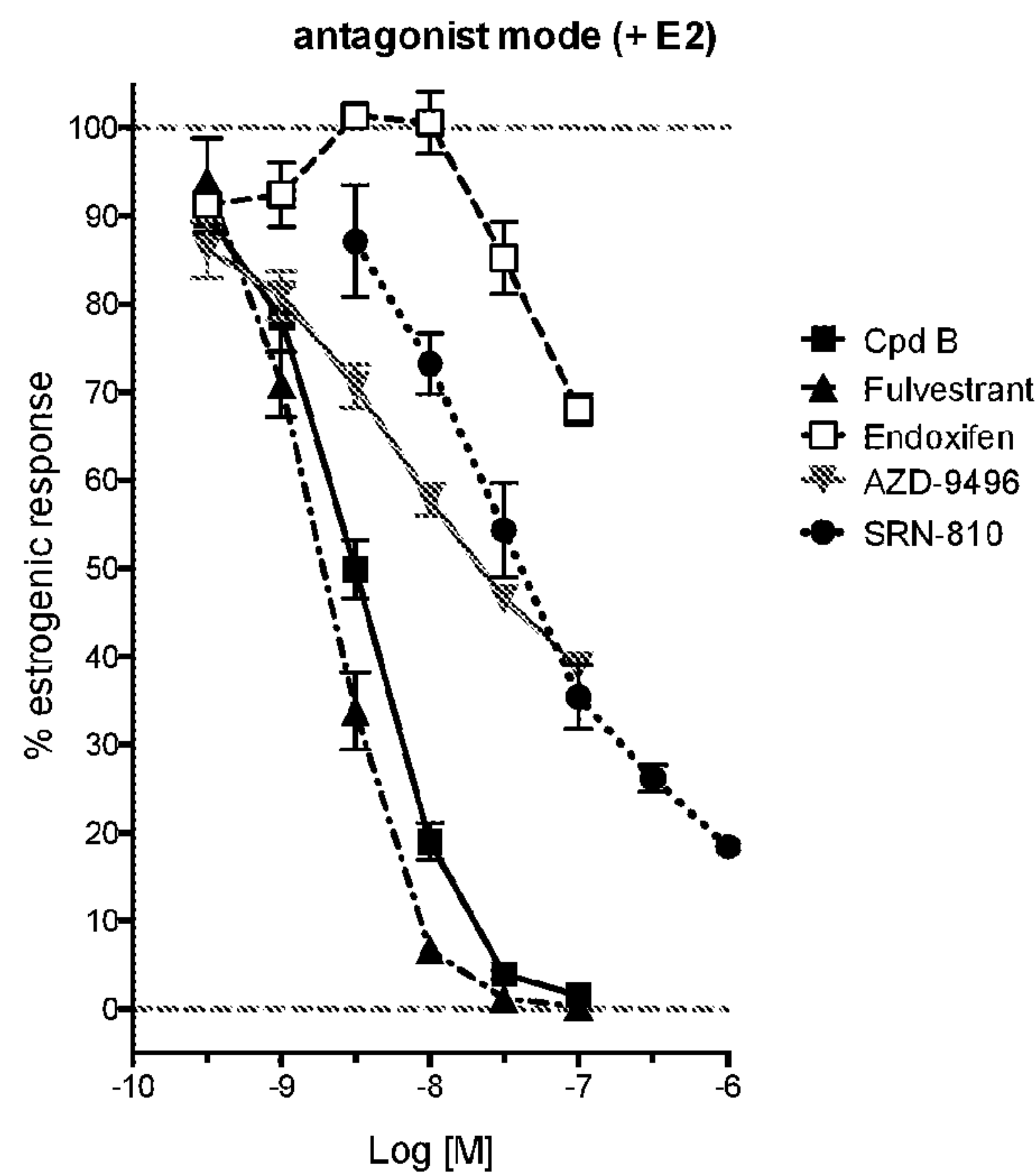
FIG. 6B
