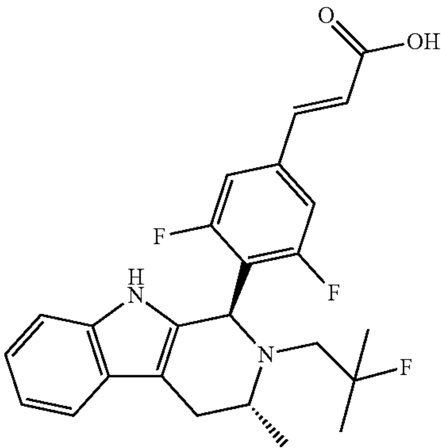
WO 2014/191726 Example 1 (AZD9496)
