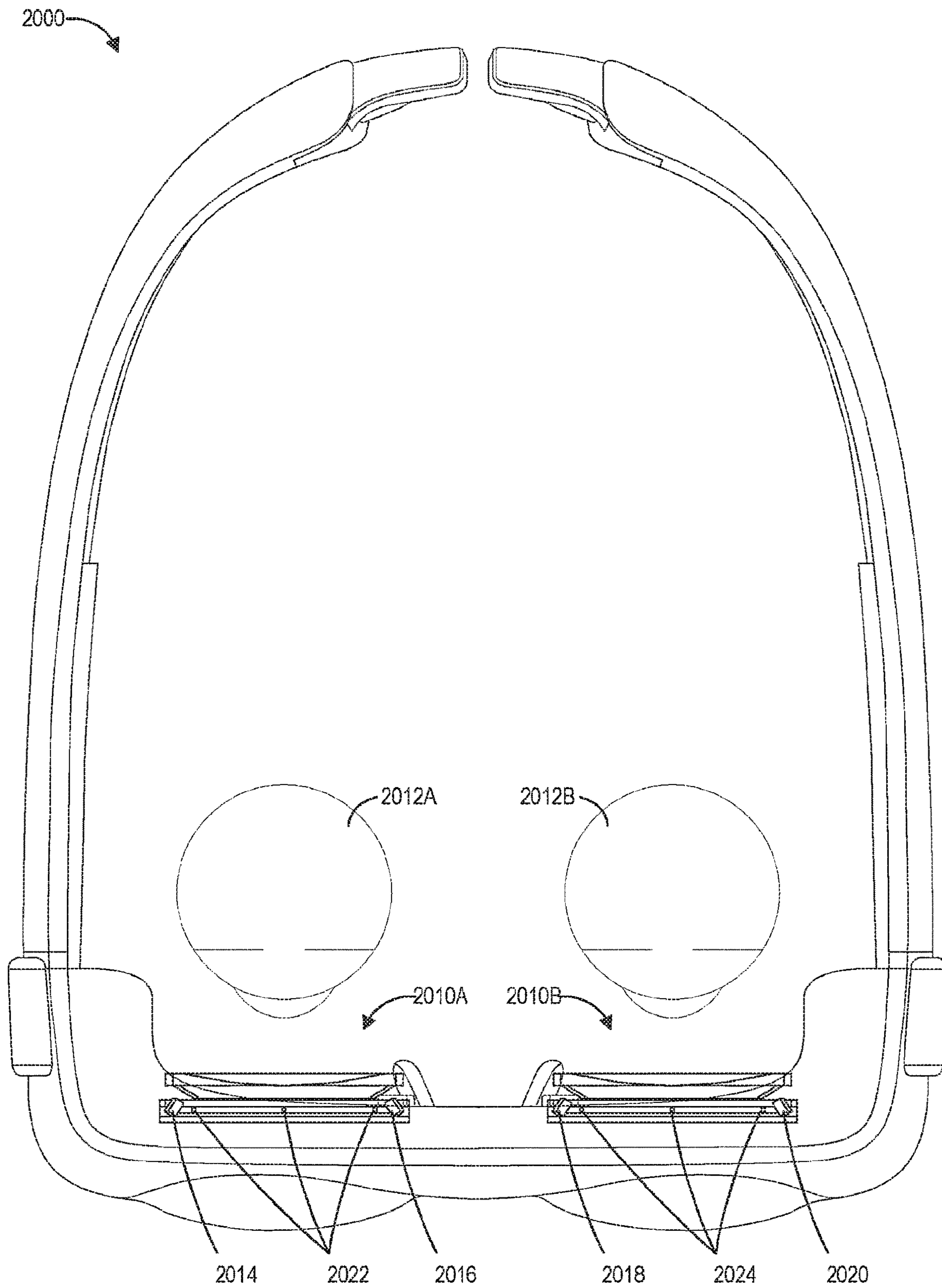
FIG. 9B
