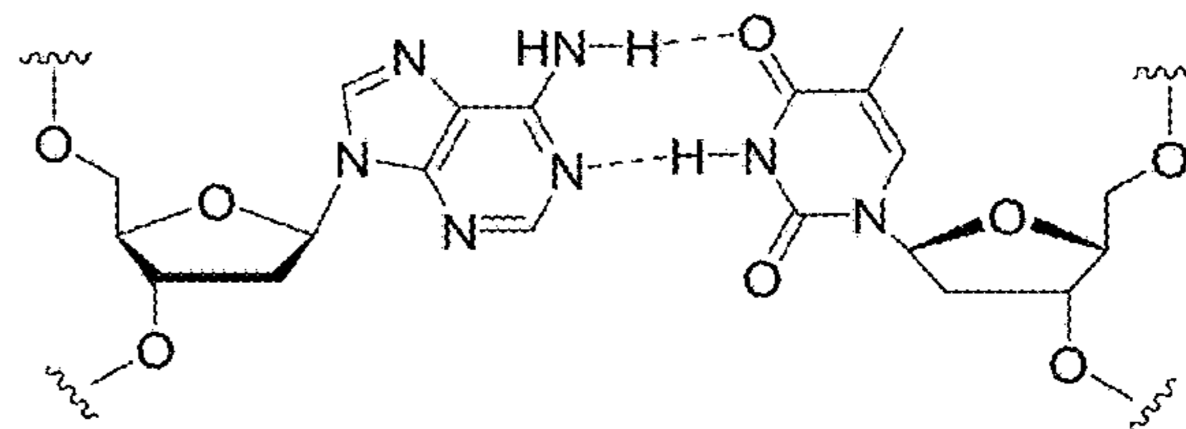
dA-dT
