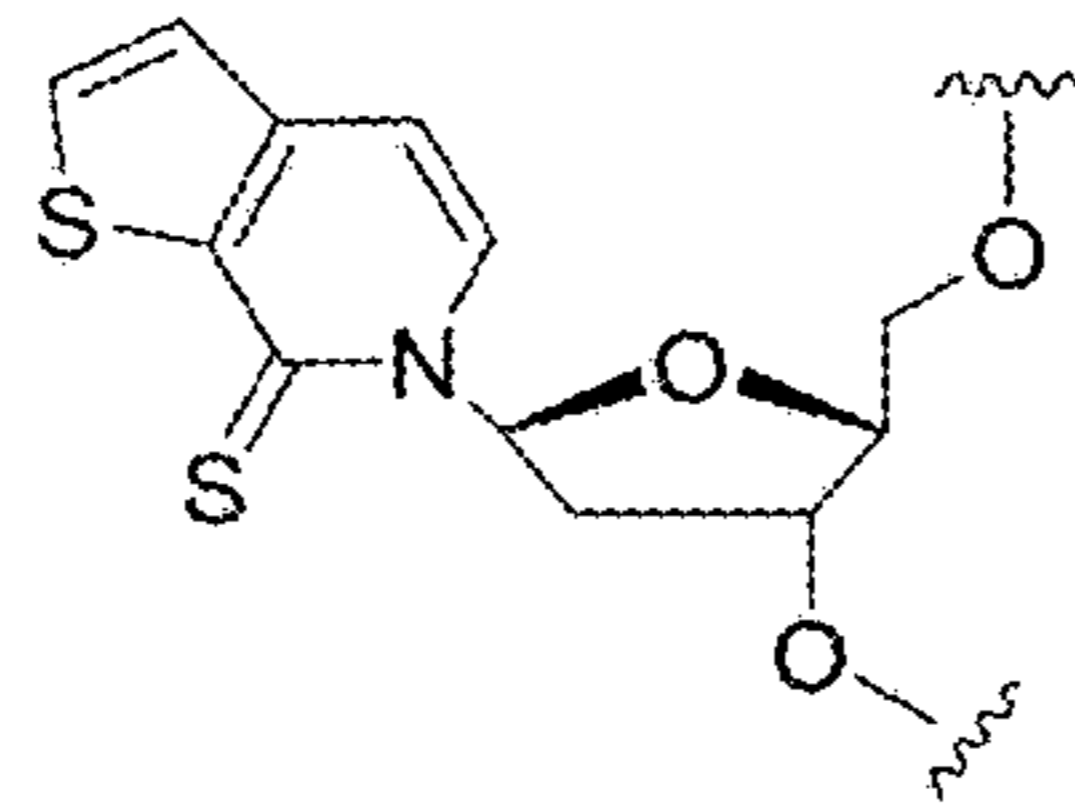
dNaM-dTPT3
