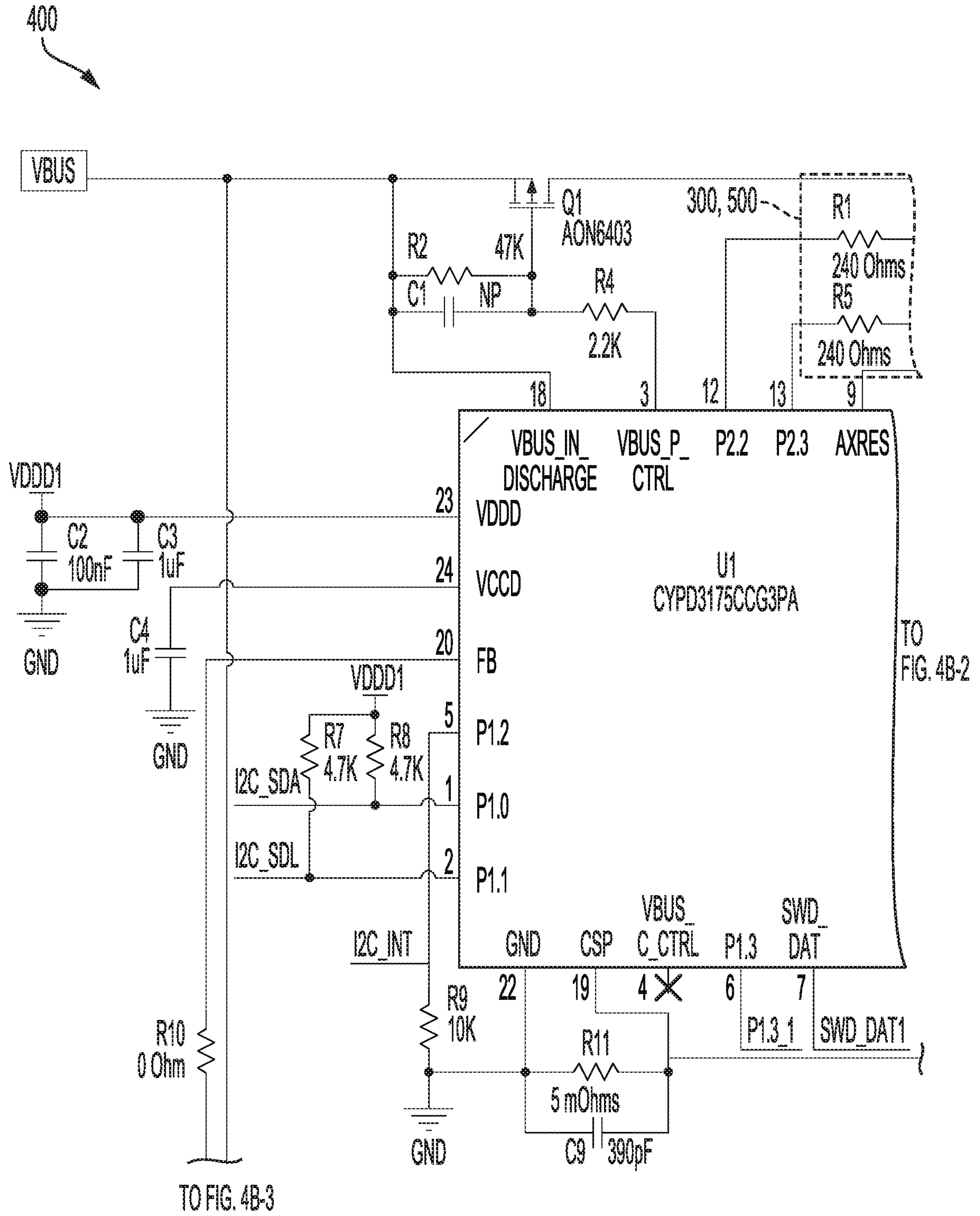
FIG. 4B-1
