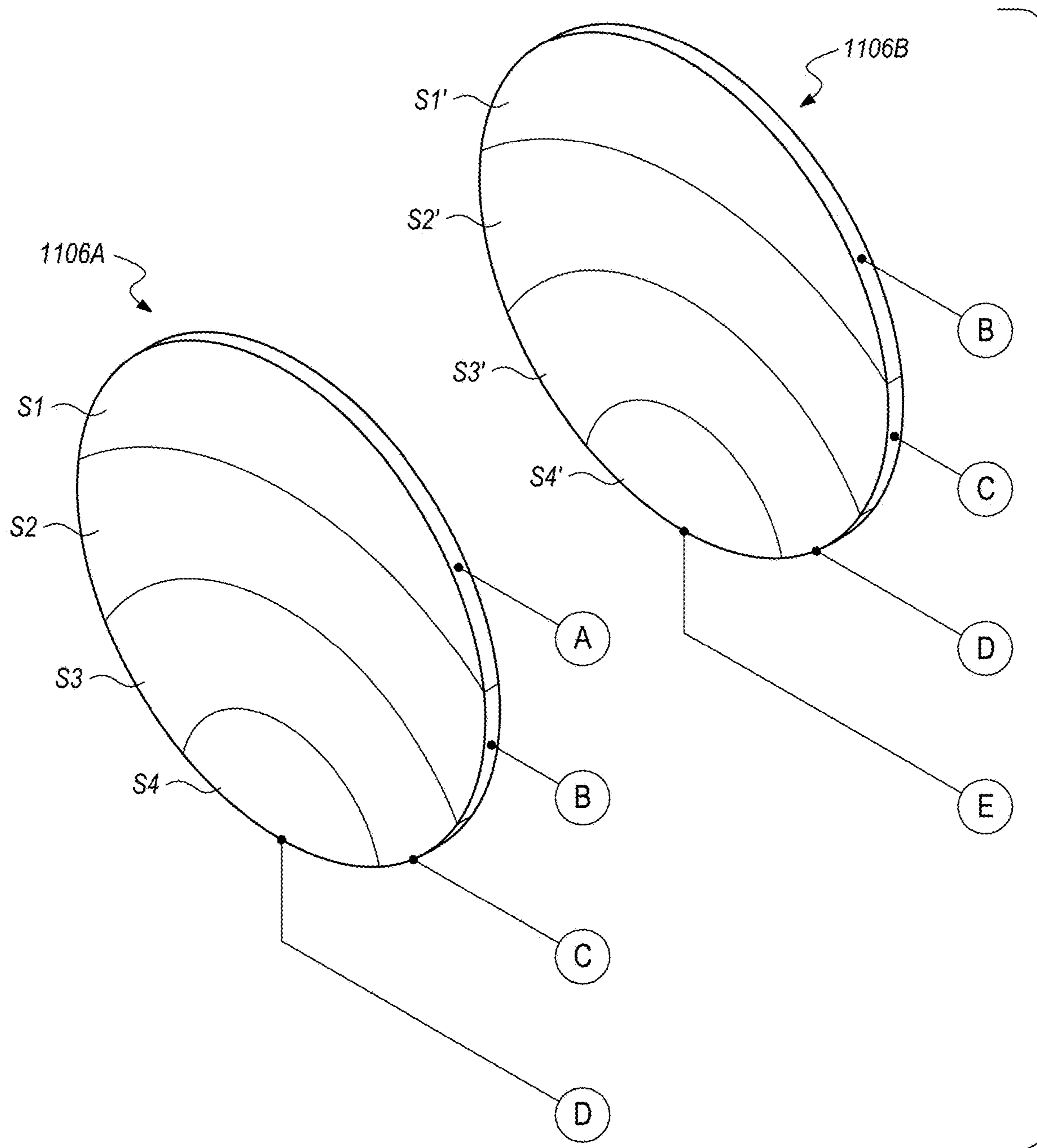
FIG. 17A
