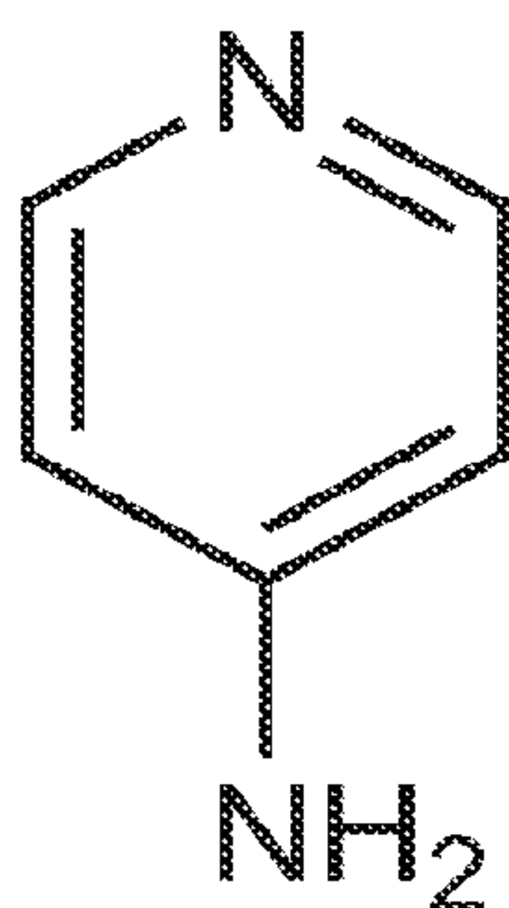
4-aminopyridine
