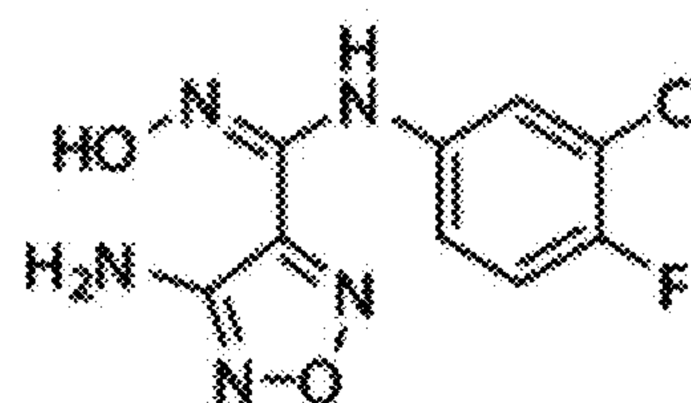
INCB024360 (Epacadostat)
