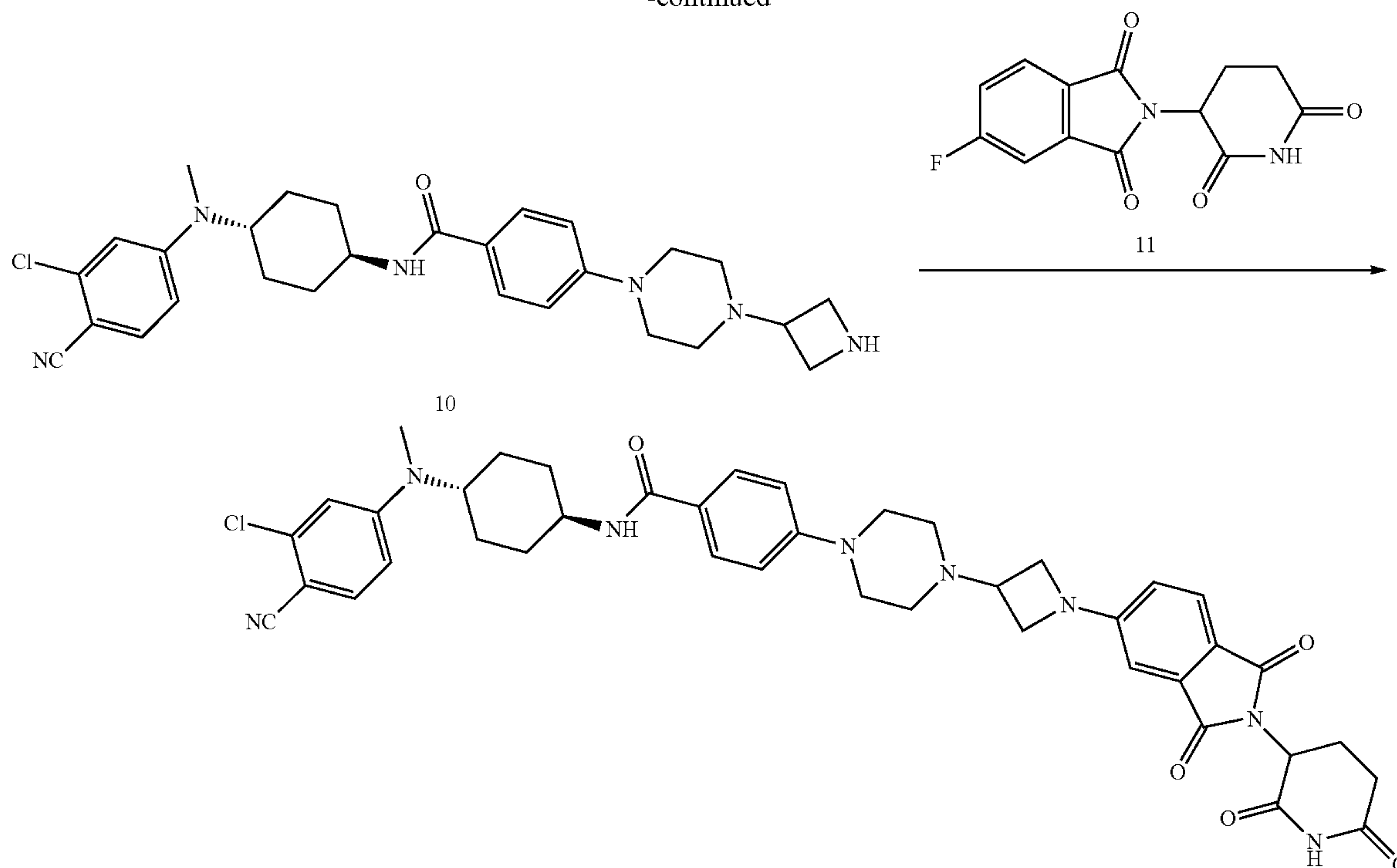
Cpd. No. 31
