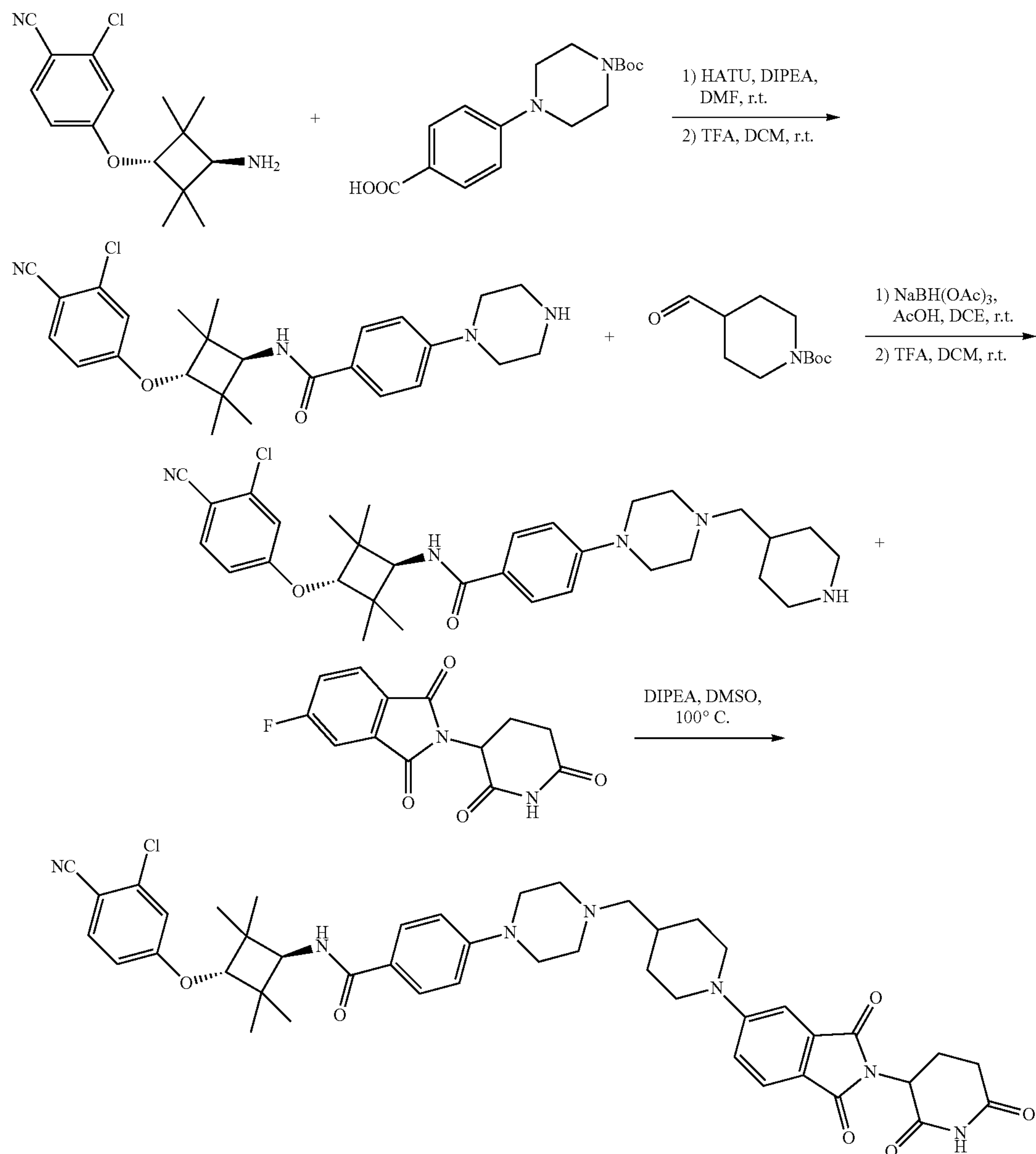
Cpd. No. 46
