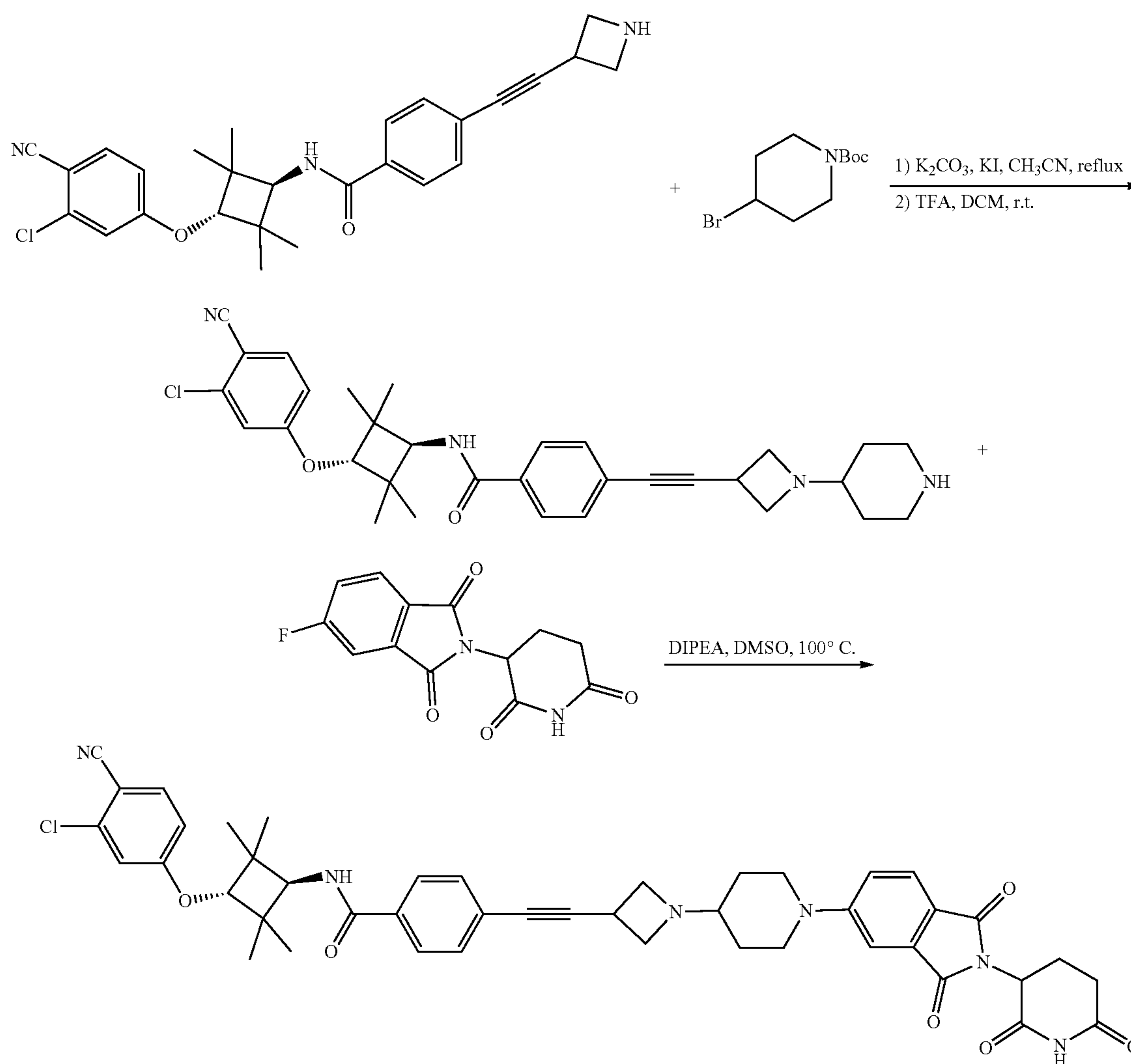
Cpd. No. 111
