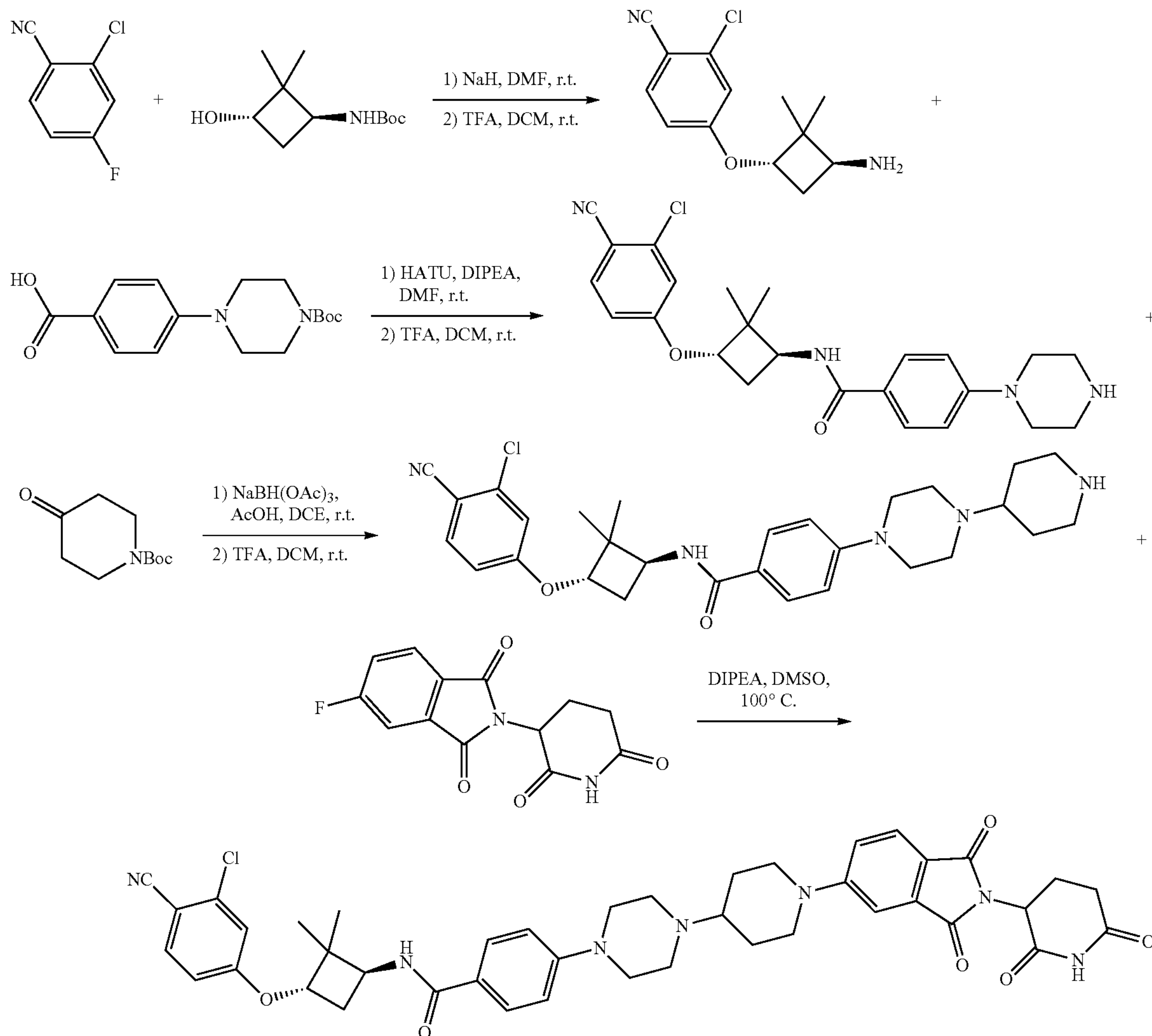
Cpd. No. 121
