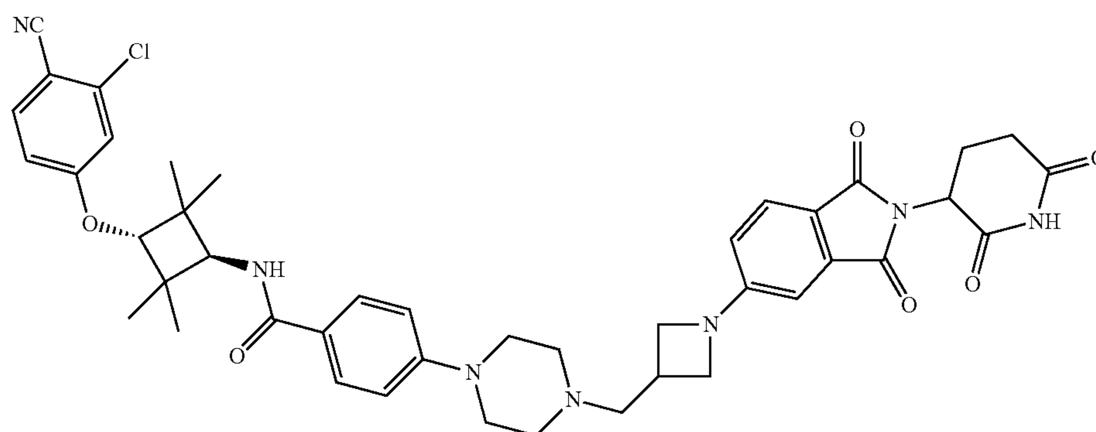
Cpd. No. 112
