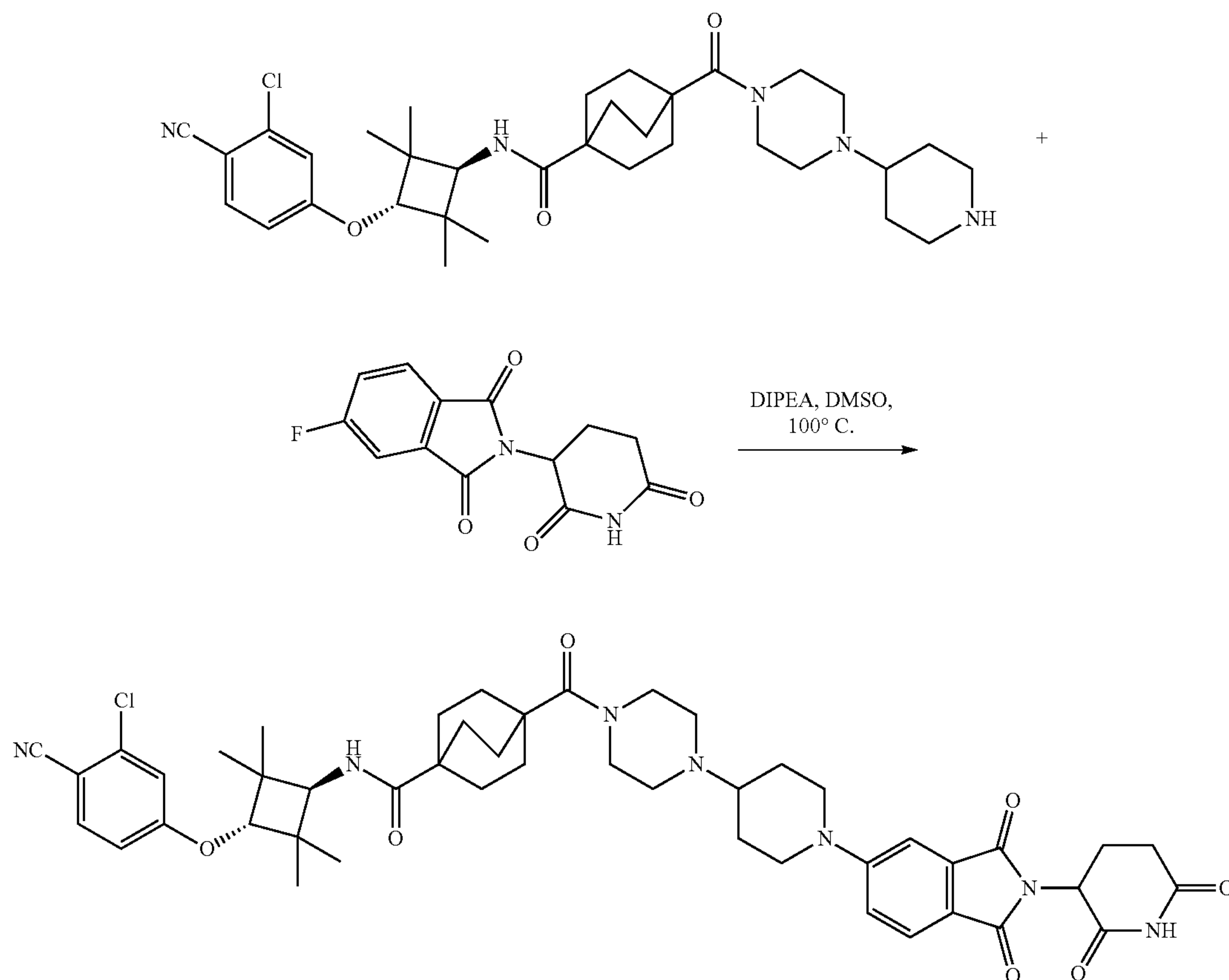
Cpd. No. 119
