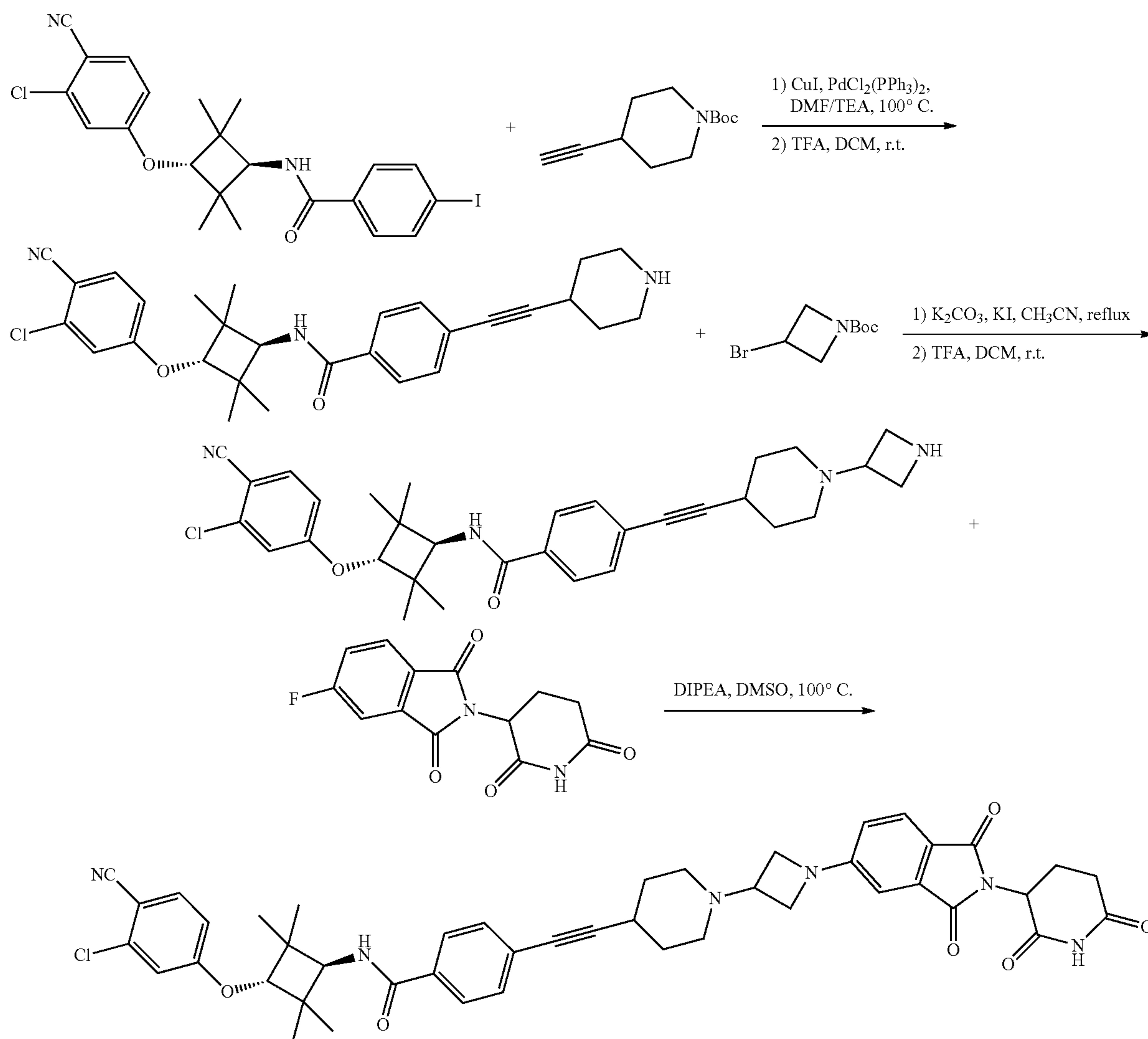
Cpd. No. 110
