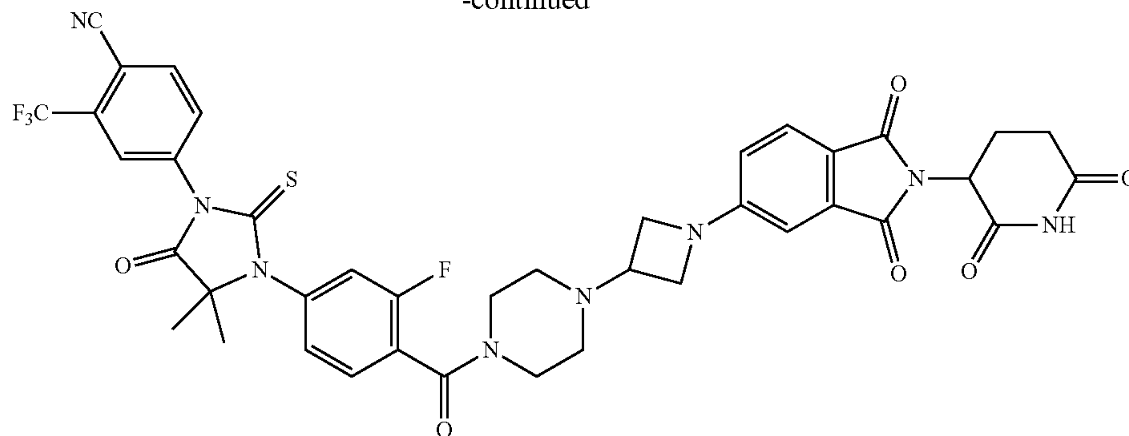
Cpd. No. 18
