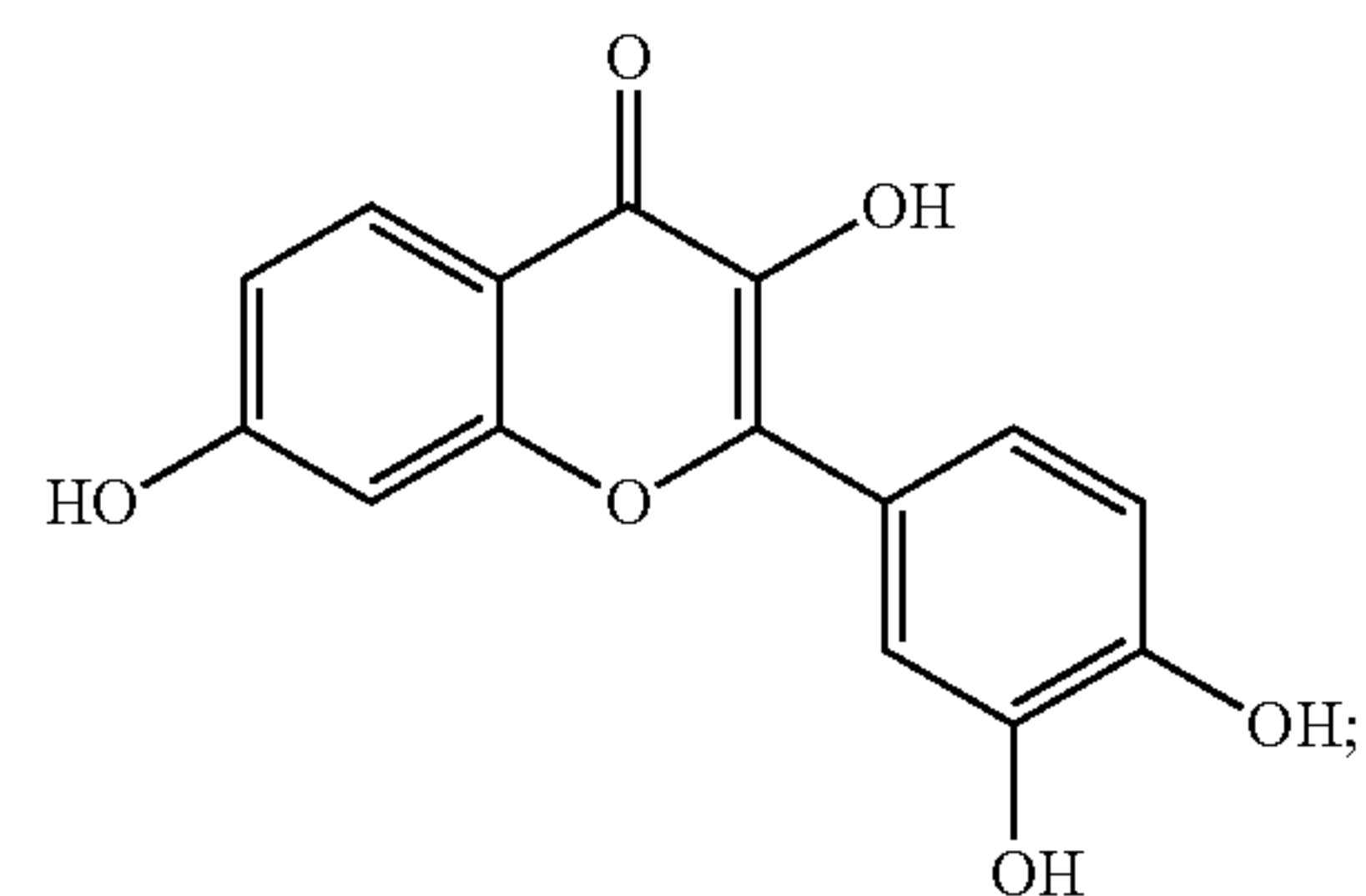
(fisetin)
