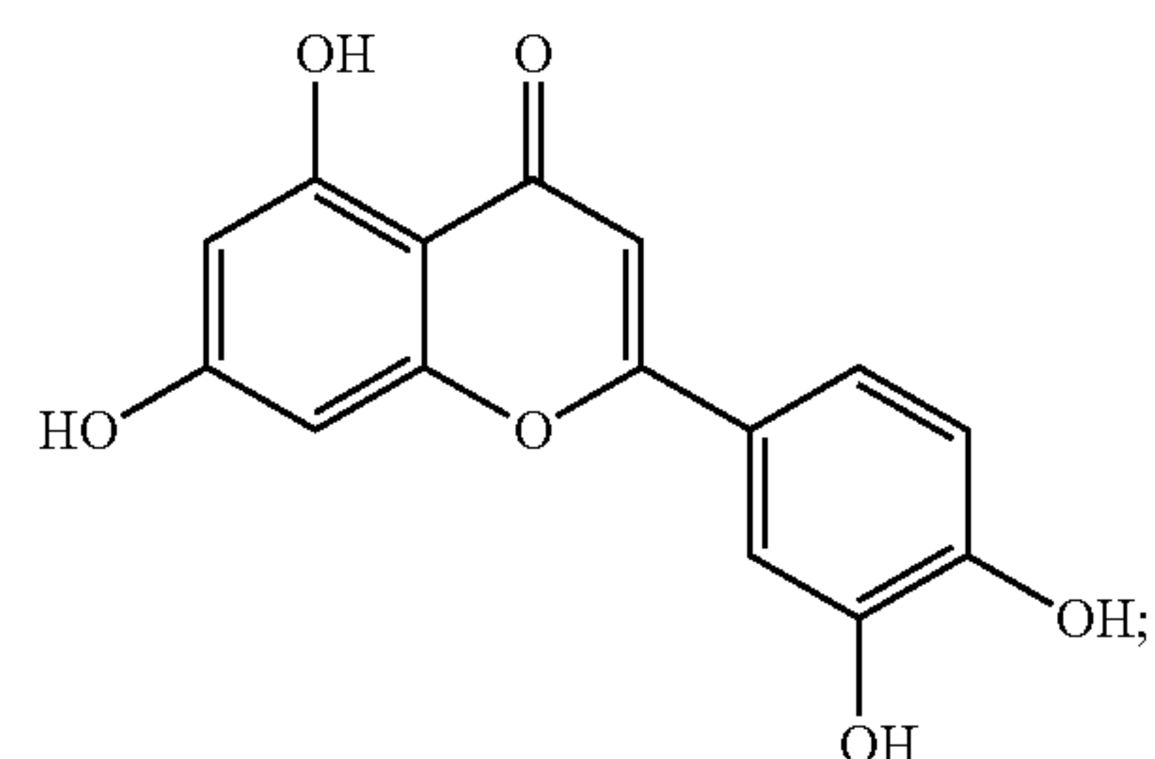
(luteolin)
