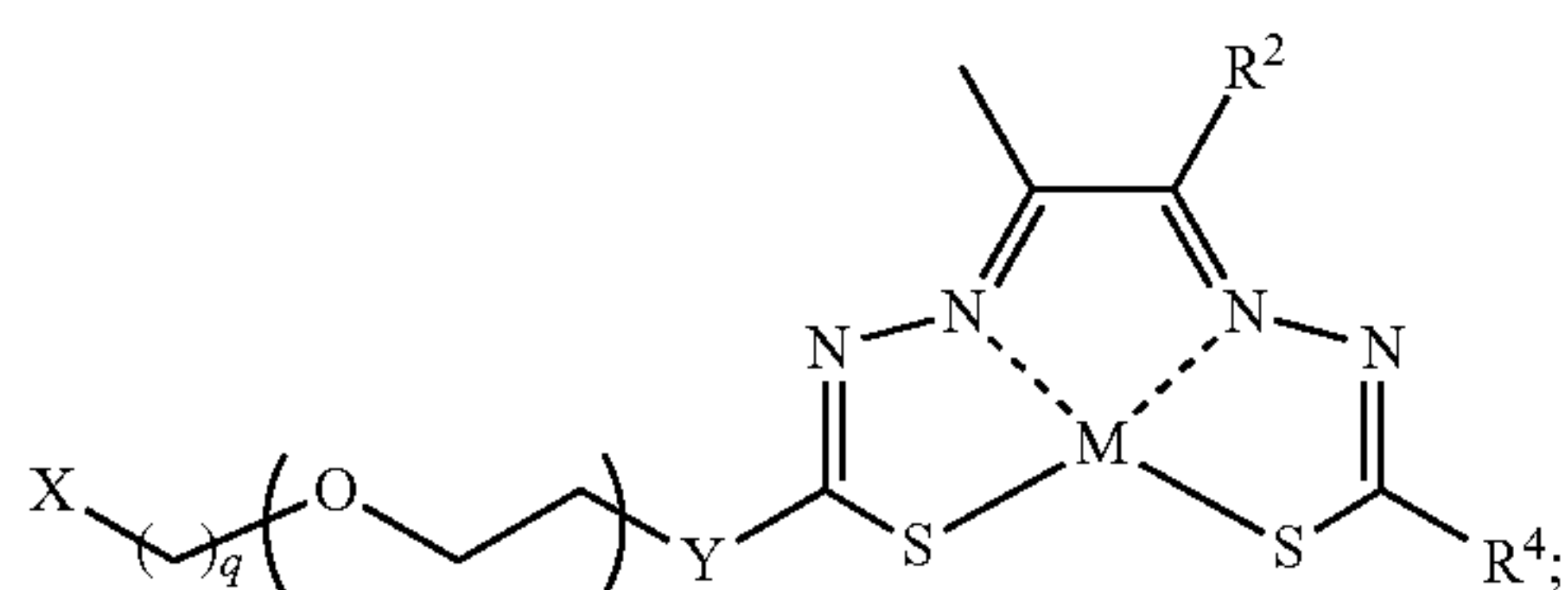
Formula IIIT'
