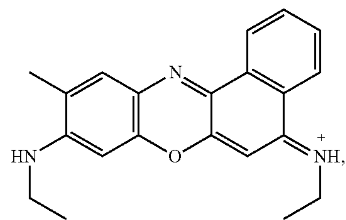
(Oxazine 720)
