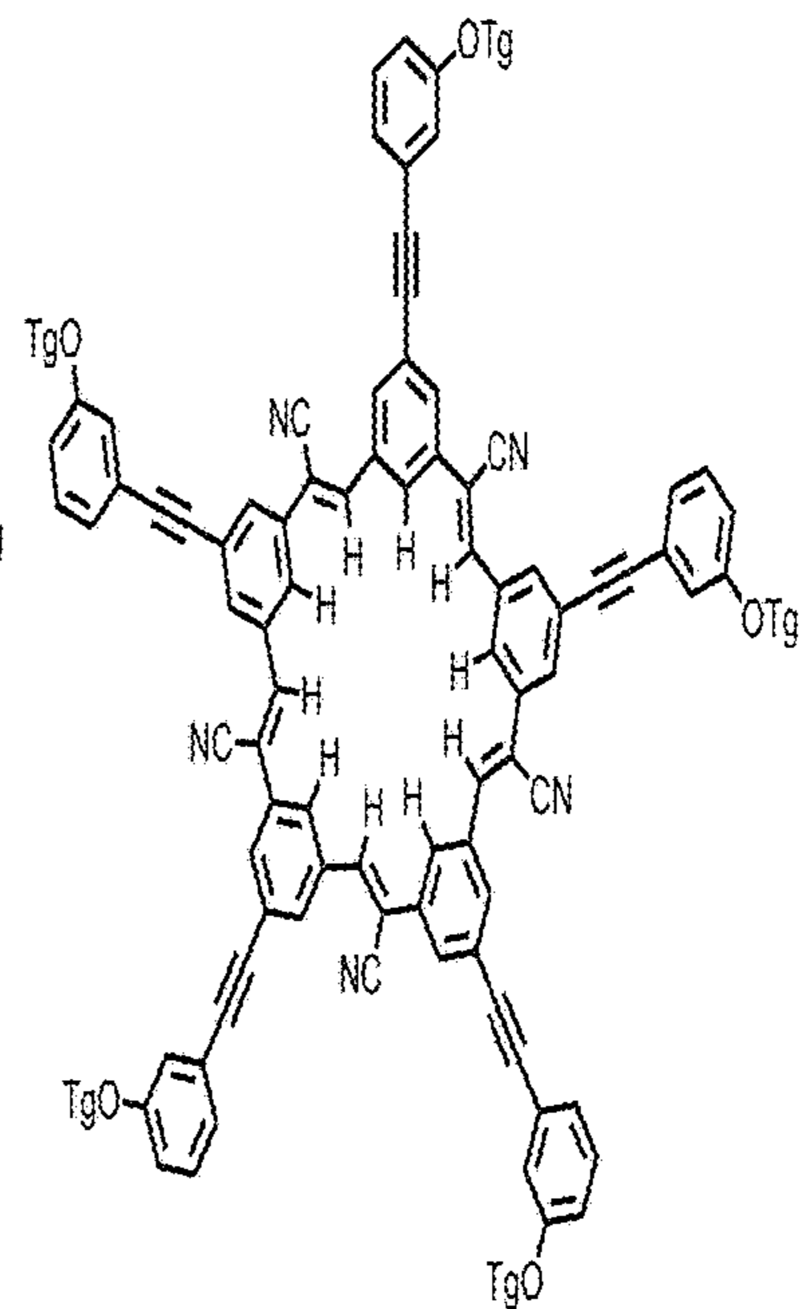
Cyanostar 4
