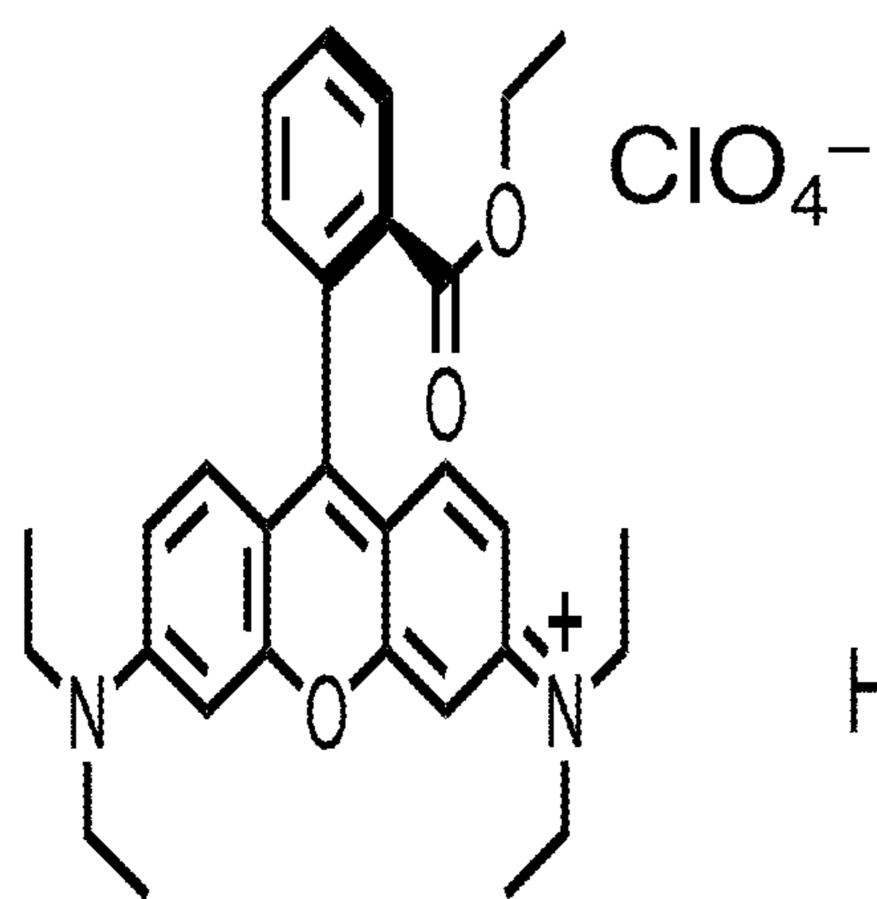
Rhodamine 3B·ClO 4
