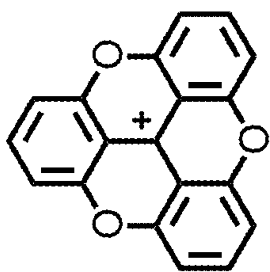
TOTA +
