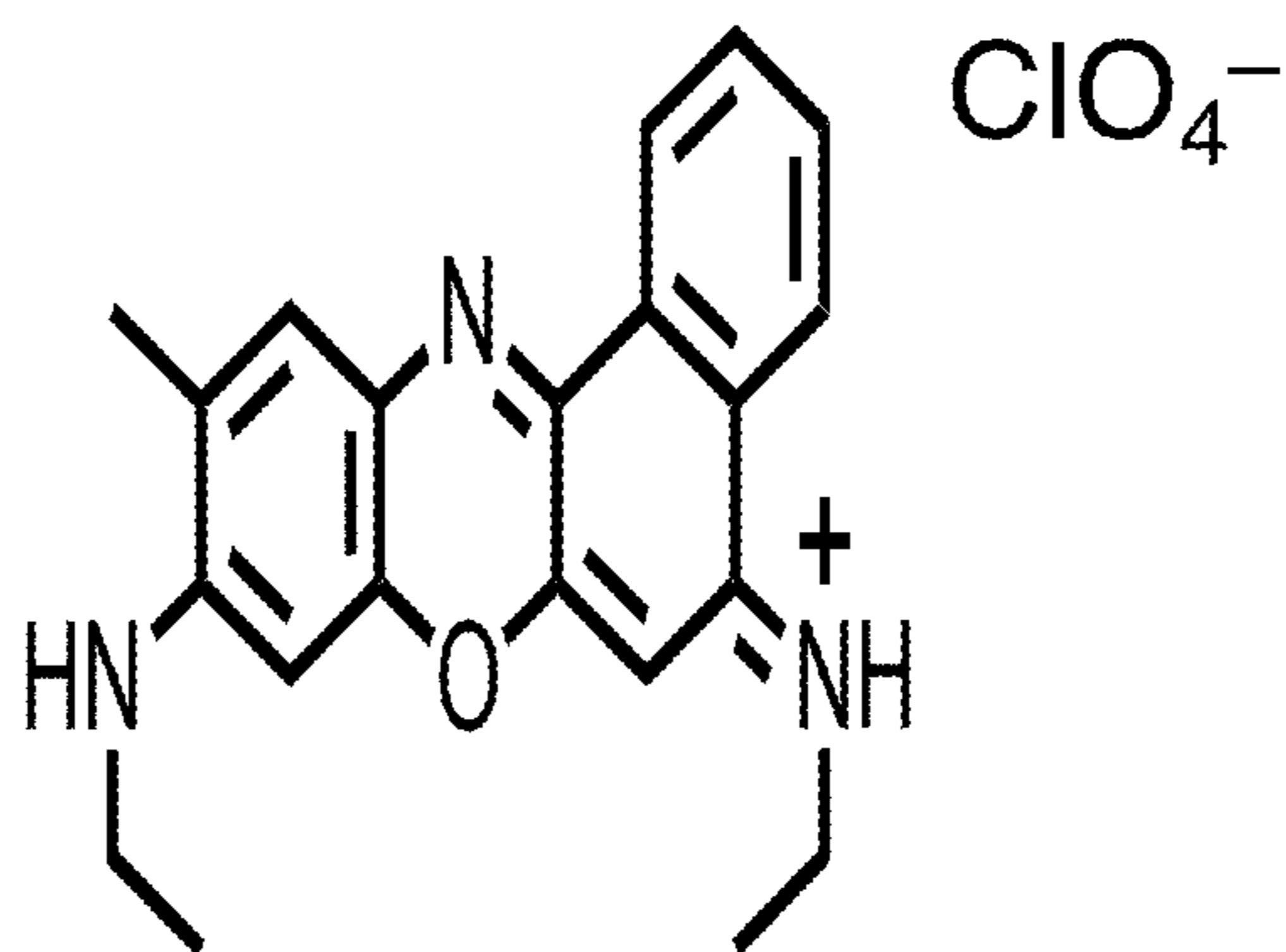
Oxazine 720·ClO 4
