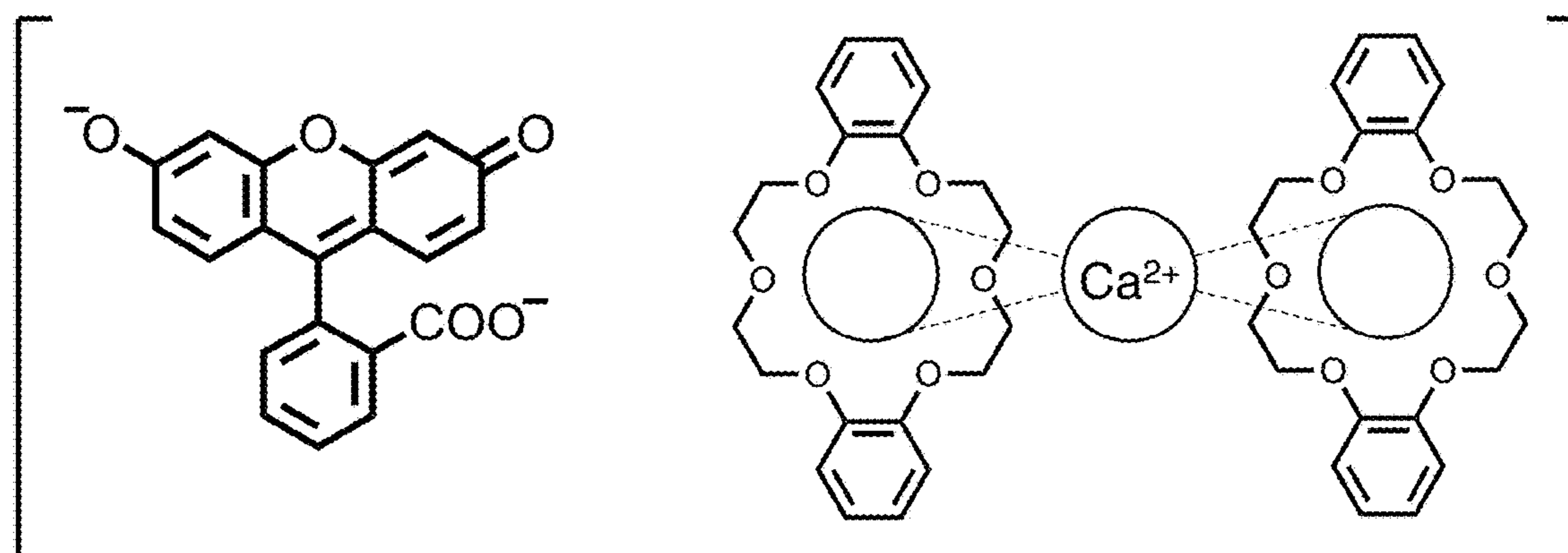
(VI-5)
