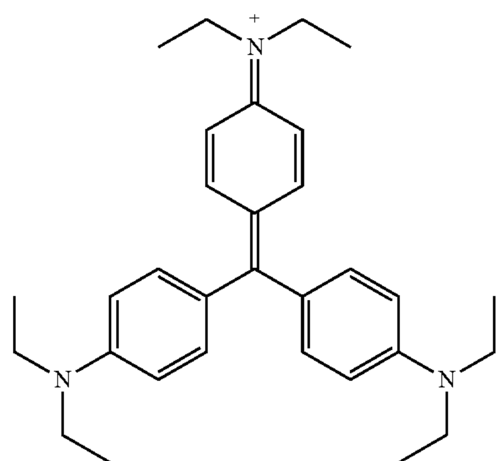
(Ethyl violet)
