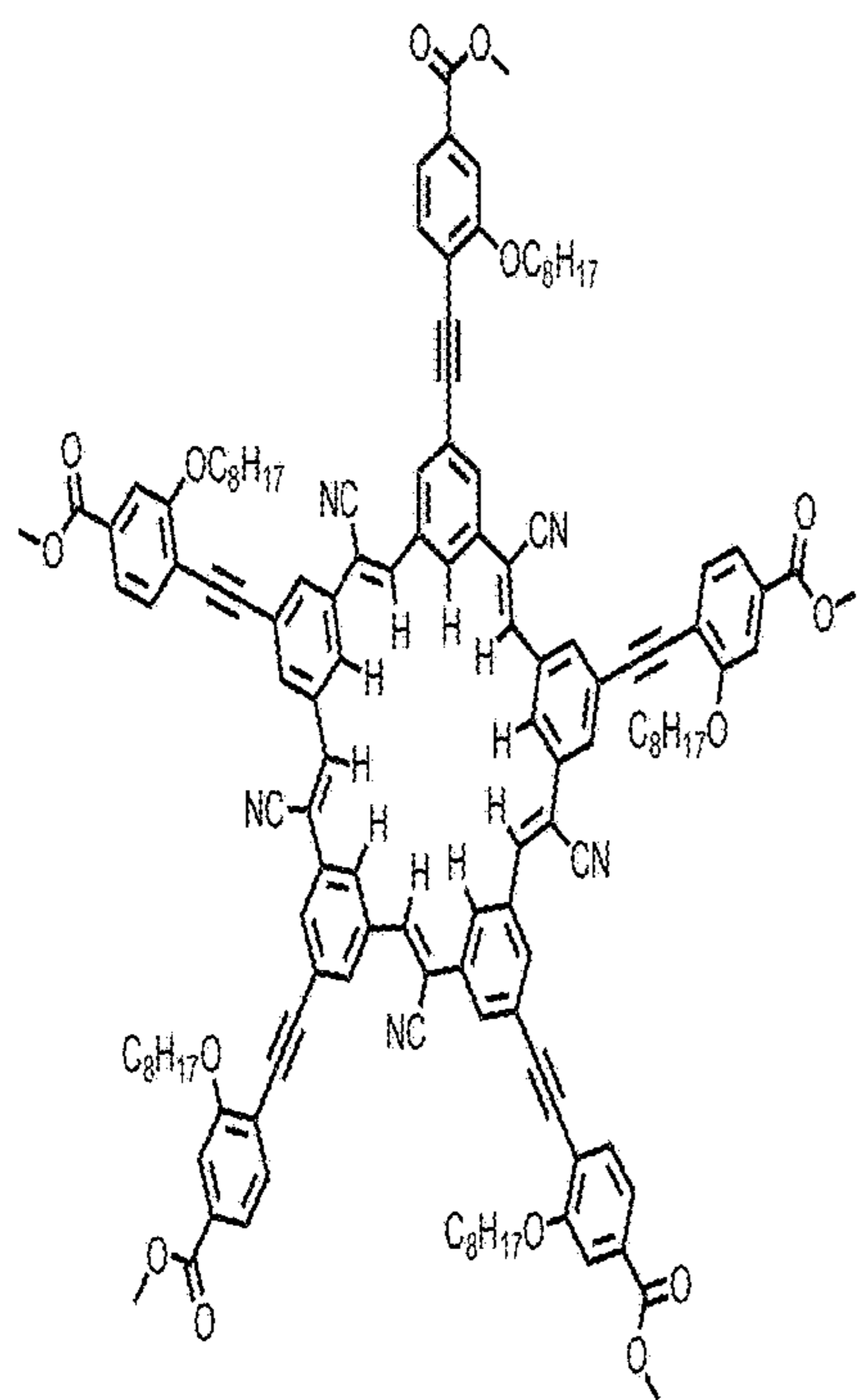
Cyanostar 2
