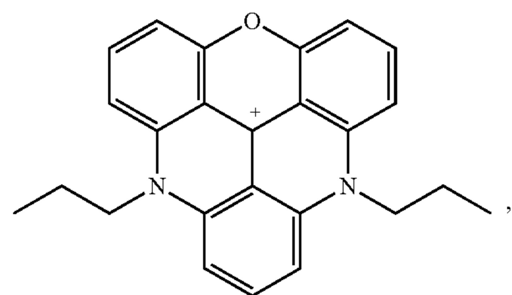
(DAOTA)
