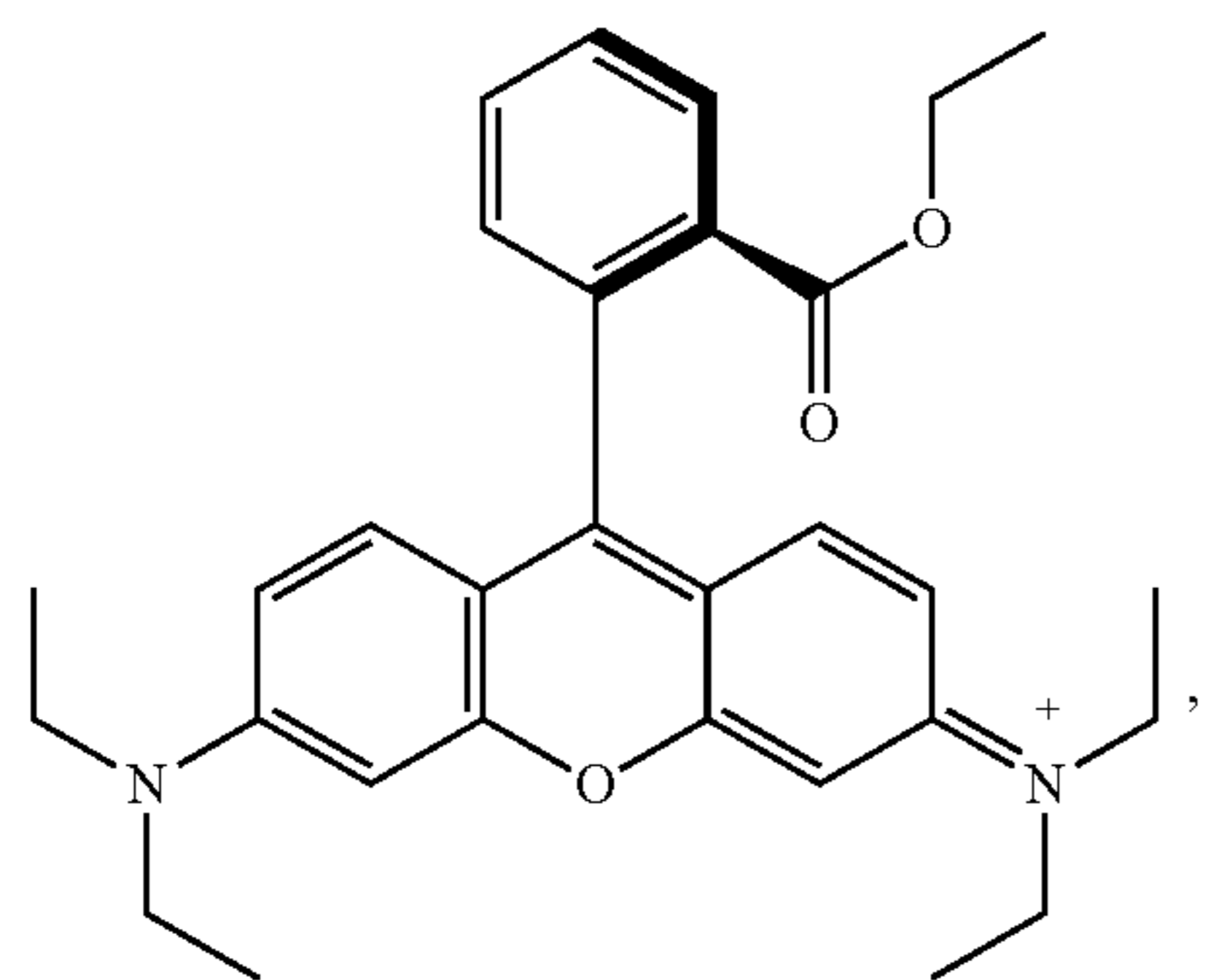
(Rhodamine 3B)
