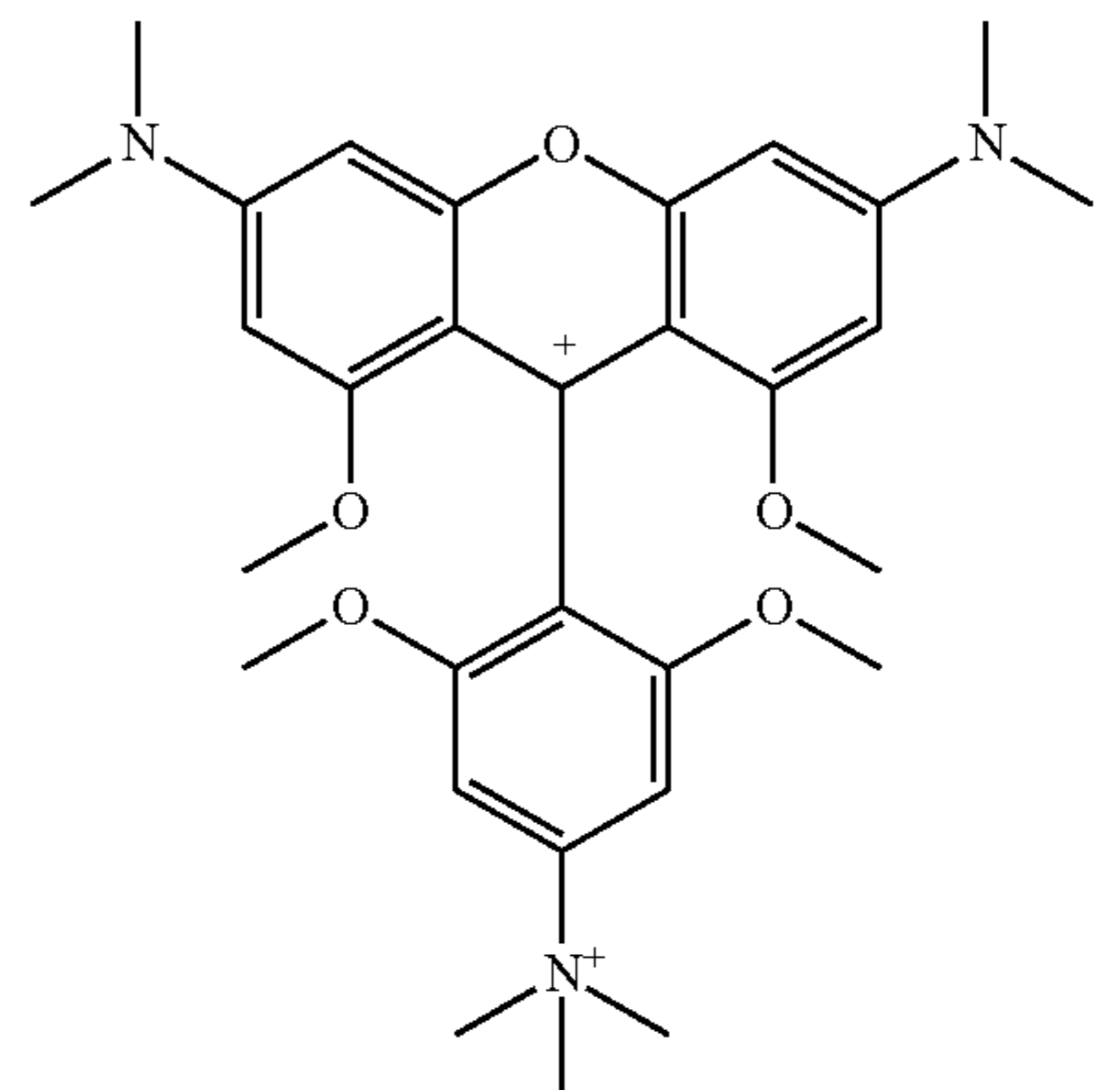
(Tetramethoxy-aminorhodamine)
