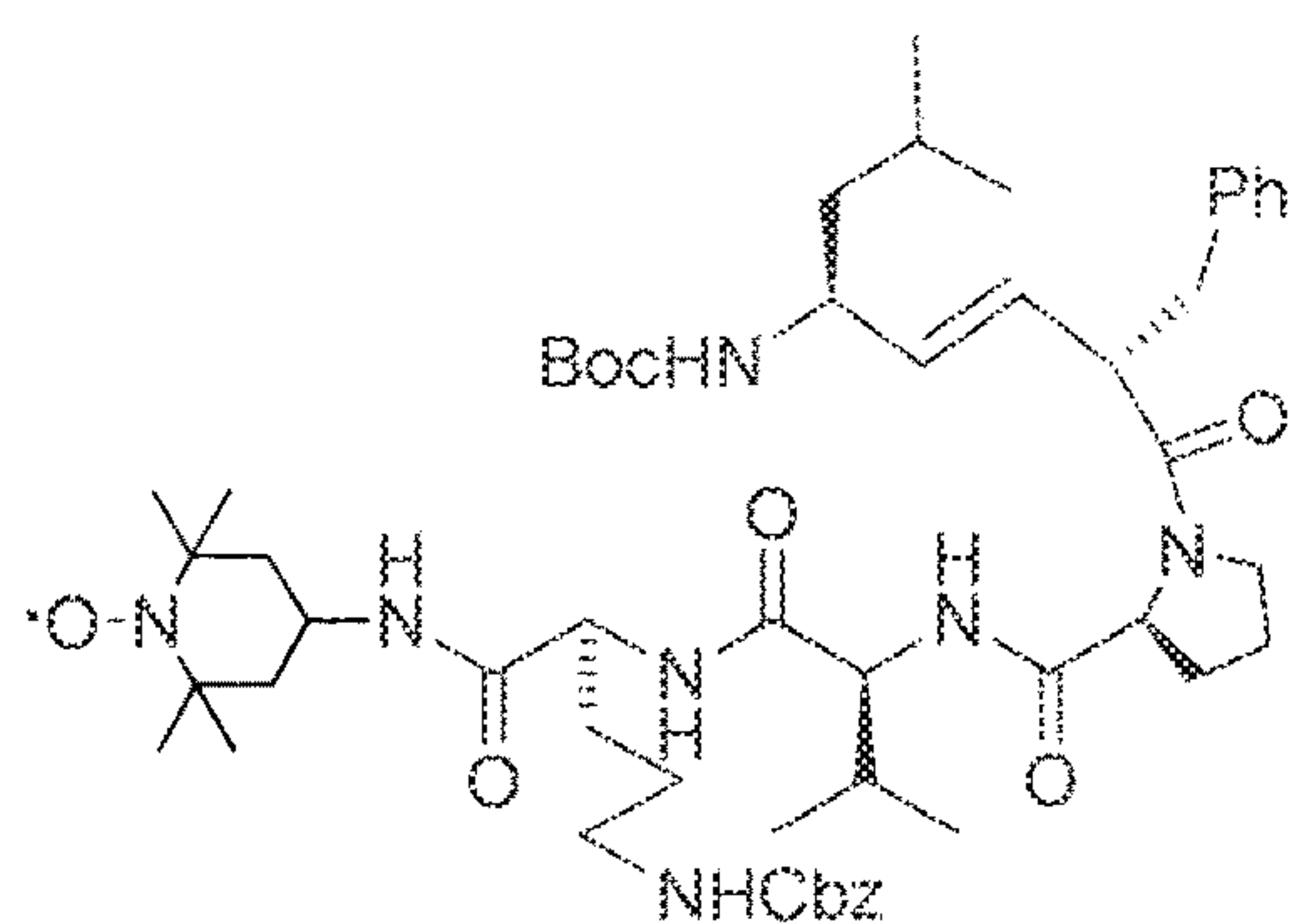
XJB-5-131
