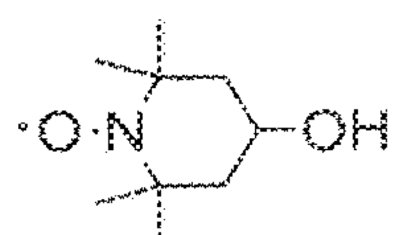
TEMPOL
