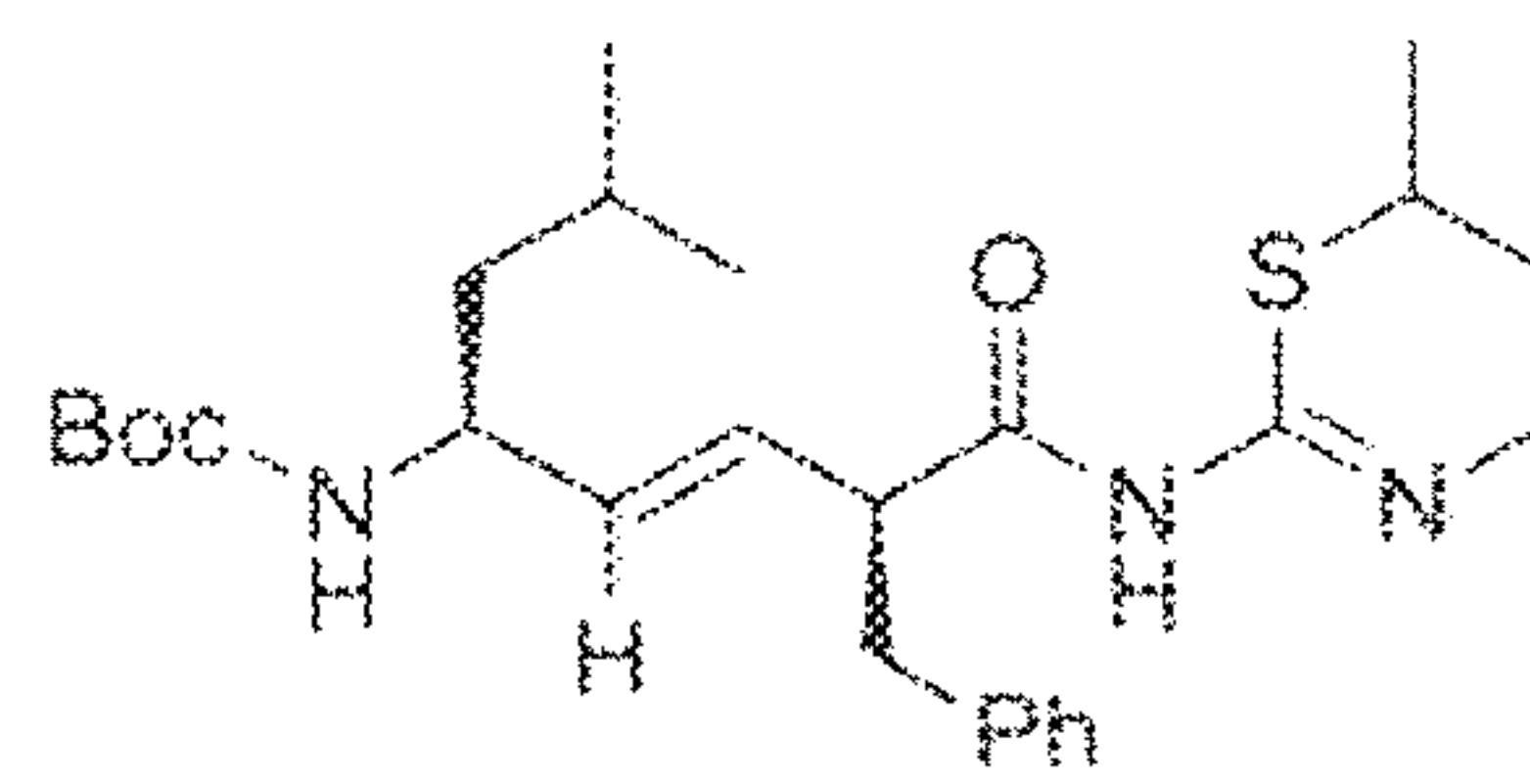
XJB-5-234
