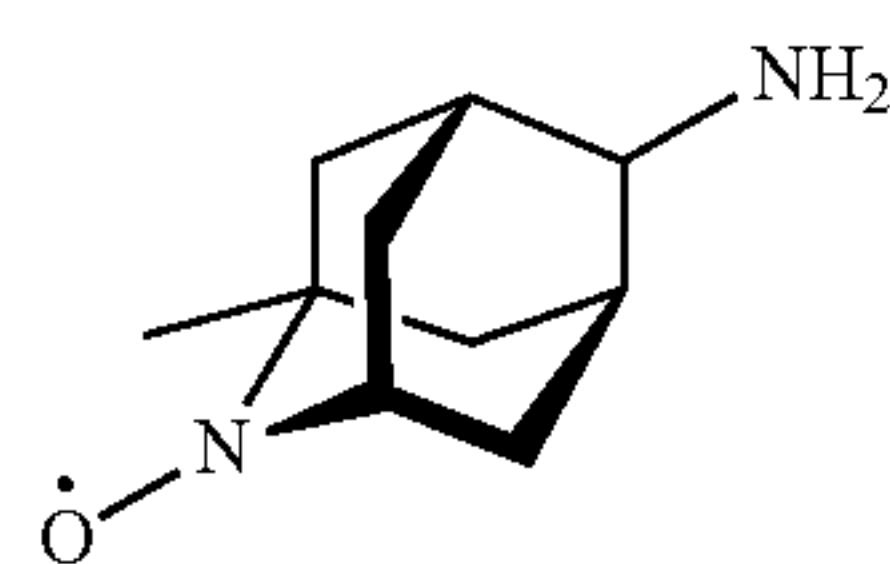
6-amino-1-Me-AZADO
