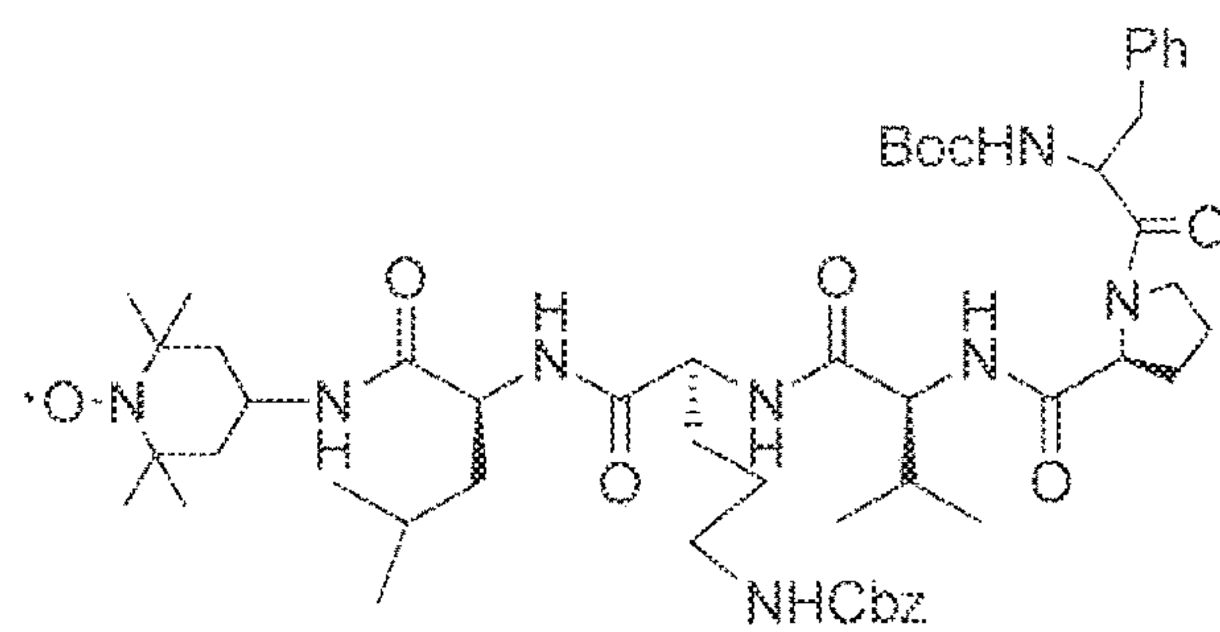
XJB-7-75
