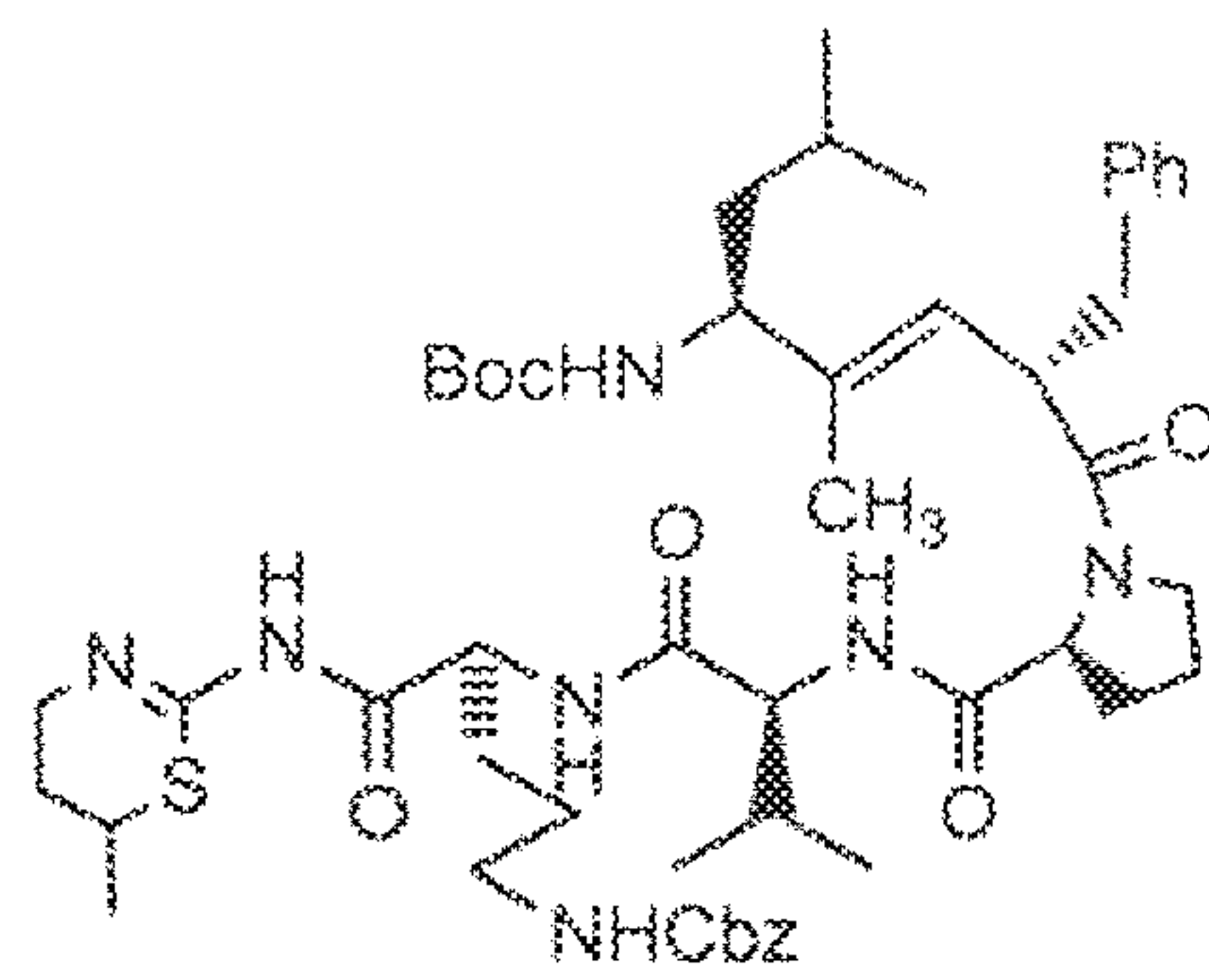
XJB-5-241
