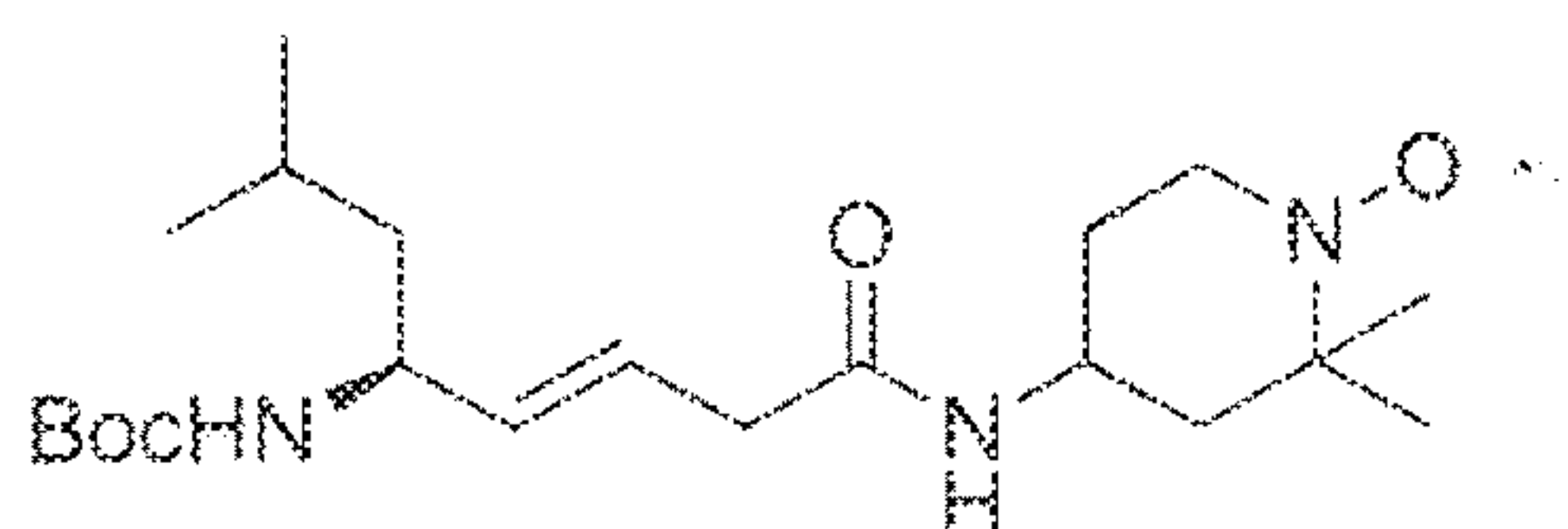
JP4-039
