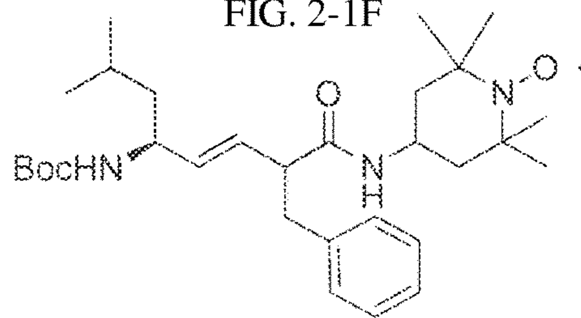
JP4-049
