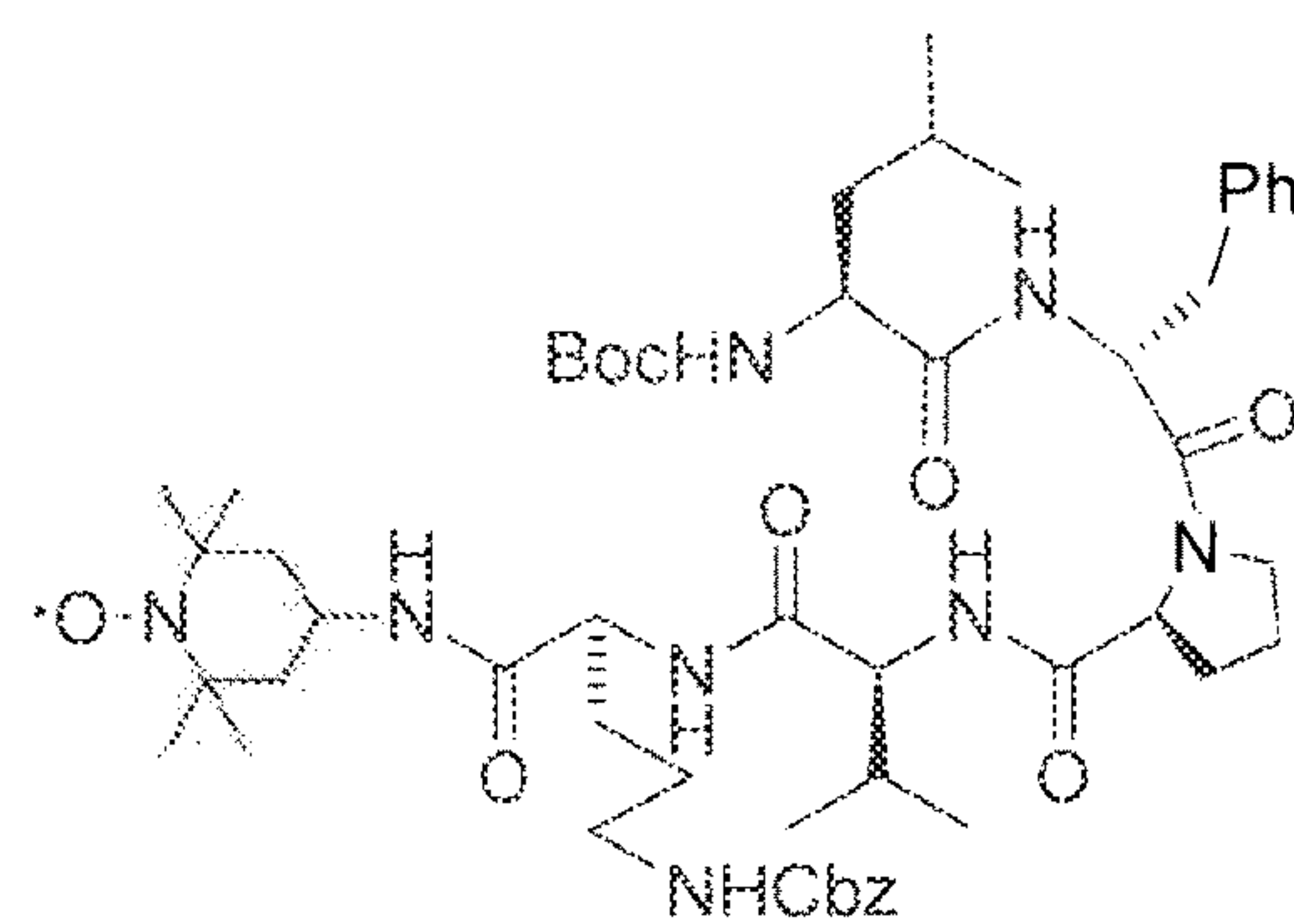
XJB-5-125
