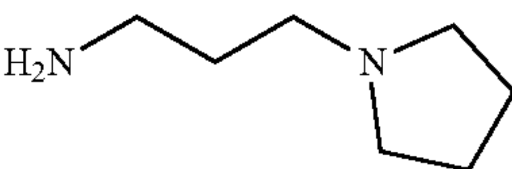
1-(3-aminopropyl)pyrrolidine
