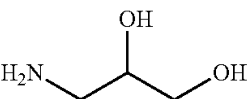
3-aminopropane-1,2-diol
