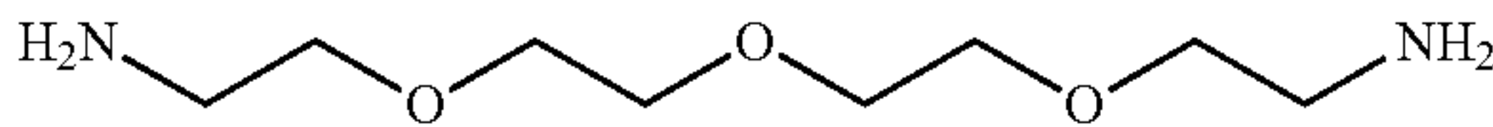
(PEO)4-bis-amine
