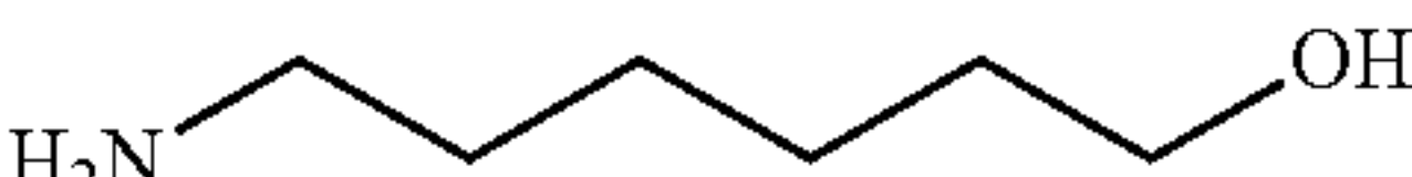
6-amino-1-hexanol
