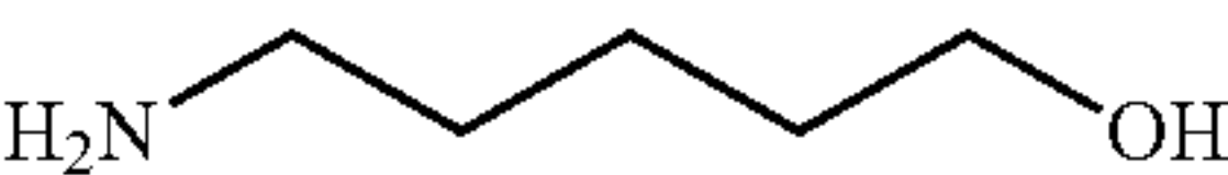
5-amino-1-pentanol
