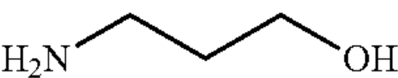
3-amino-1-propanol
