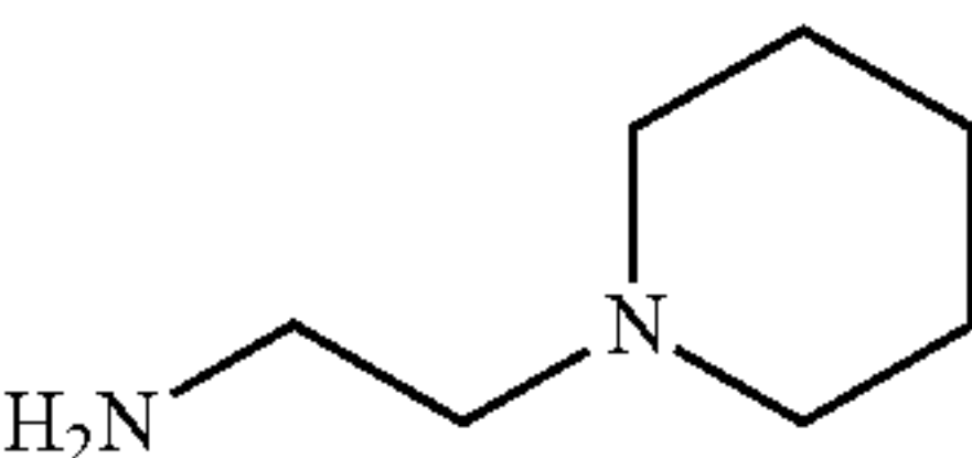
1-(2-aminoethyl)piperidine
