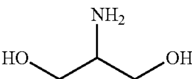
2-aminopropane-1,3-diol
