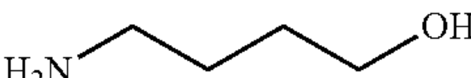
4-amino-1-butanol
