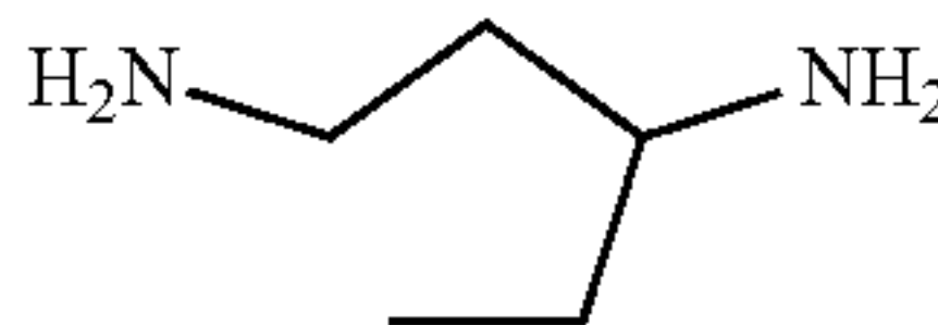
pentane-1,3-diamine
