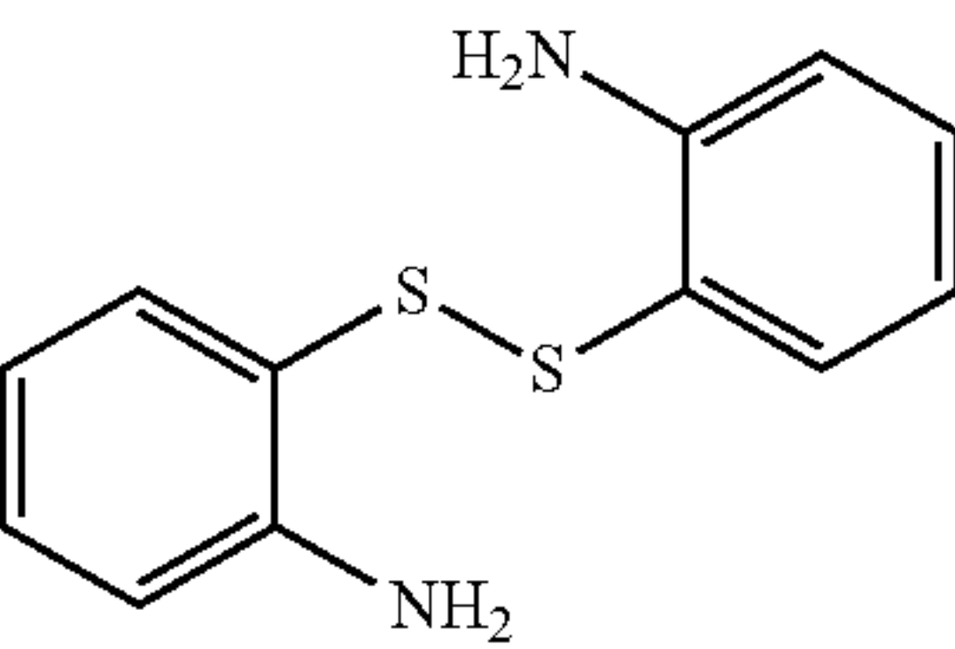
2,2'-dithiobis-benzenamine
