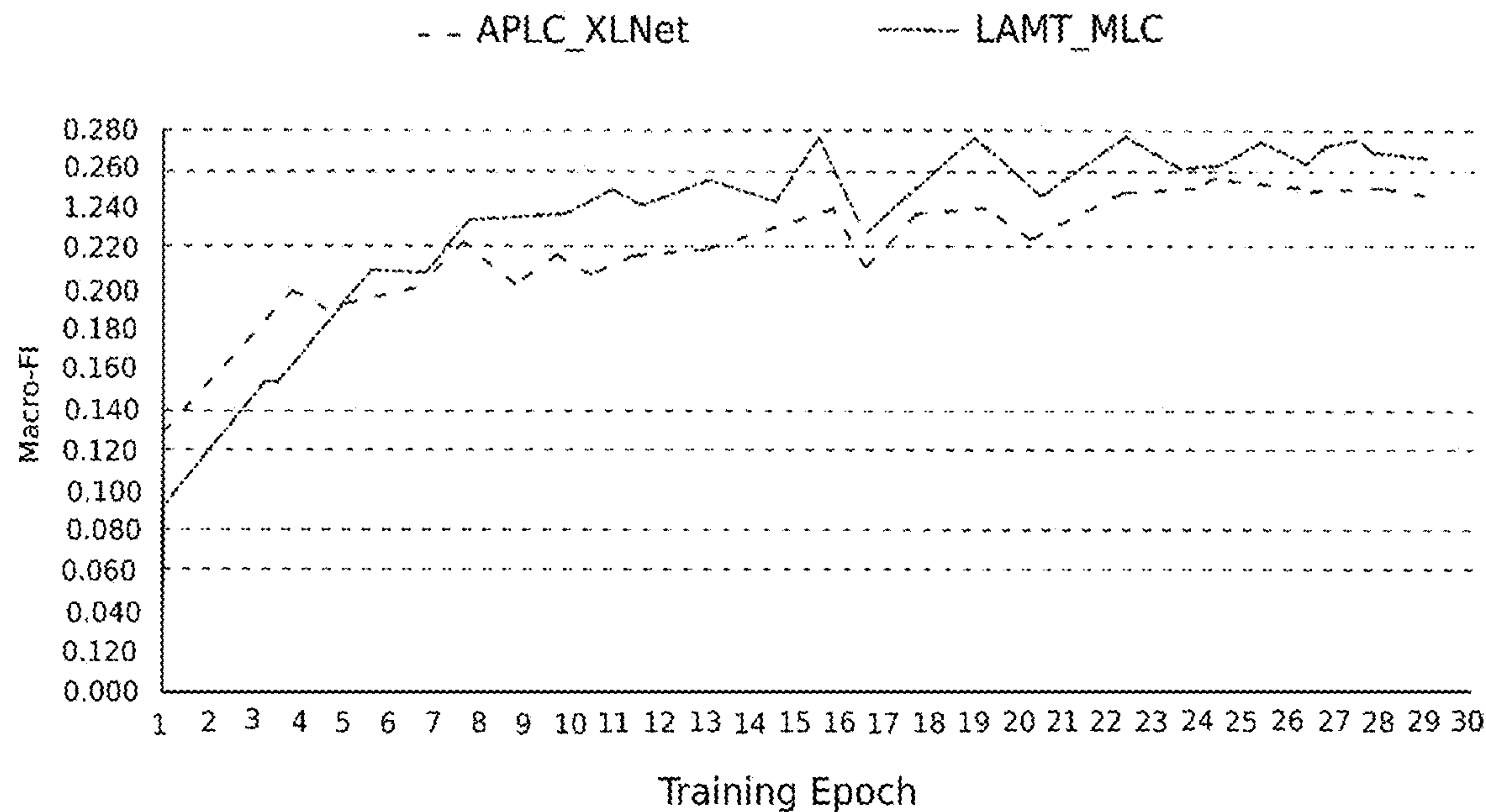
Fig. 7B Macro-F1
