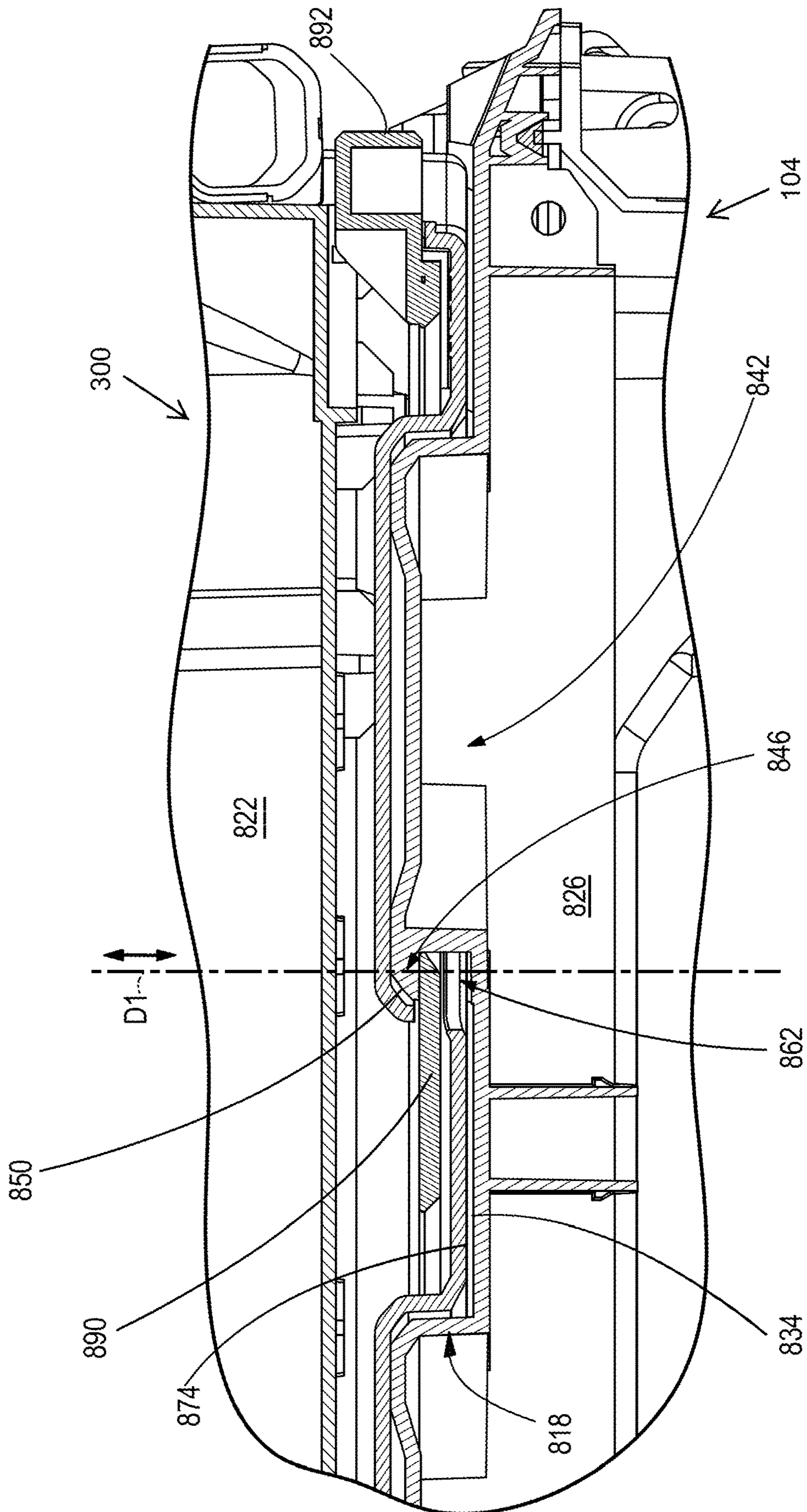
FIG. 31A
