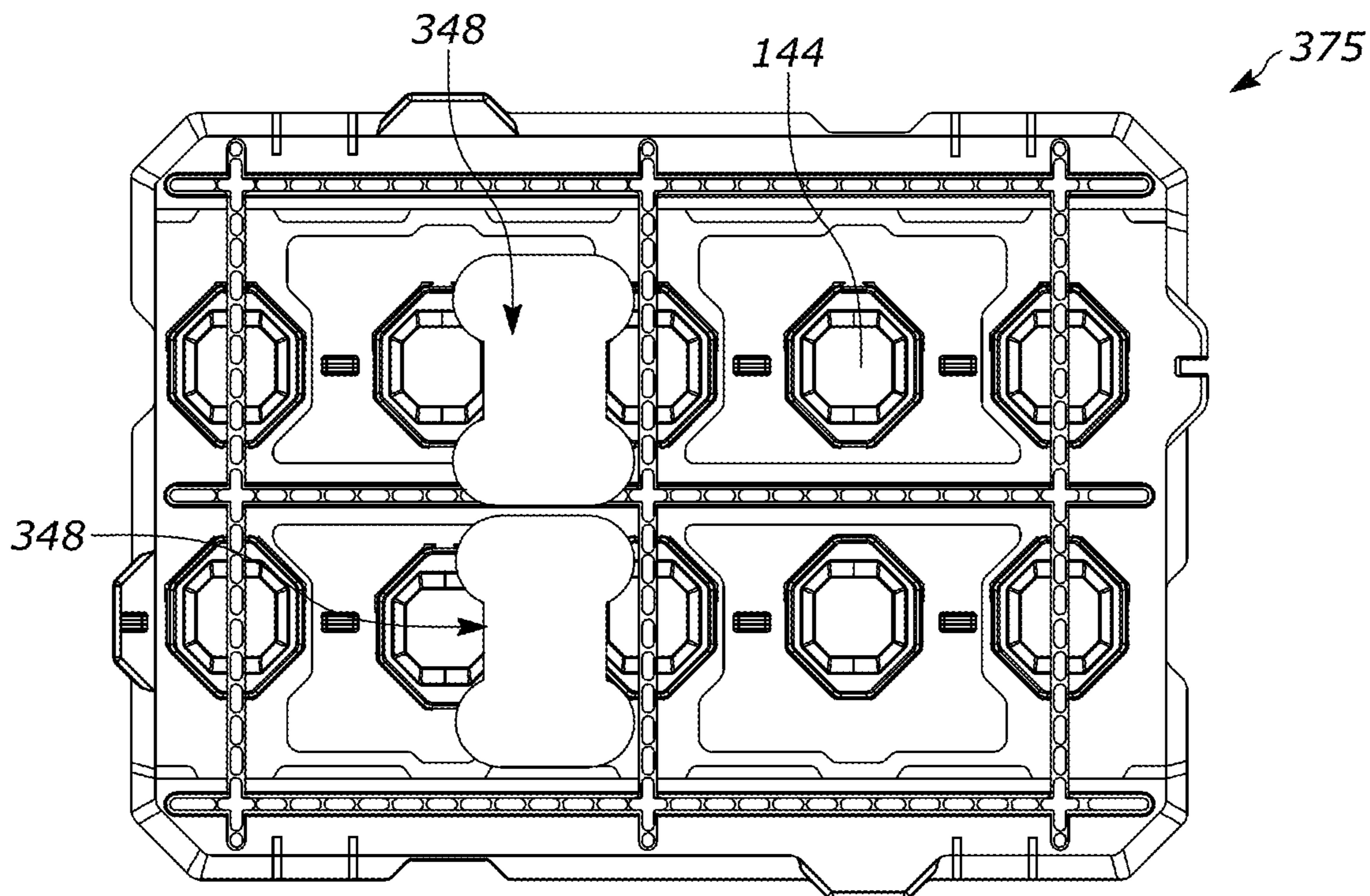
FIG. 19B
