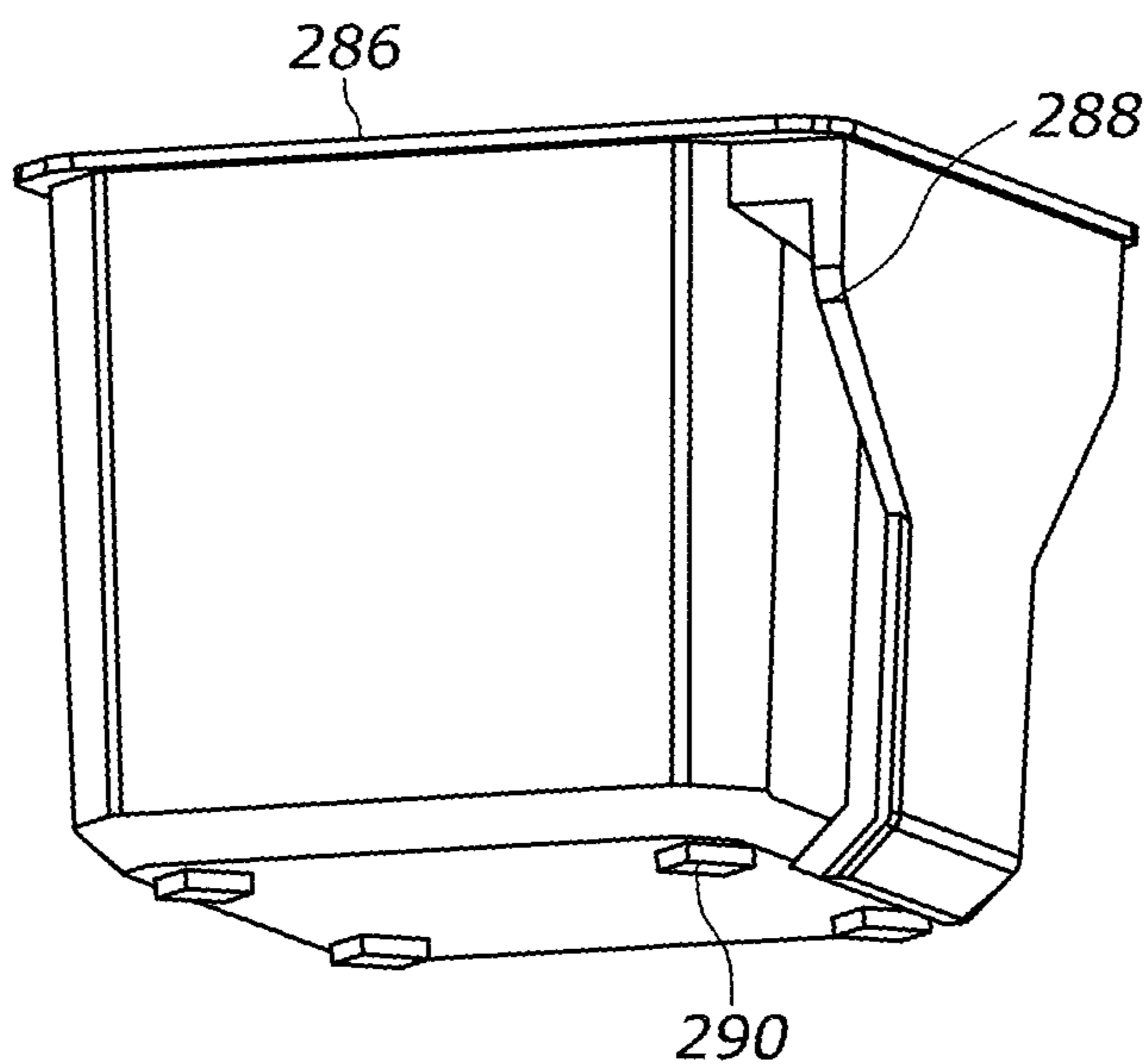
FIG. 16D
