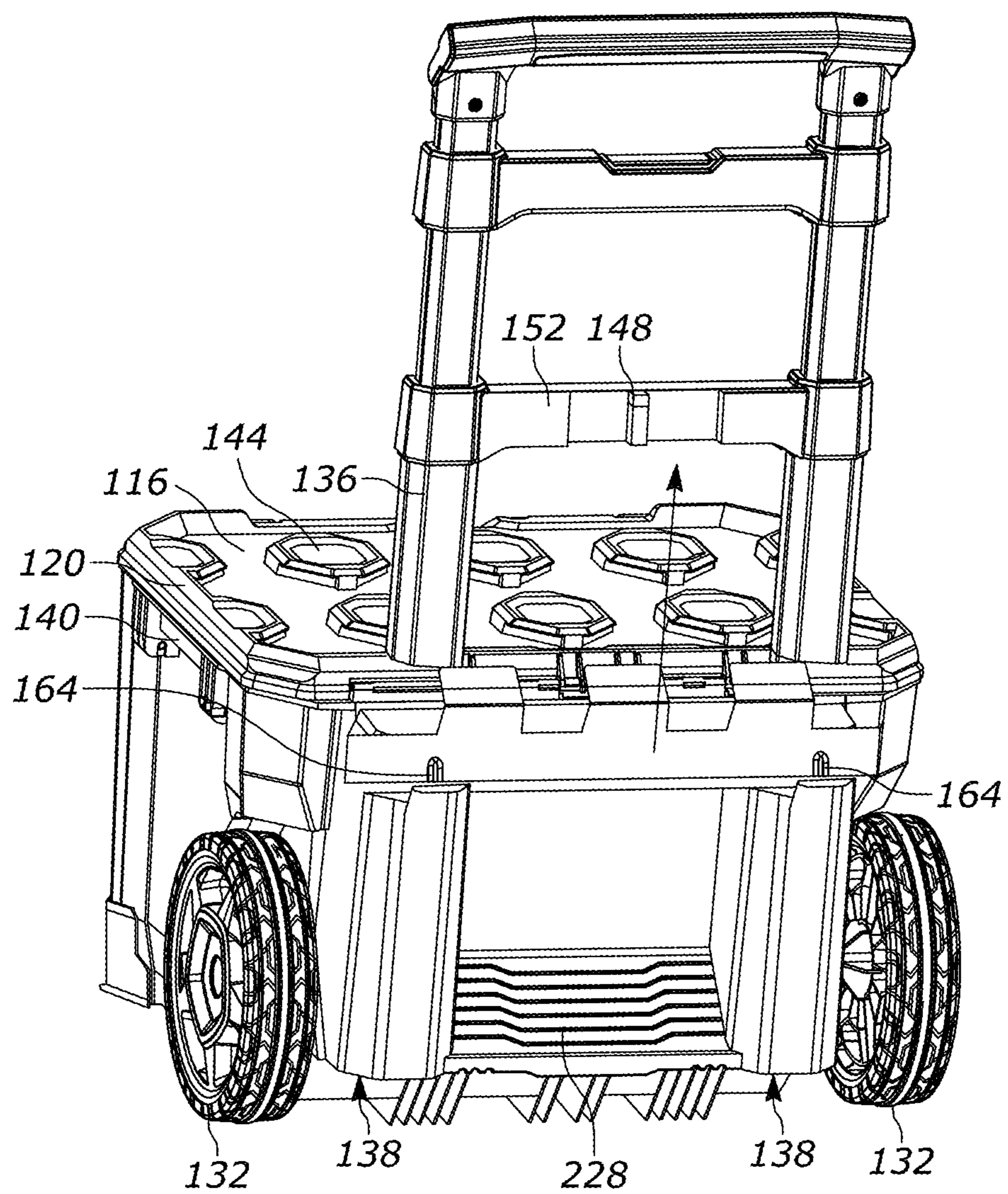
FIG. 4
