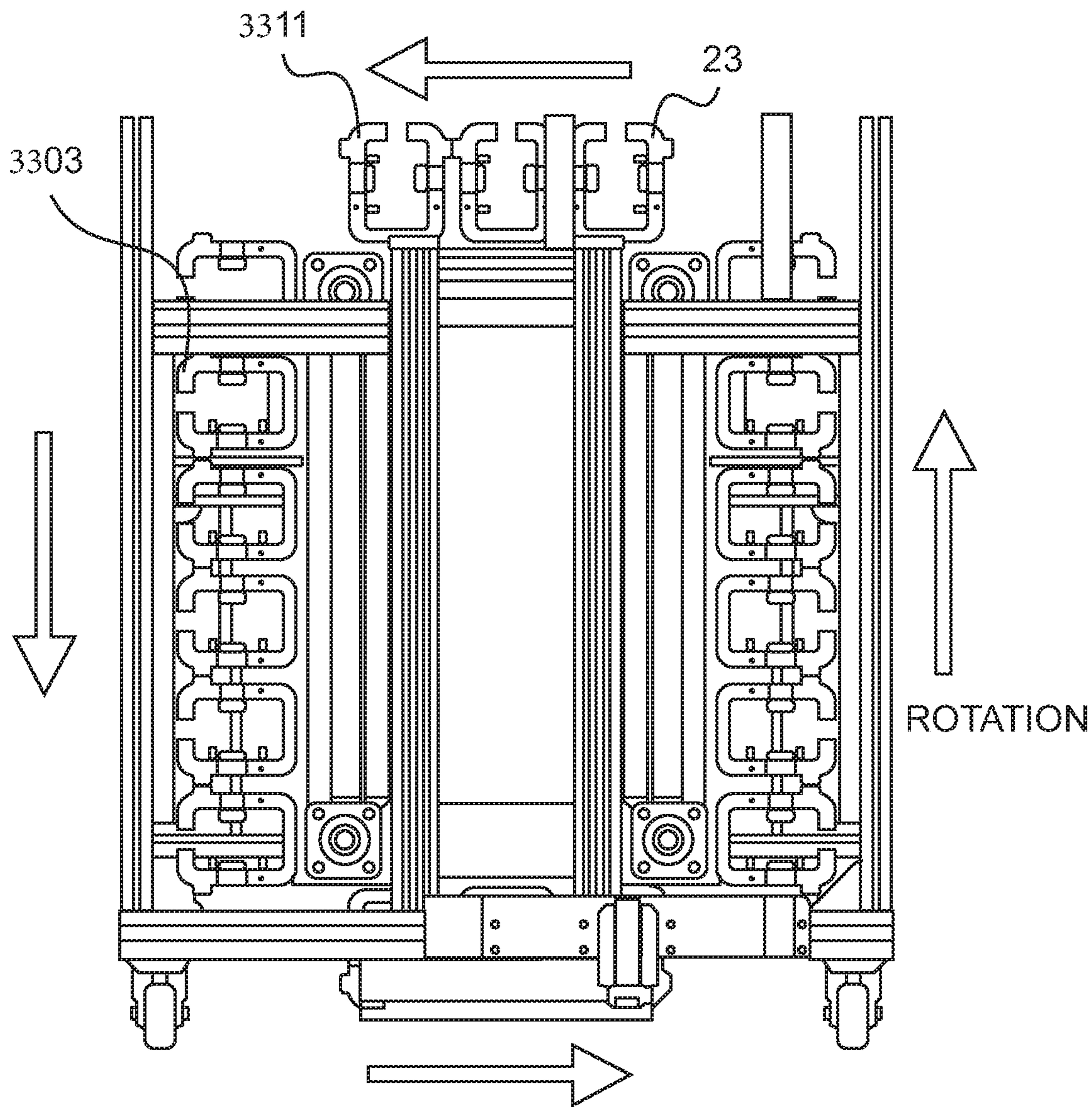
FIG. 33C
