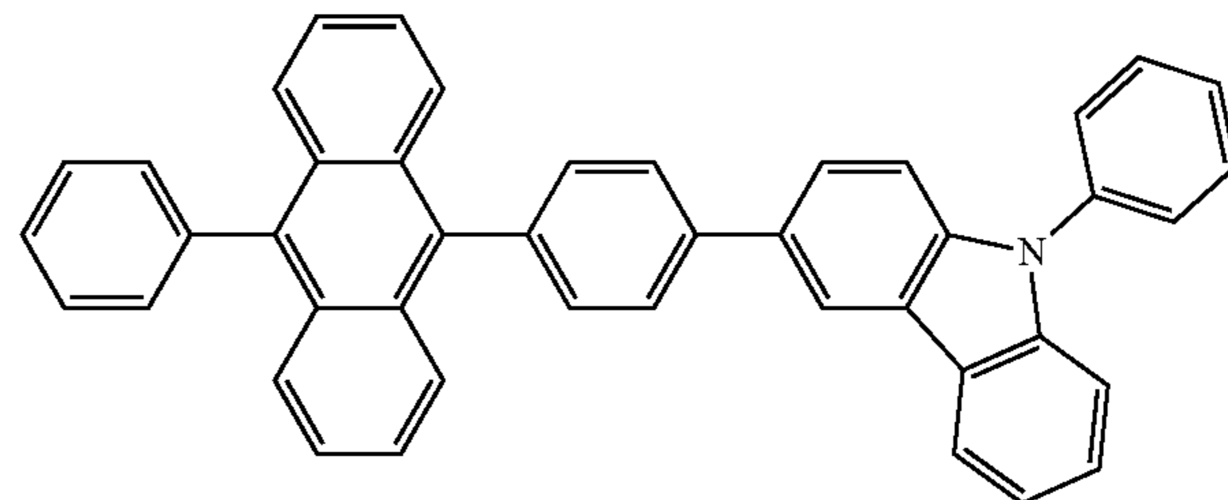
PCzPA
