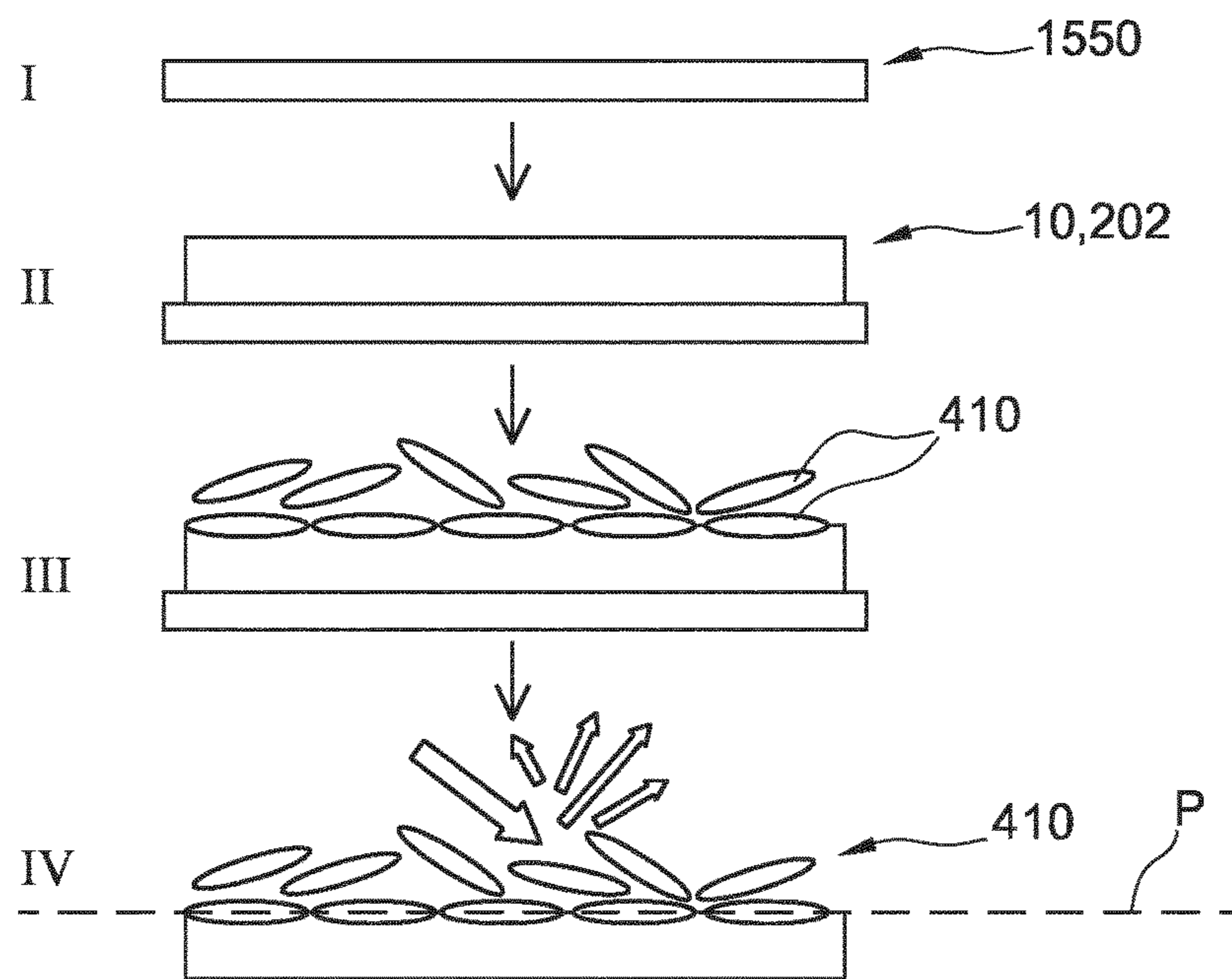
FIG. 2A
