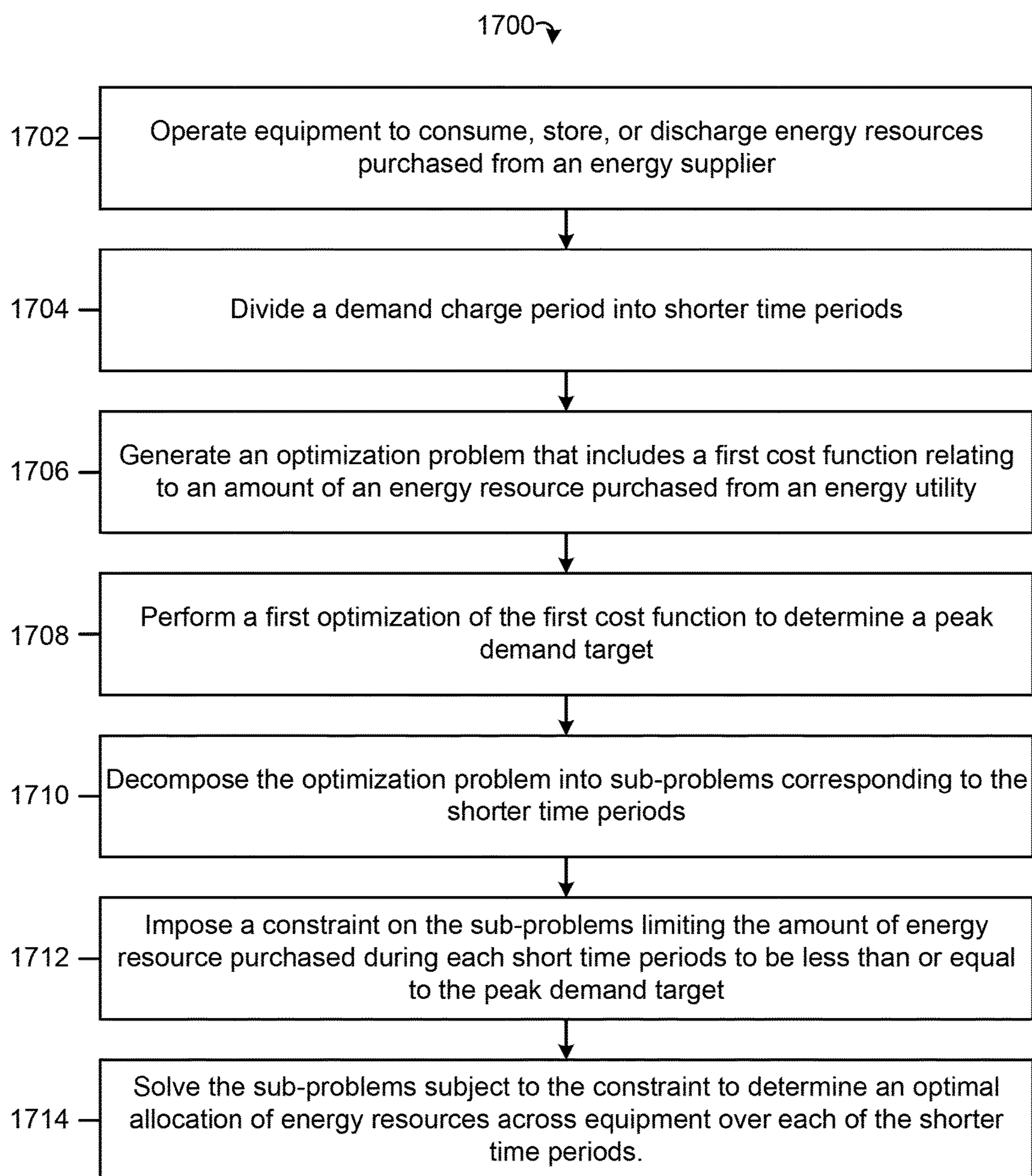
FIG. 17
