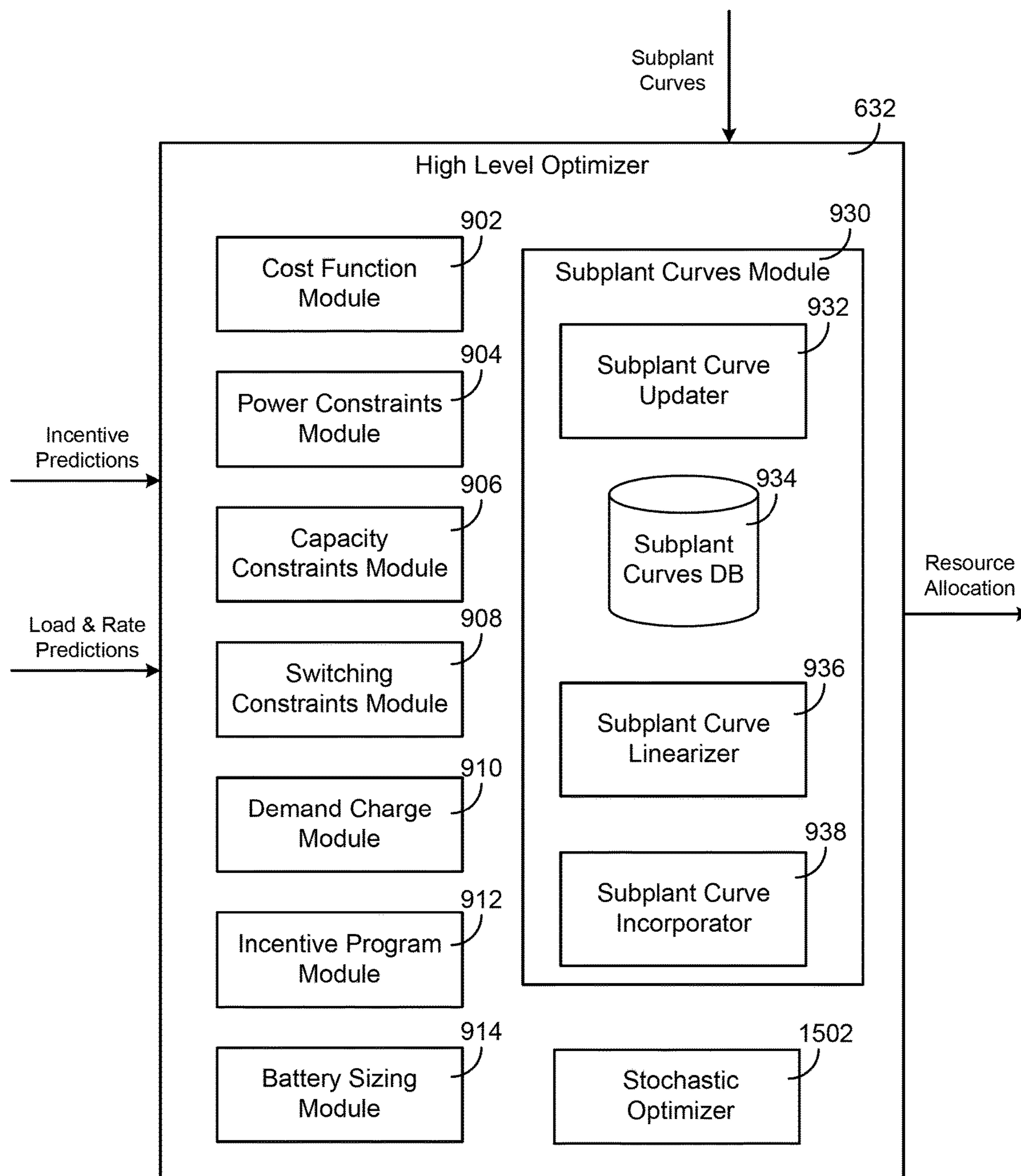
FIG. 9A
