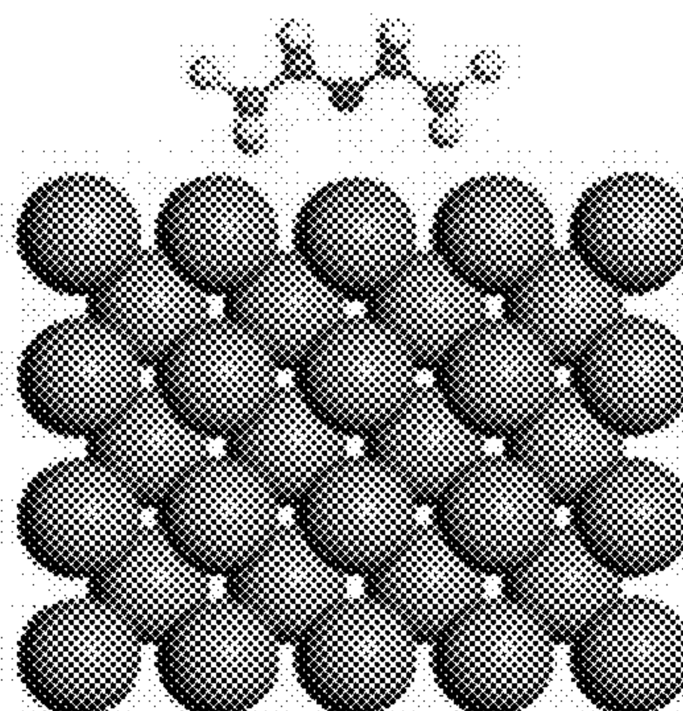
BTFE
