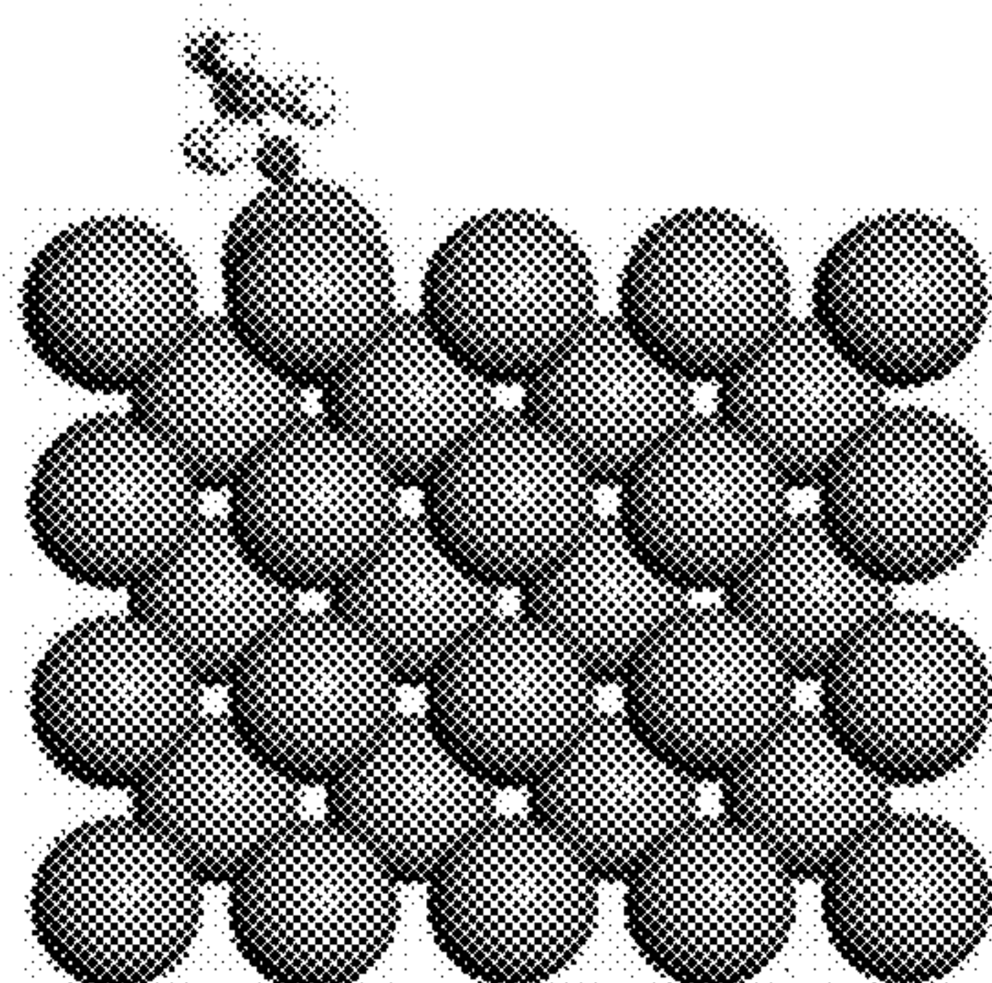
DMC
