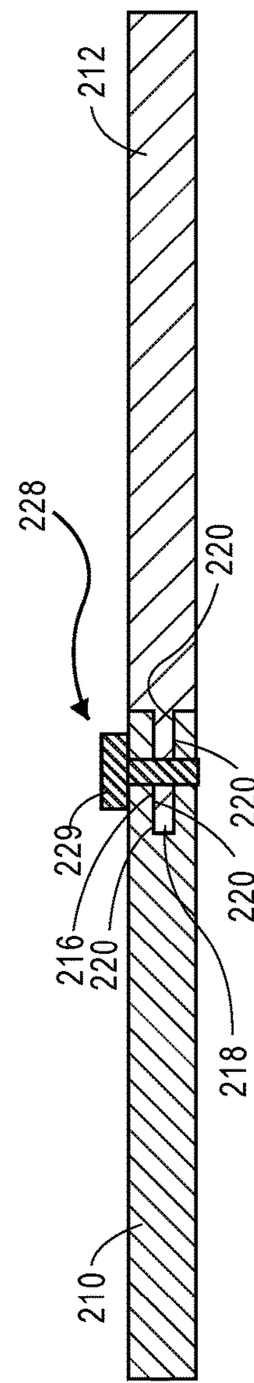
FIG. 9D
