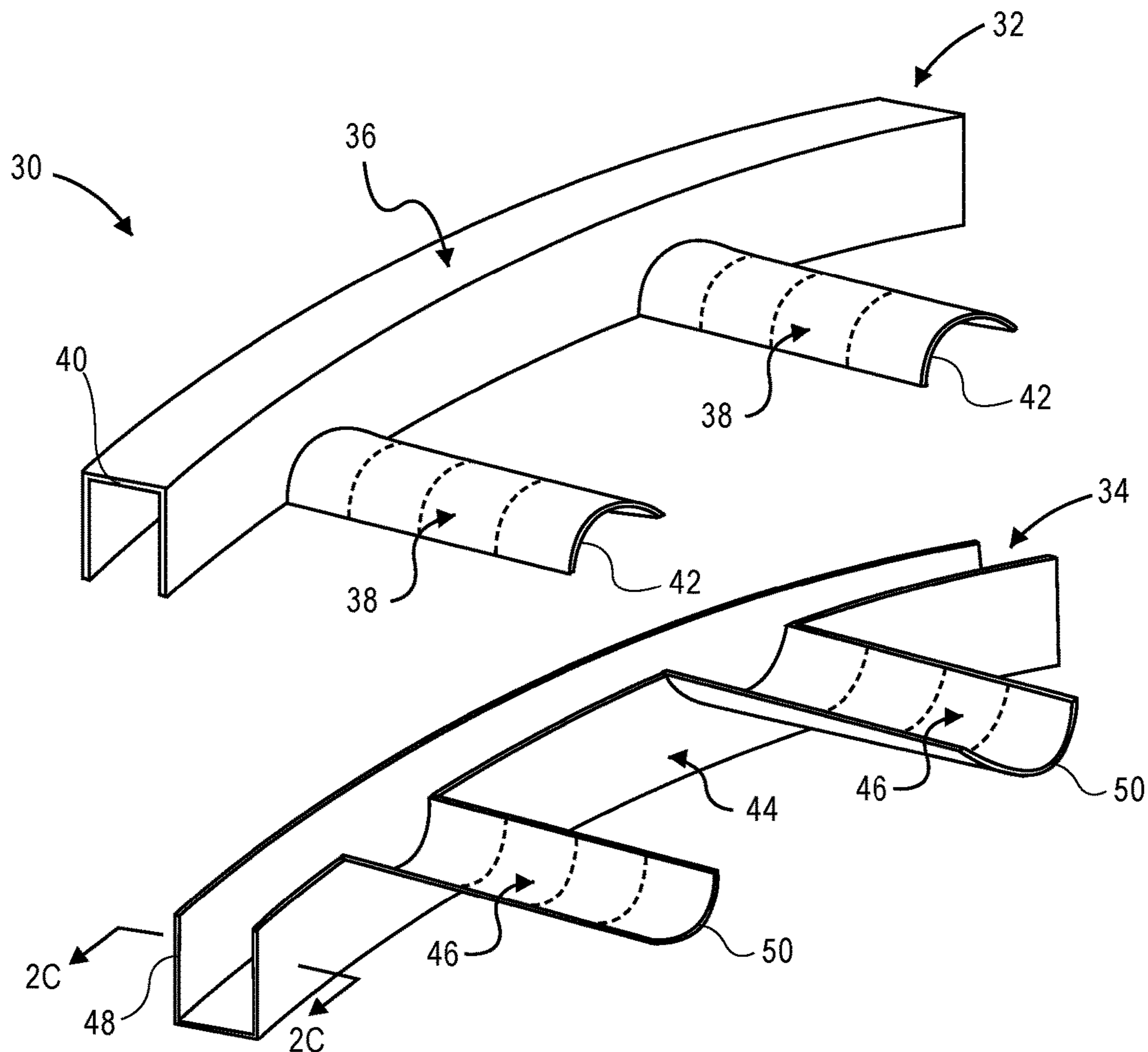
FIG. 2A
