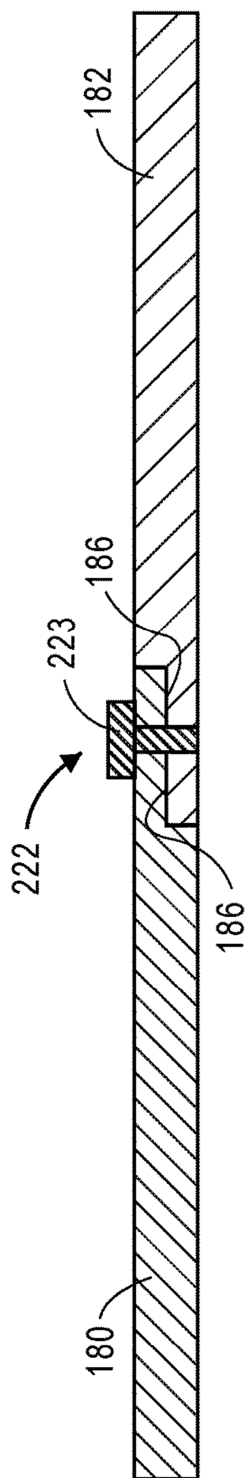
FIG. 9A
