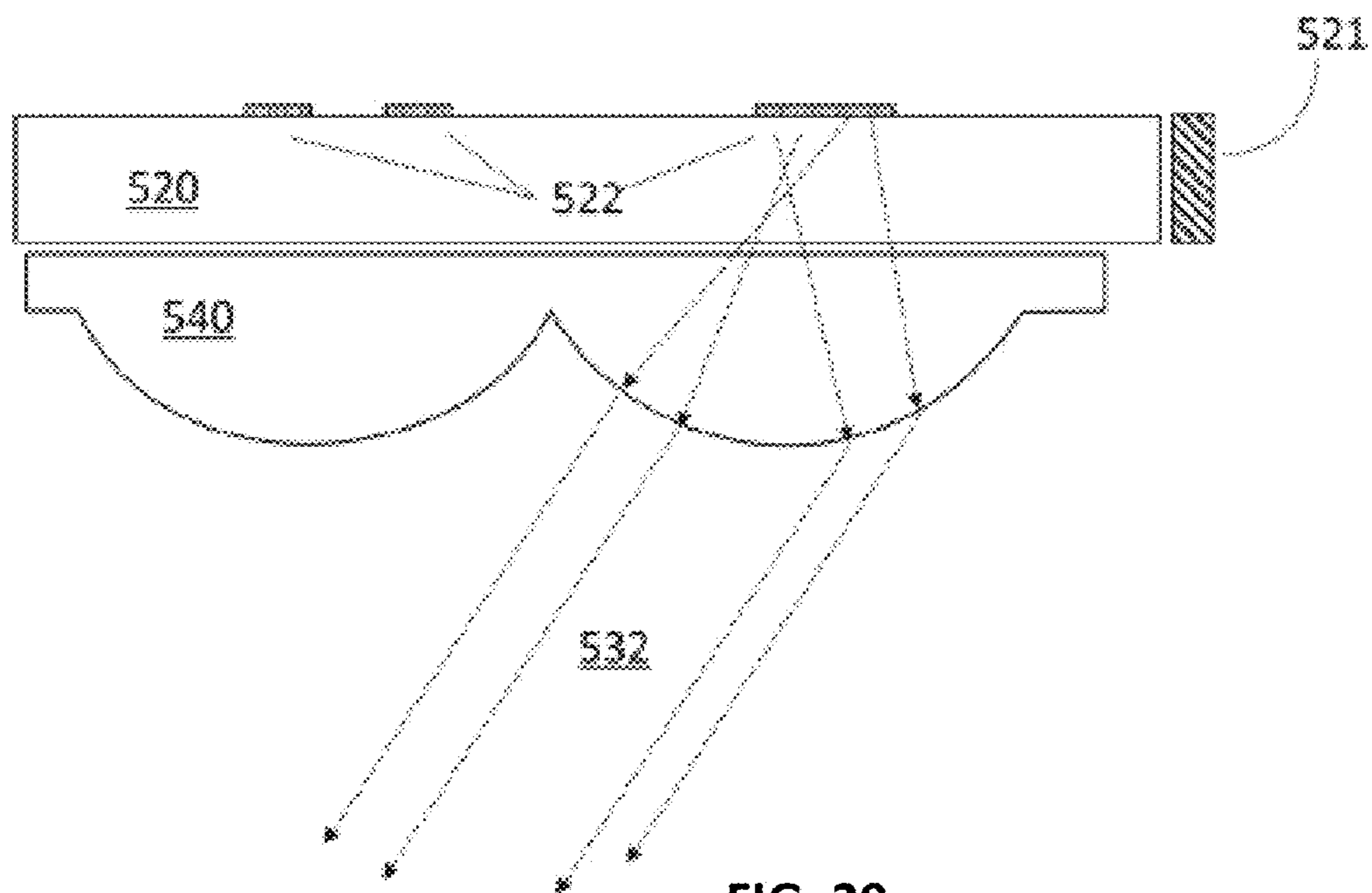
FIG. 29
