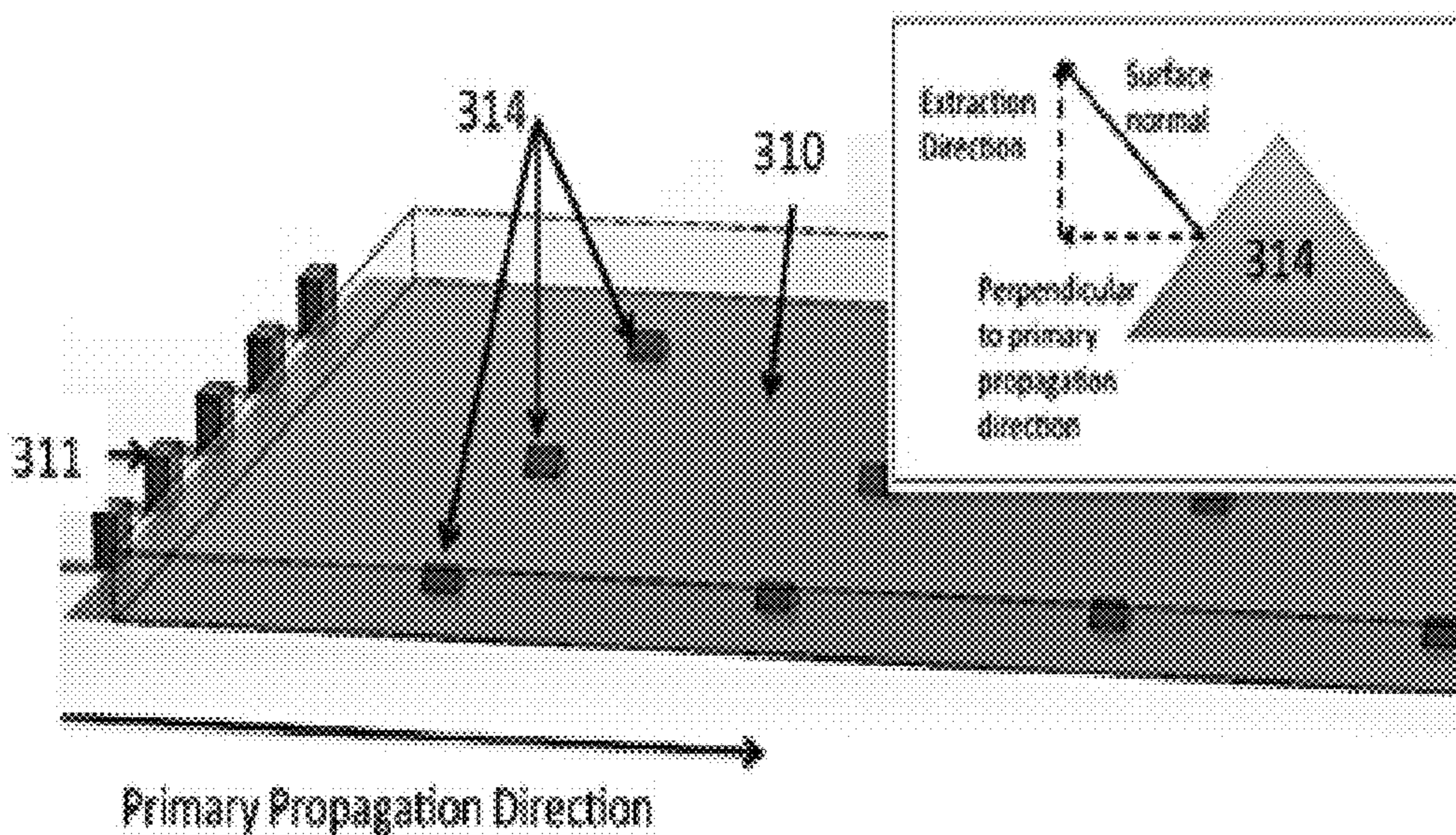
FIG. 23B
