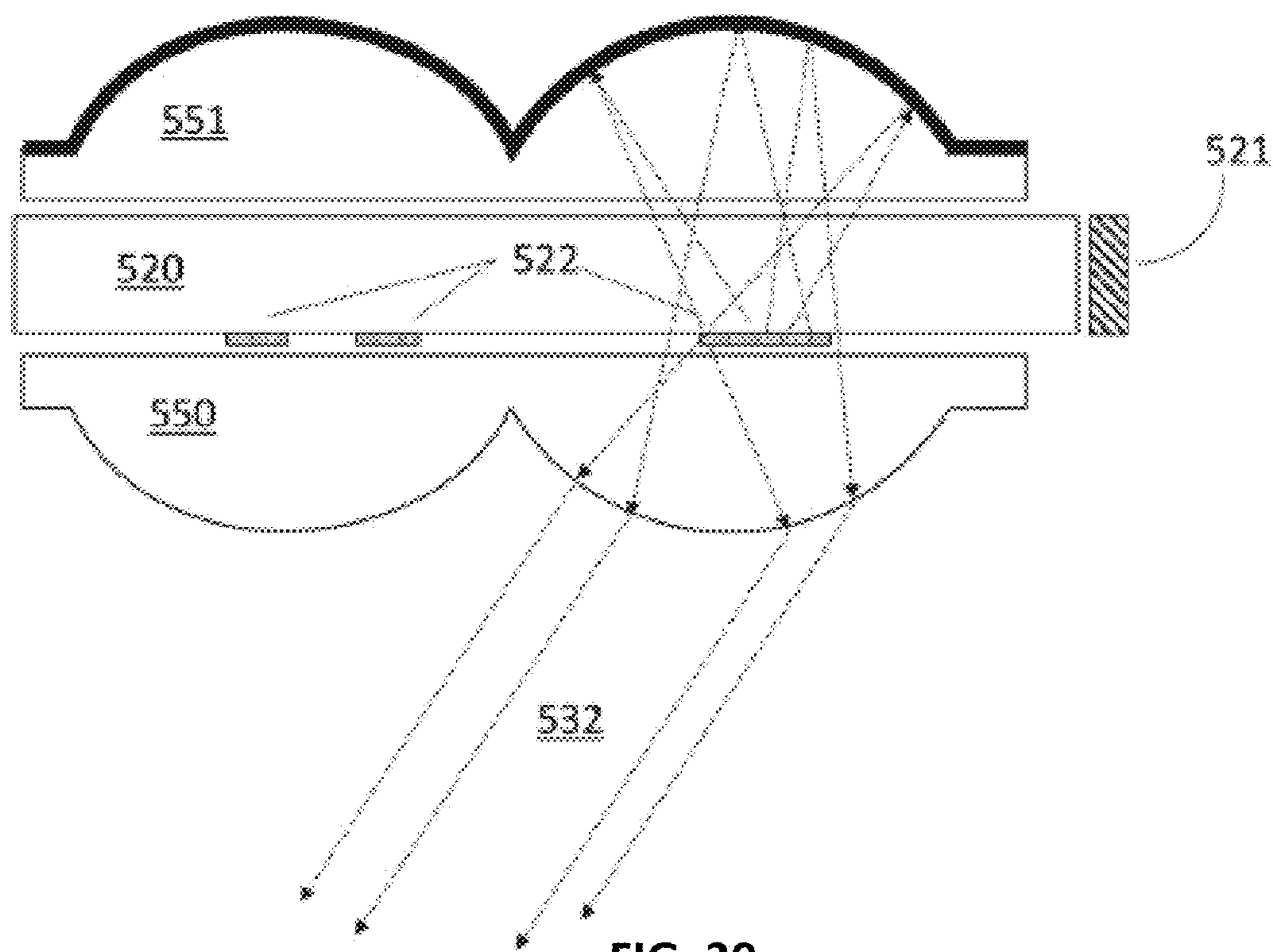
FIG. 30
