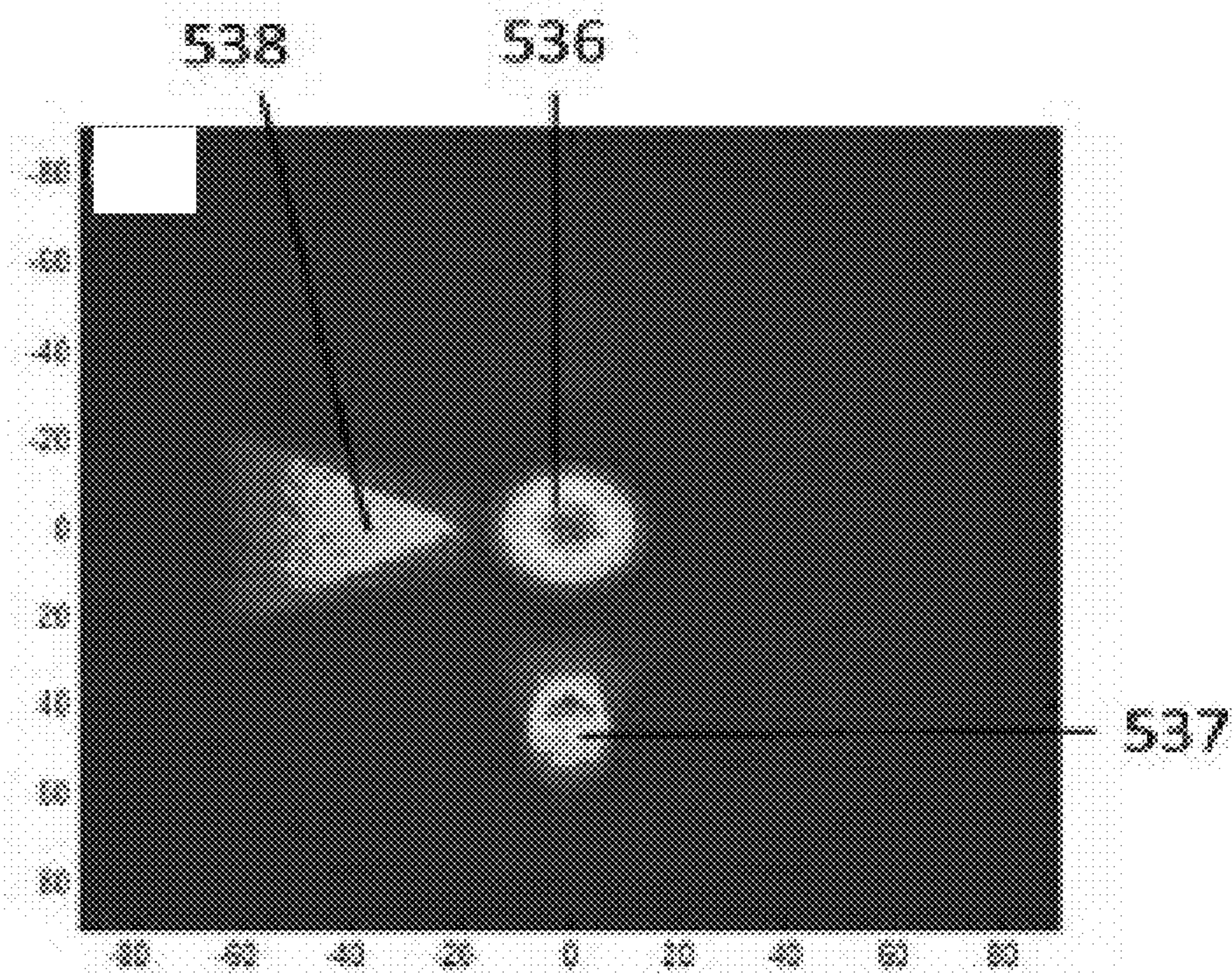
FIG. 28B
