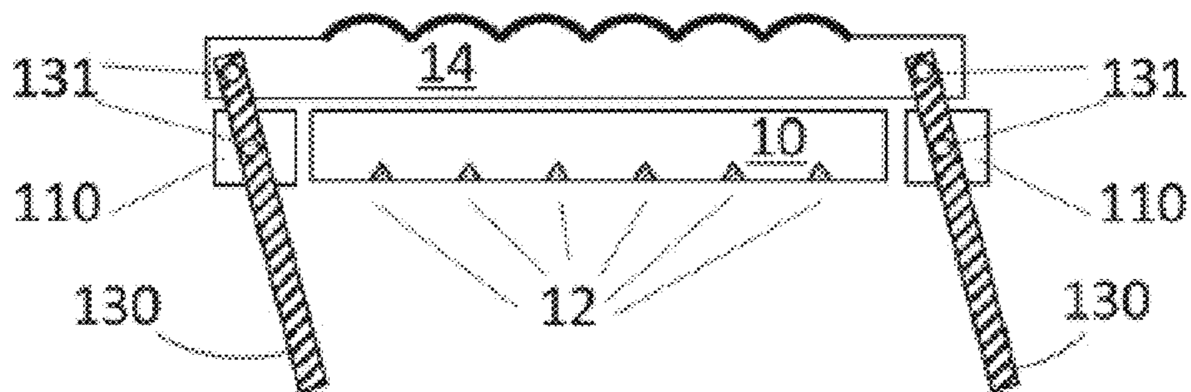
FIG. 17
