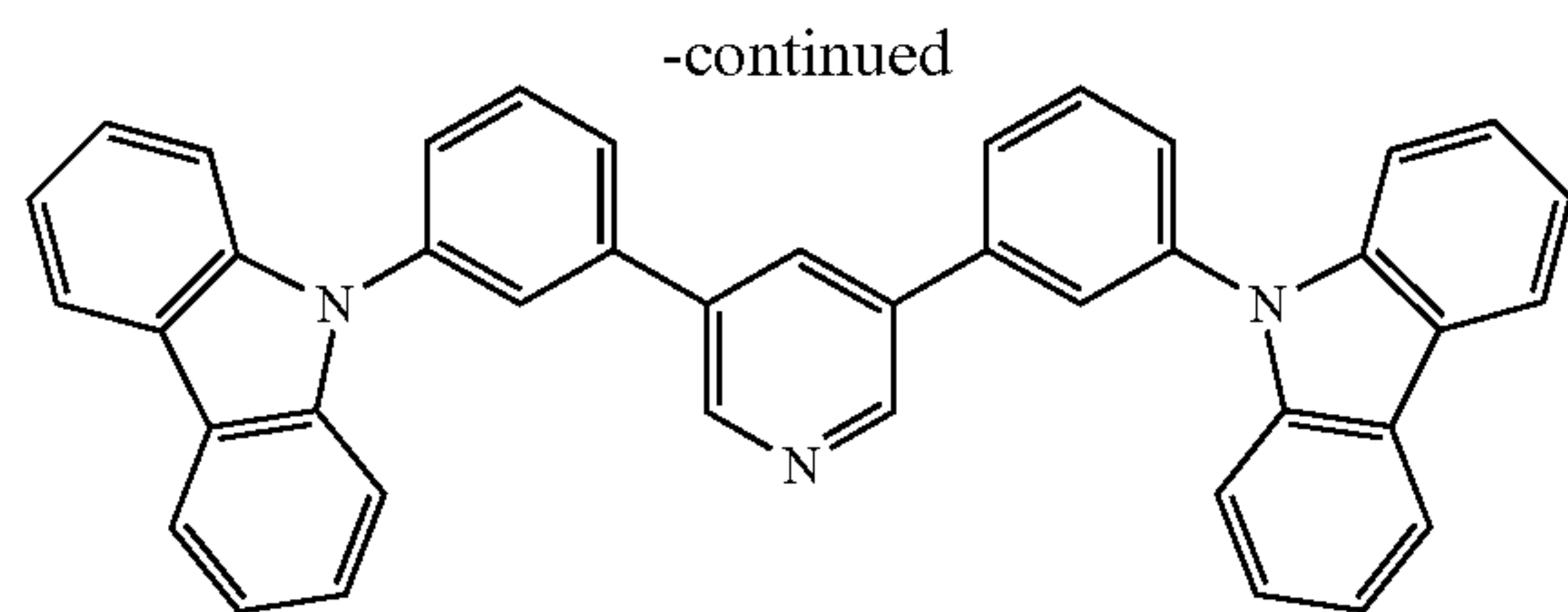
(viii) 35DCzPPy
