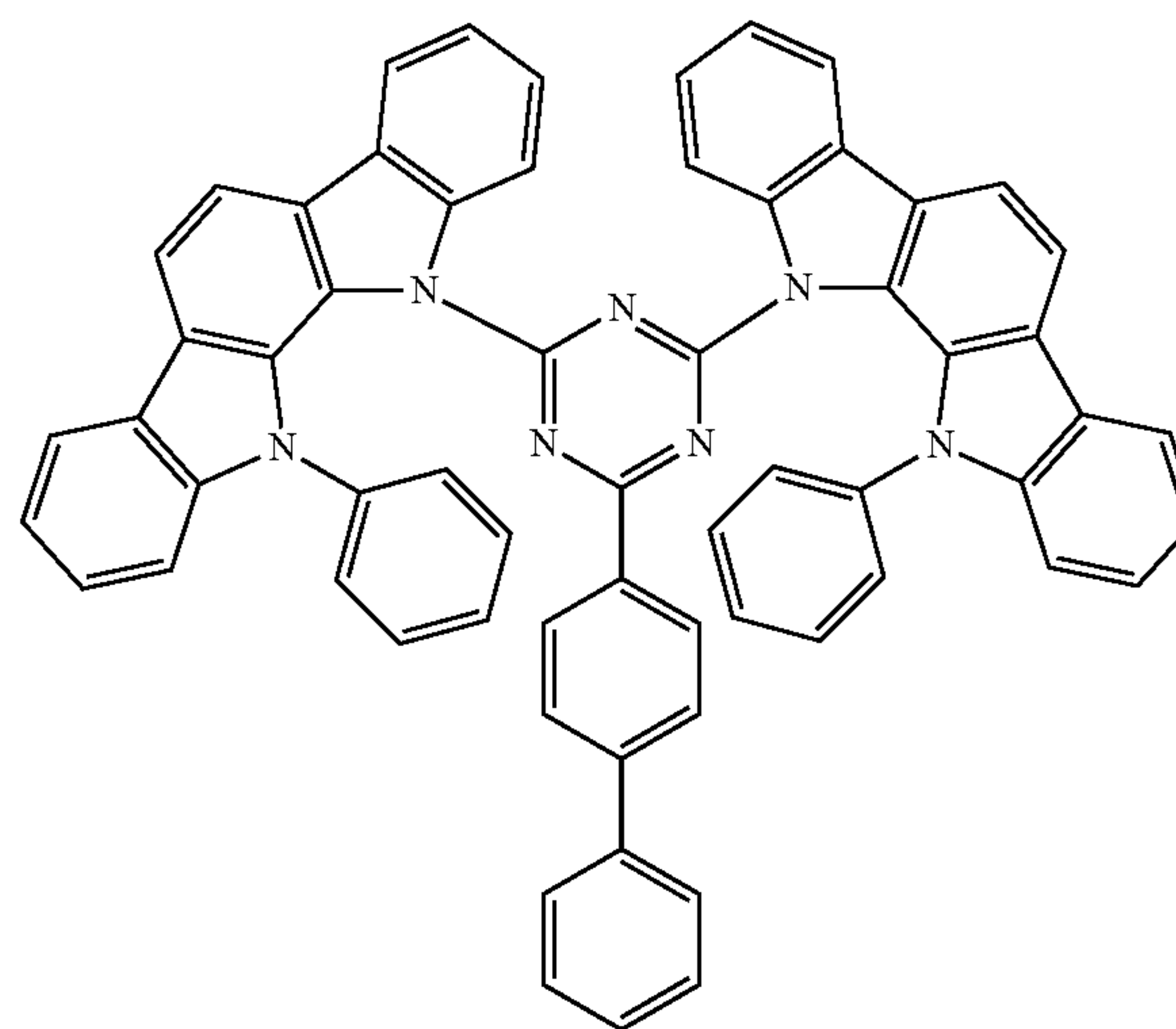
PIC-TRZ
