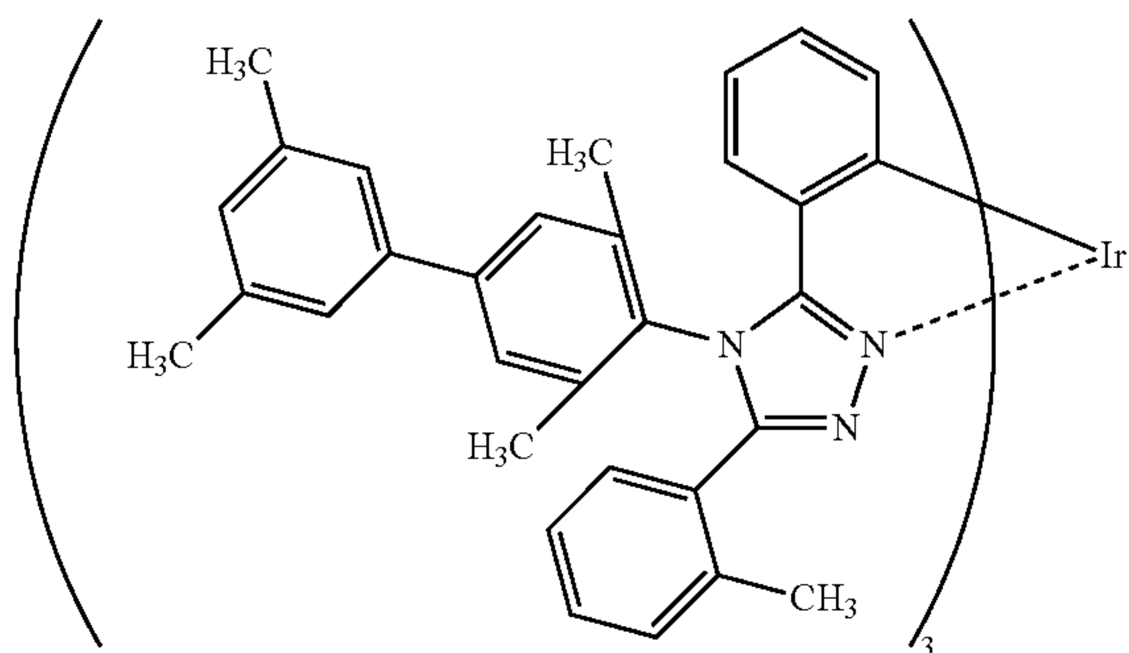
(ix) Ir(mpptz-tetmb) 3
