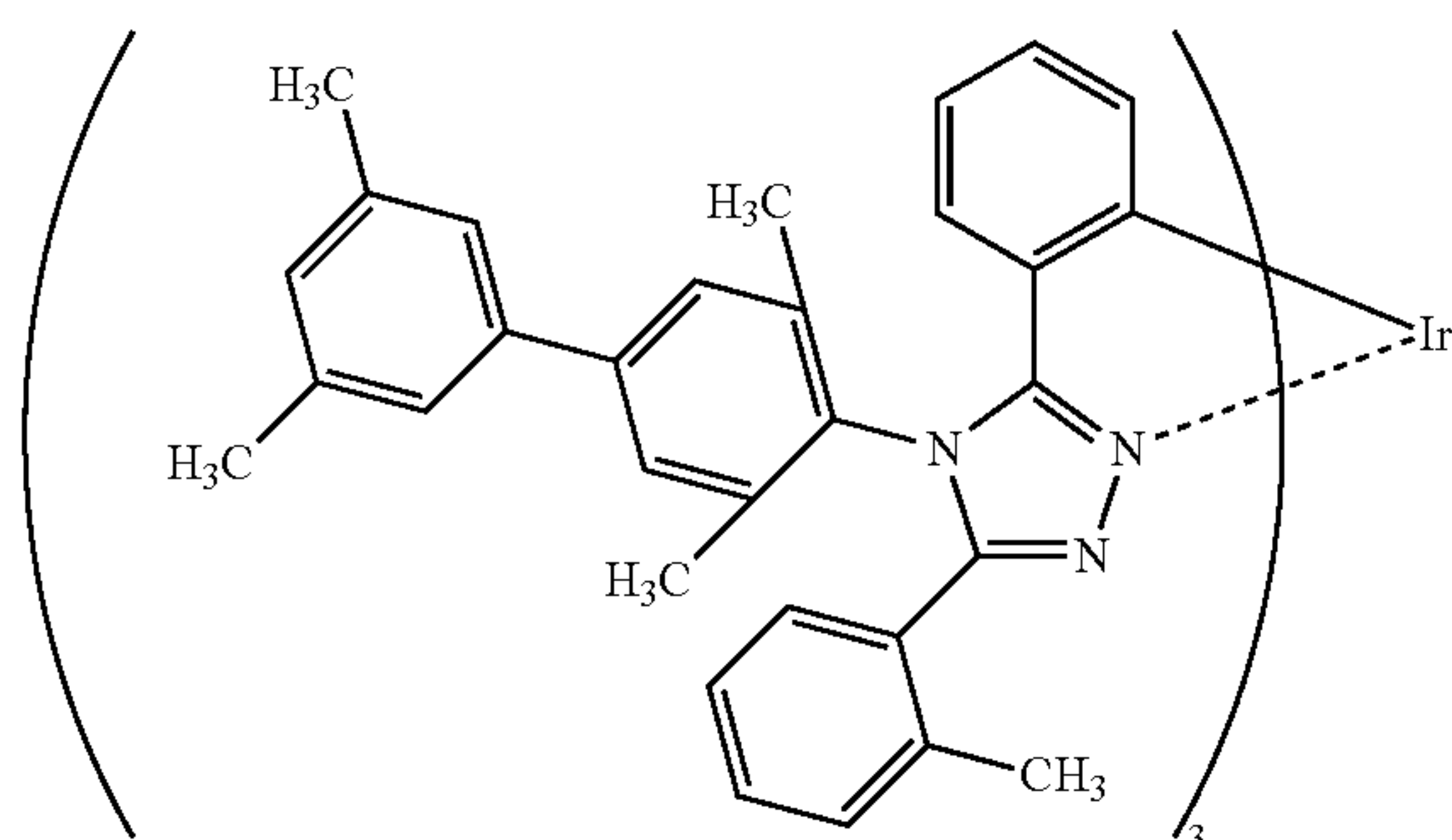
(100) Ir(mpptz-tetmb) 3
