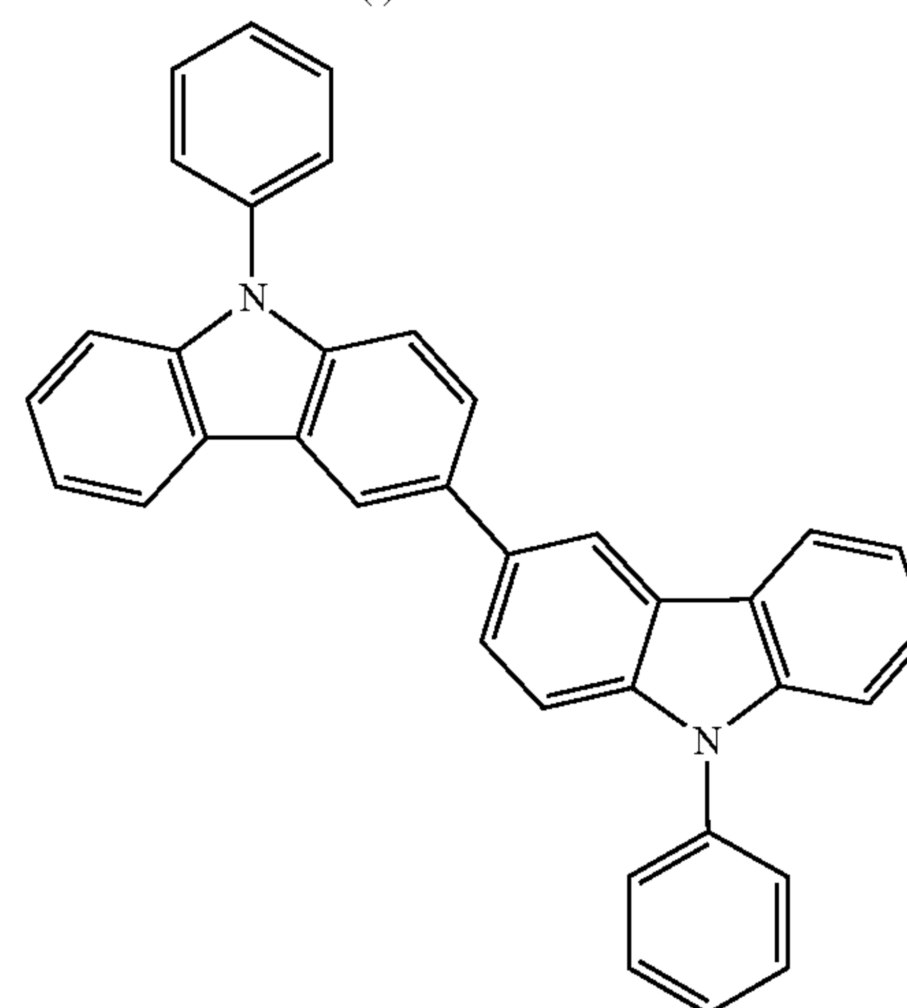
(vii) PCCP
