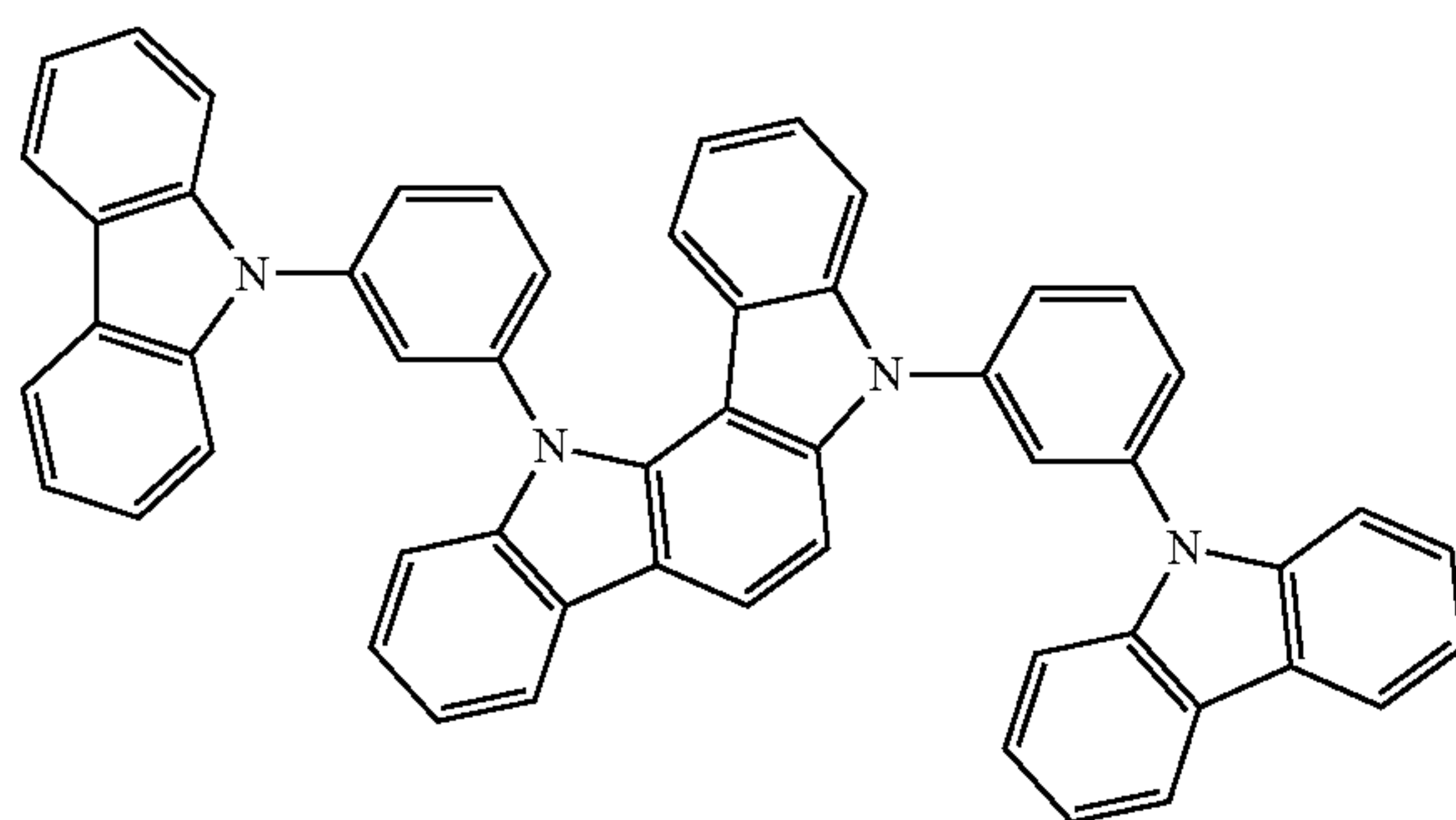
(iii) mCzPICz
