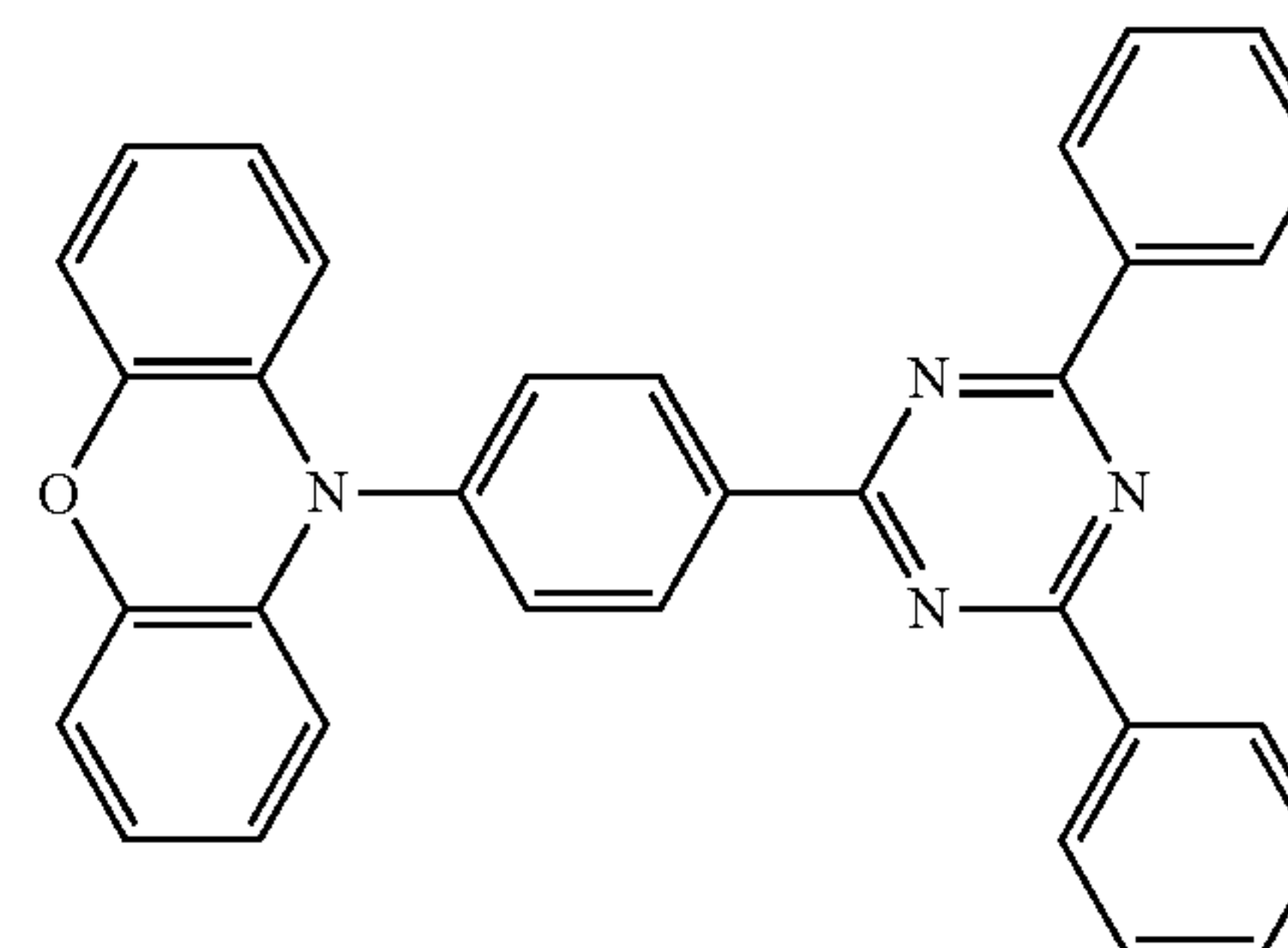
PXZ-TRZ
