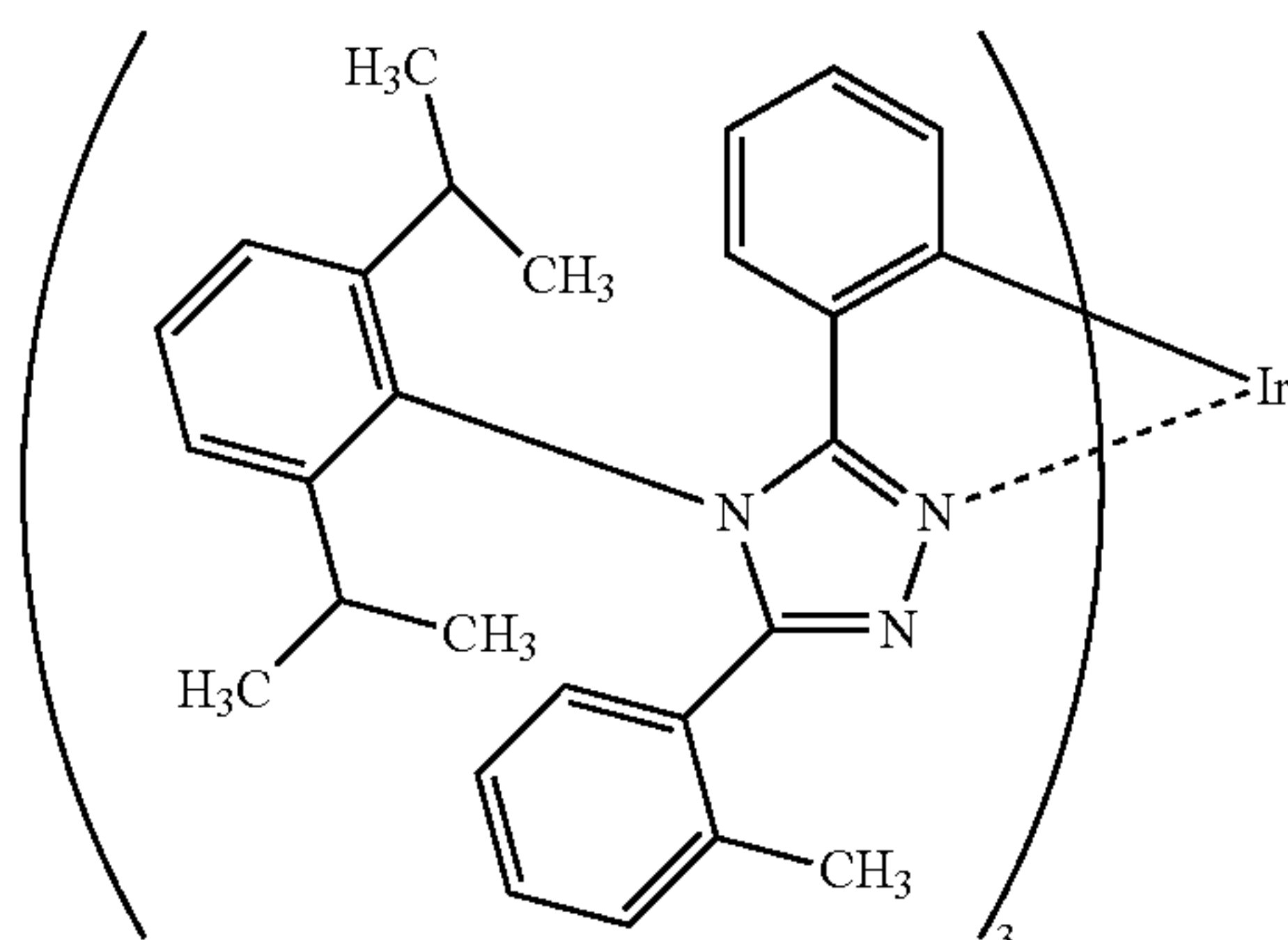
(xi) Ir(mpptz-diPrp) 3
