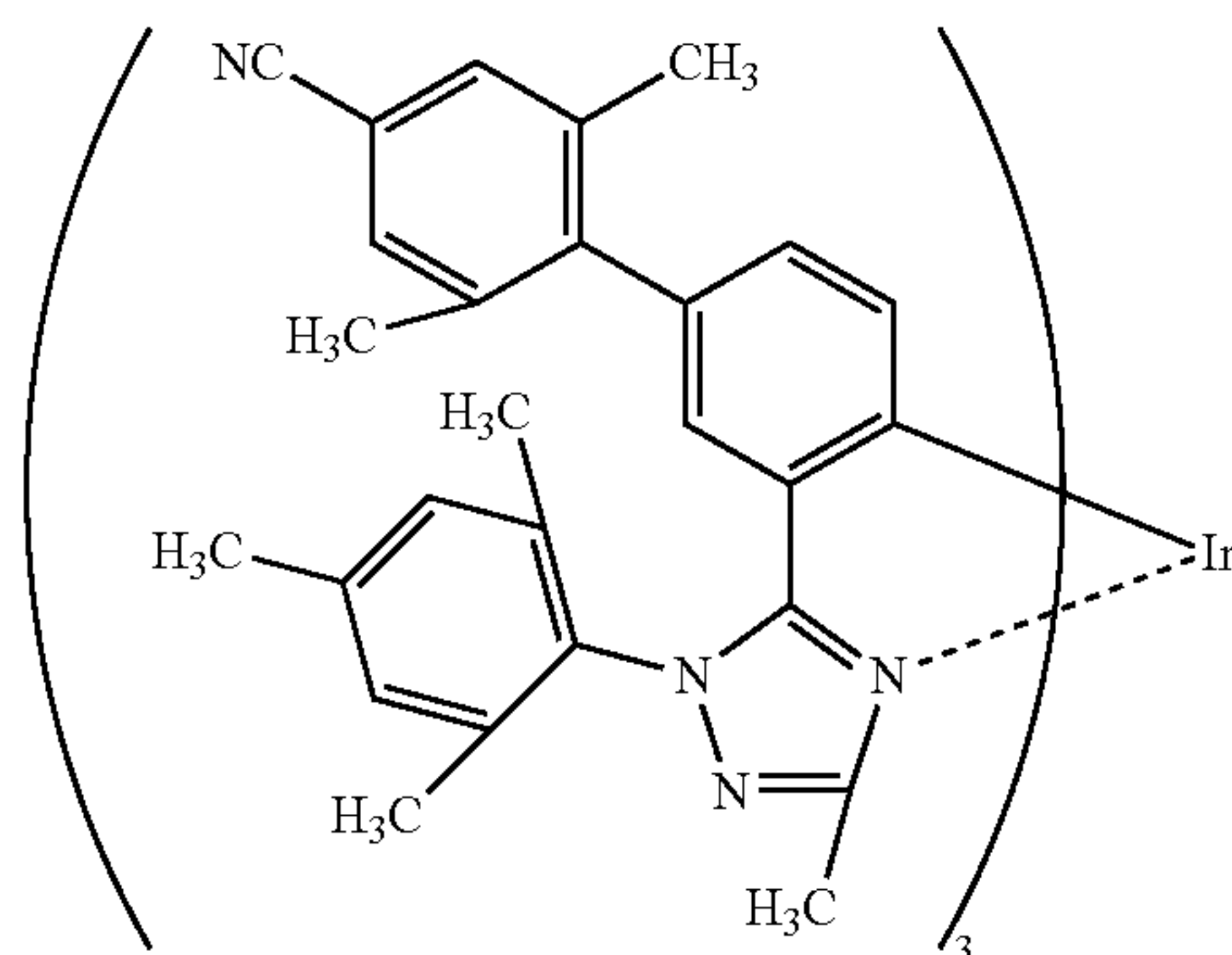
(v) Ir(MdmCN5btz1-tmp) 3
