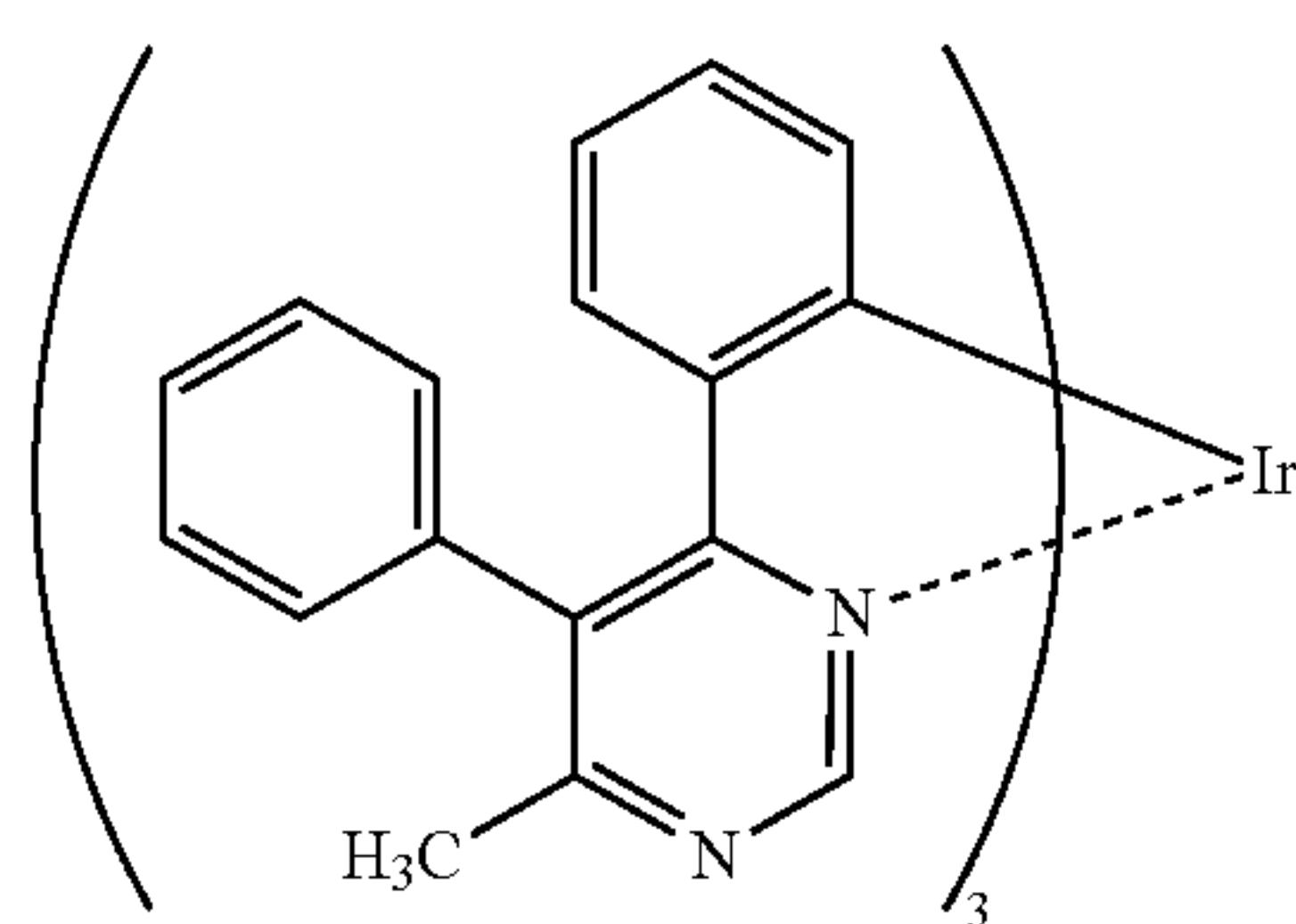
(101) Ir(mpppm) 3
