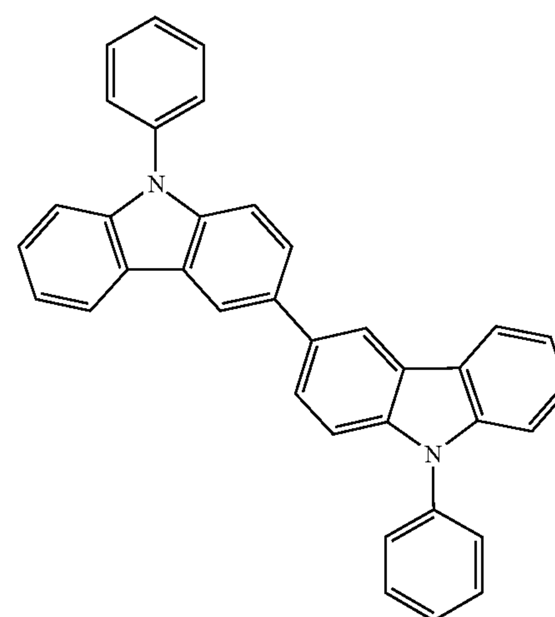
(vii) PCCP
