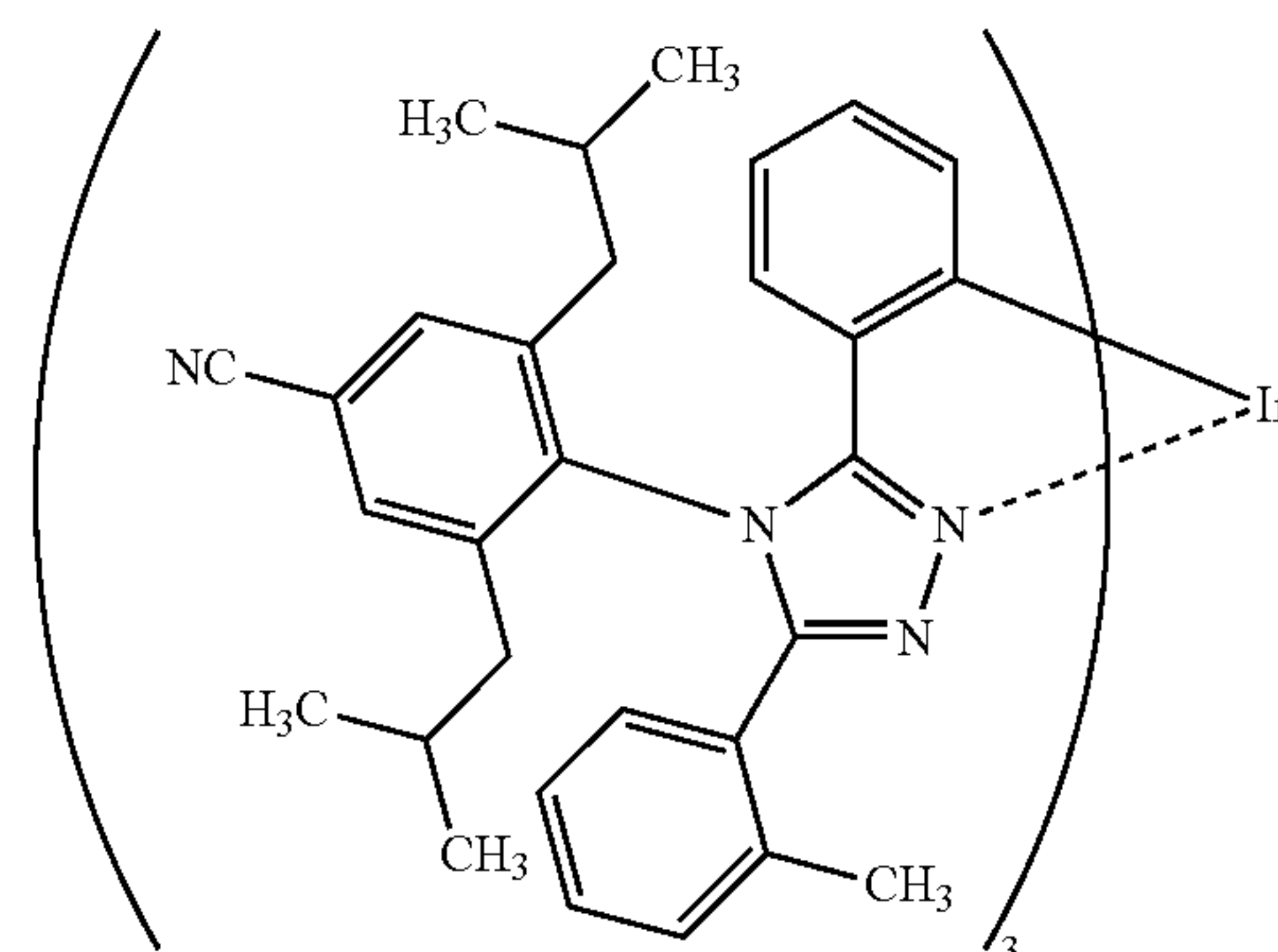
(104) Ir(mpptz-diBuCNp) 3
