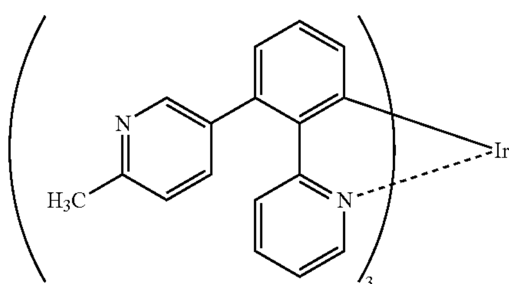
(xii) Ir(mpypy) 3
