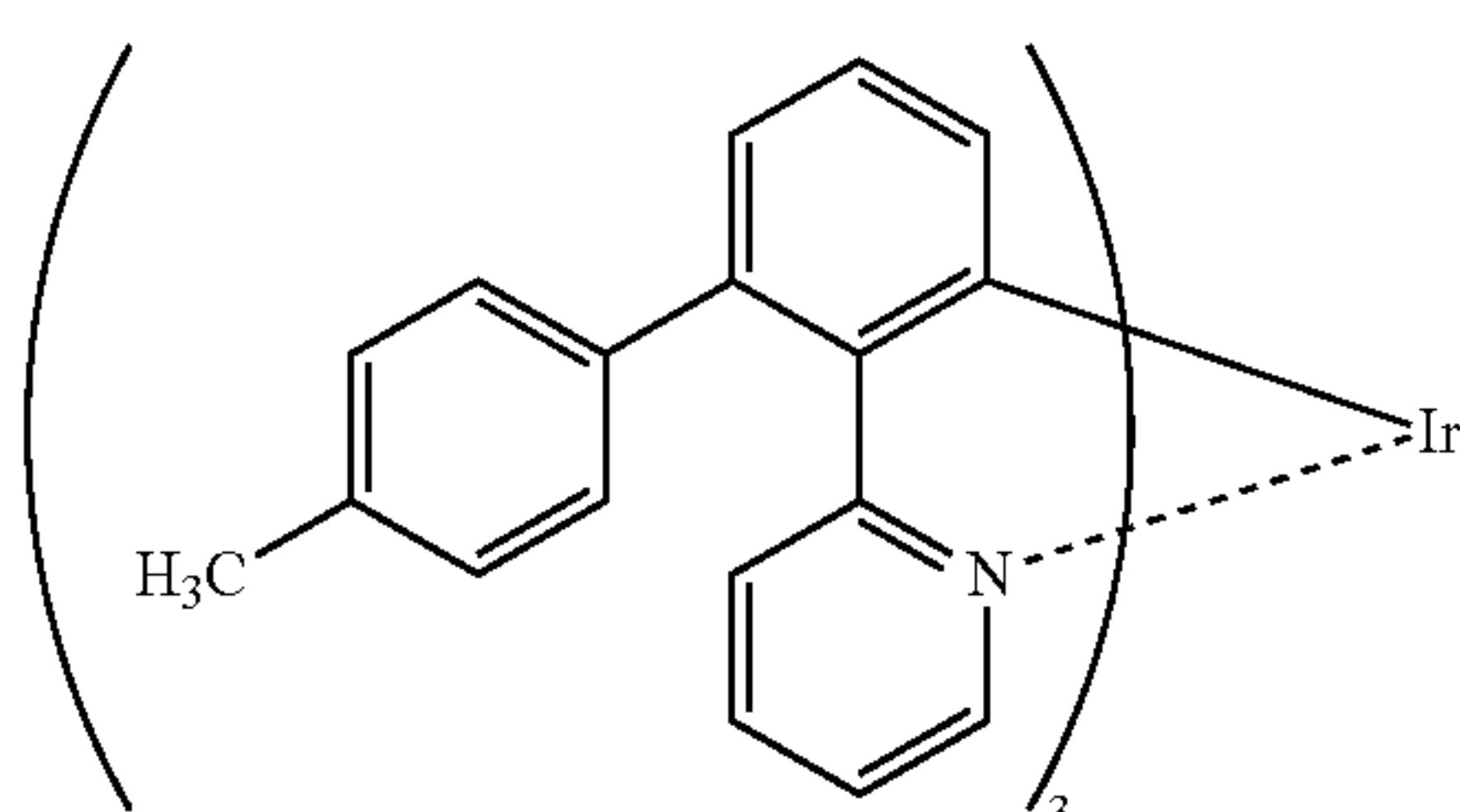
(xiii) Ir(m6bpy) 3
