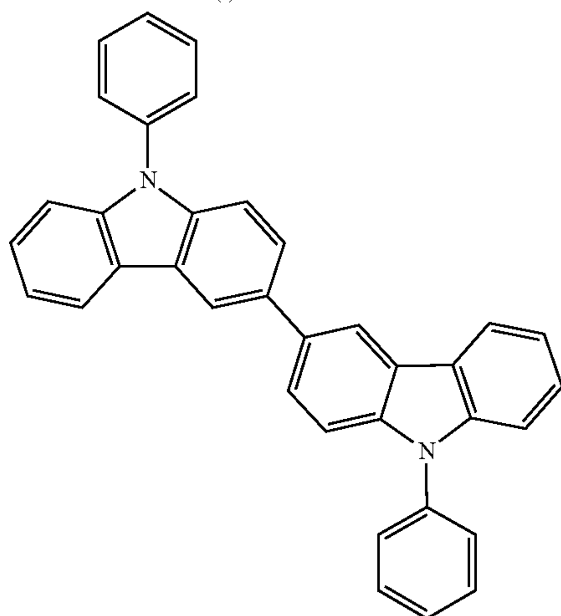
(vii) PCCP
