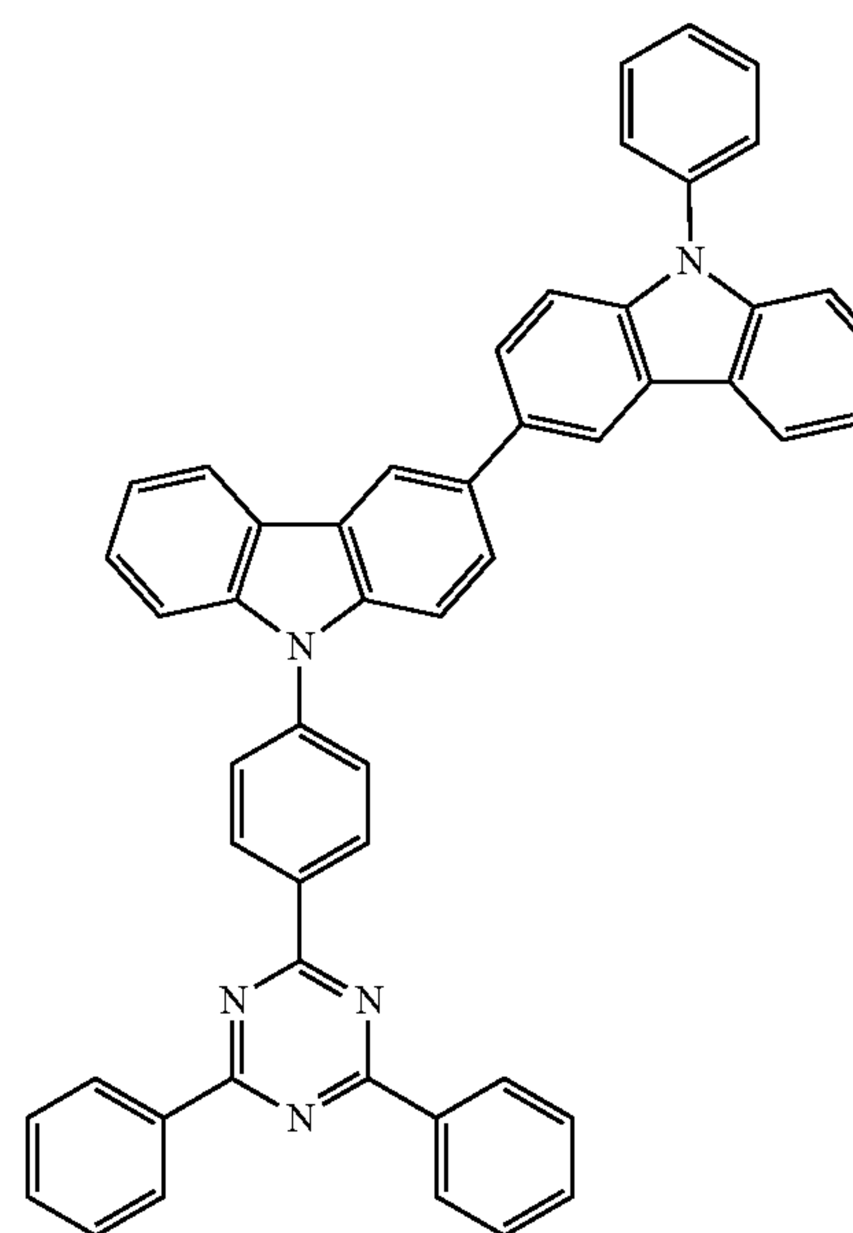
PCCzPTzn
