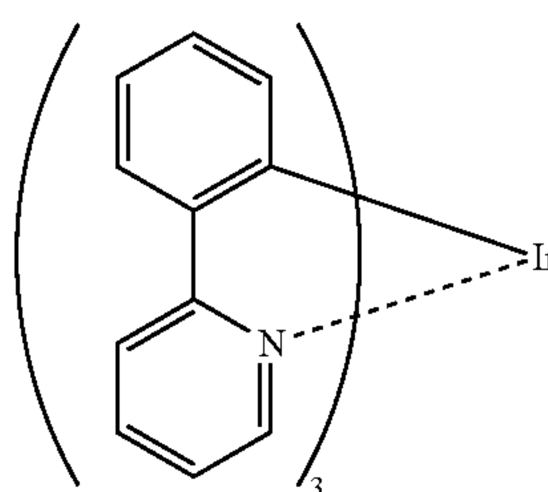
(xiv) [Ir(ppy) 3 ]
