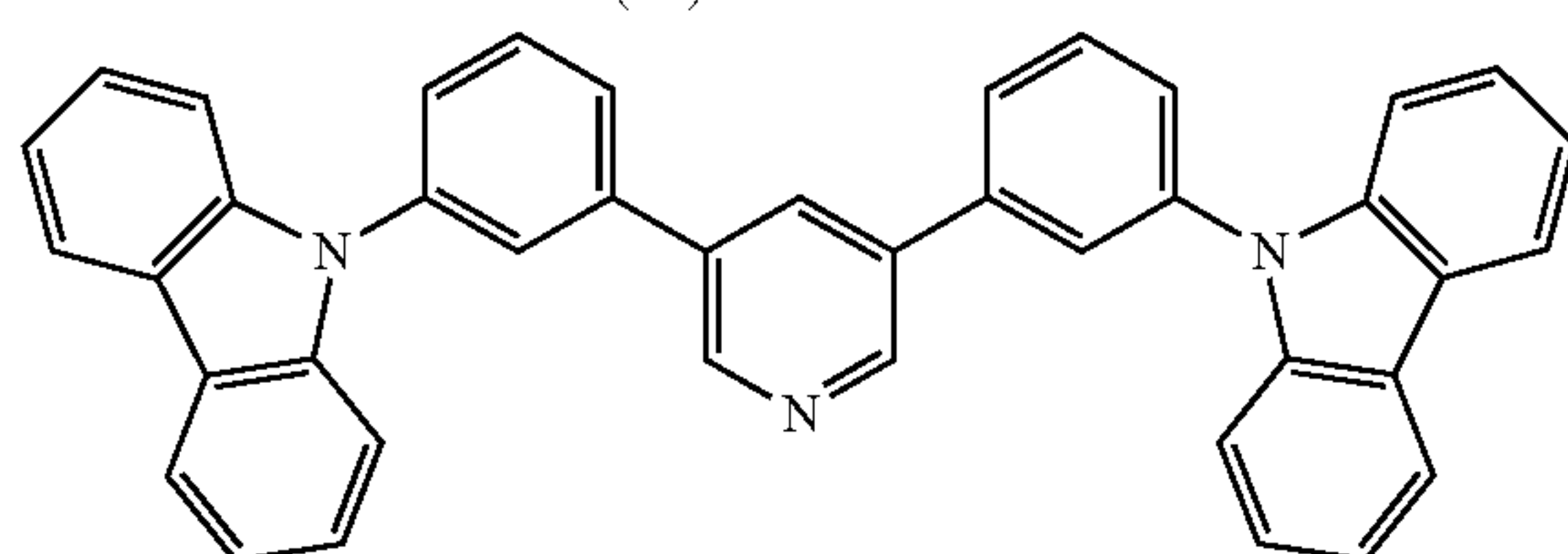
(viii) 35DCzPPy
