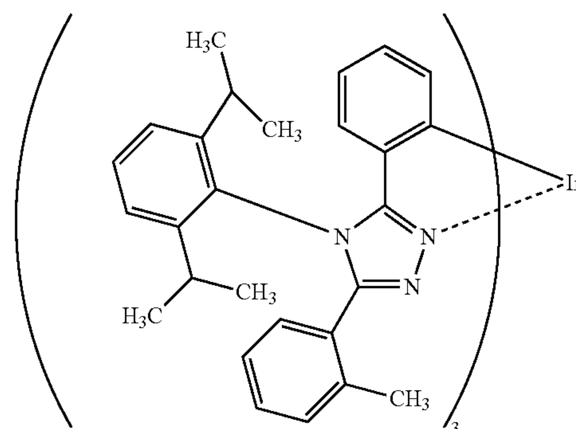
(105) Ir(mpptz-tmp) 3
