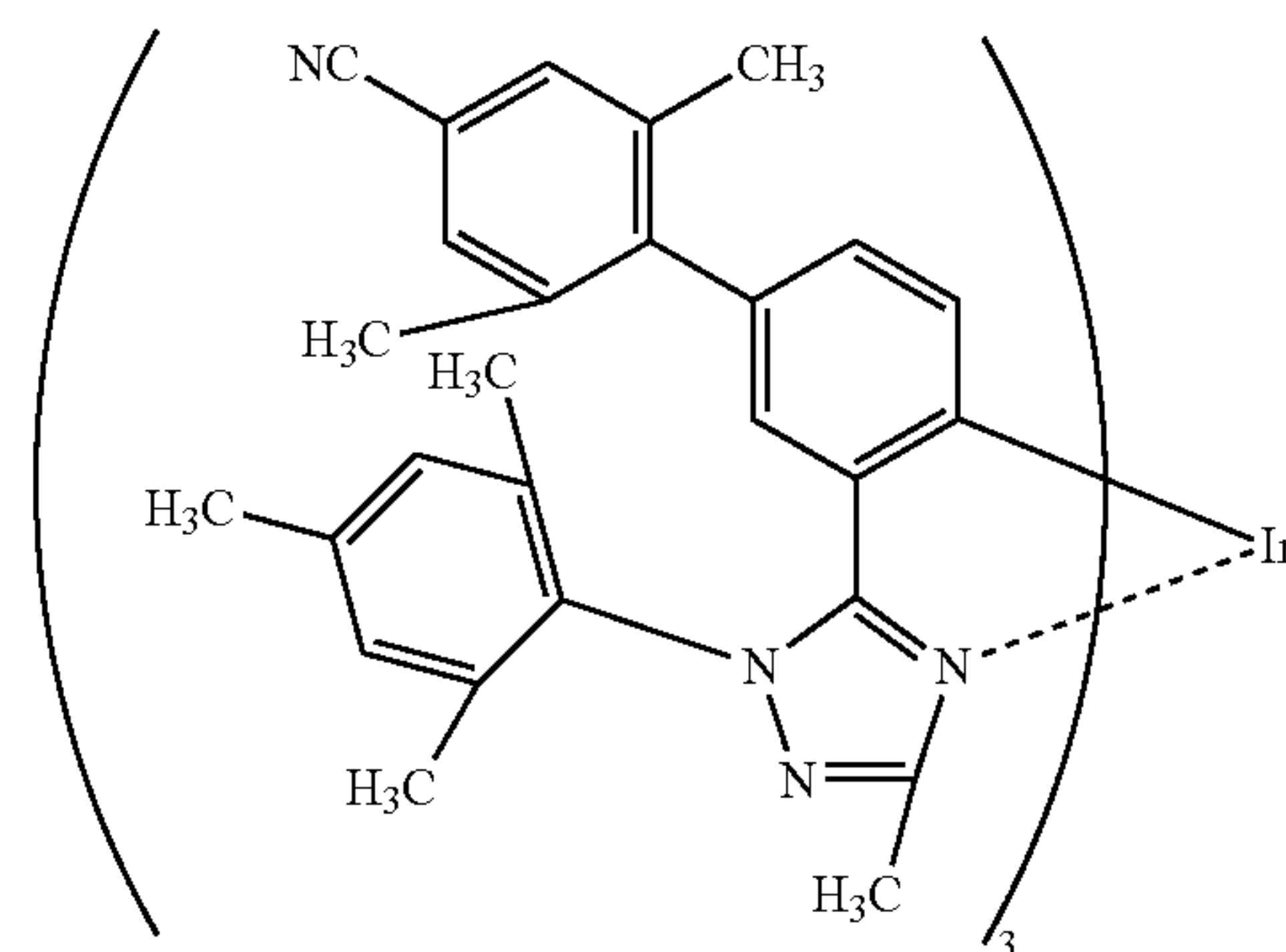
(103) Ir(MdmCN5btz1-tmp) 3
