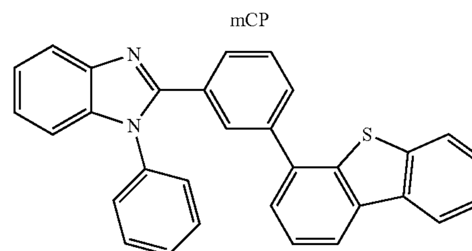
mDBTBlm-II
