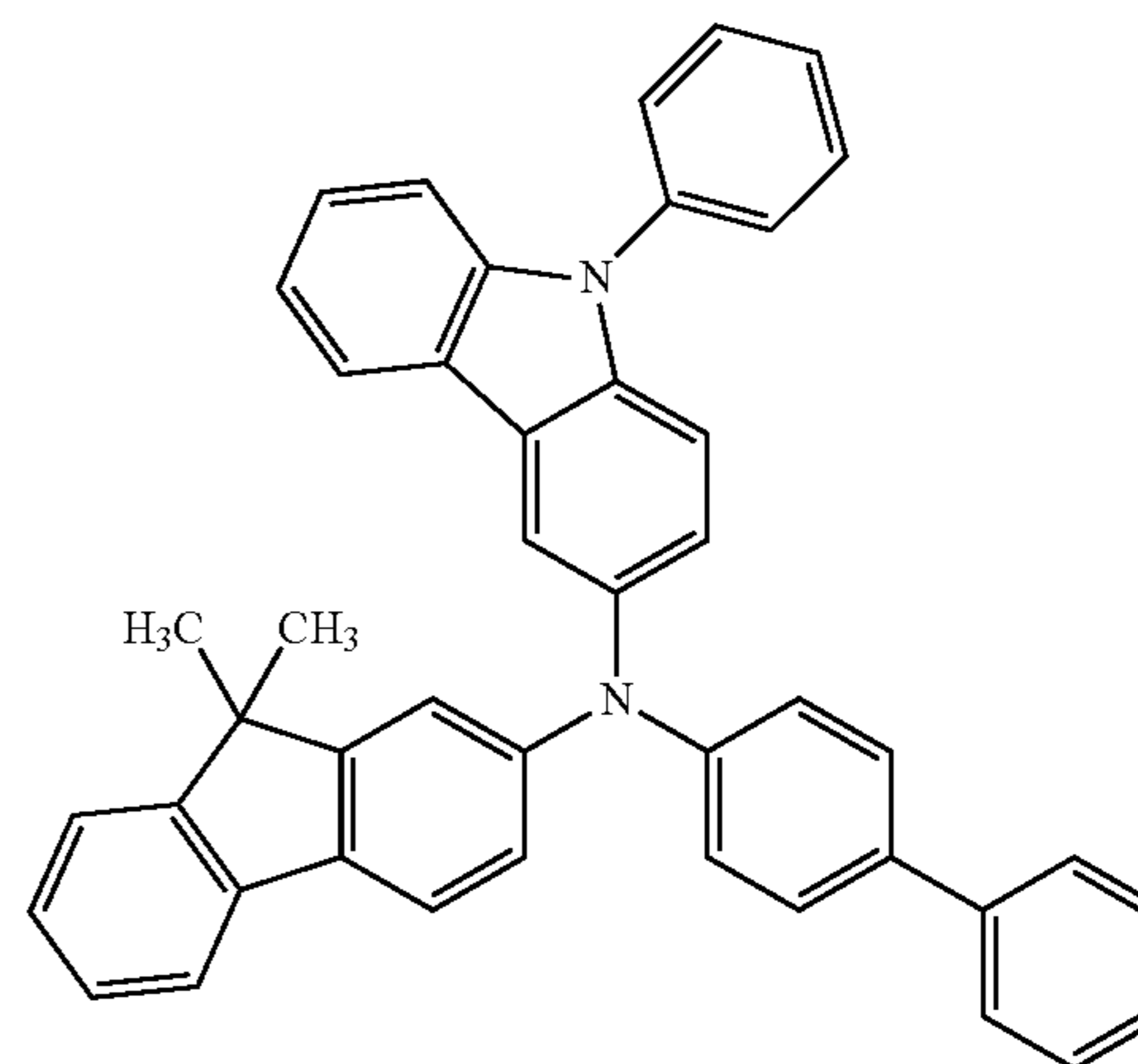
PCBiF
