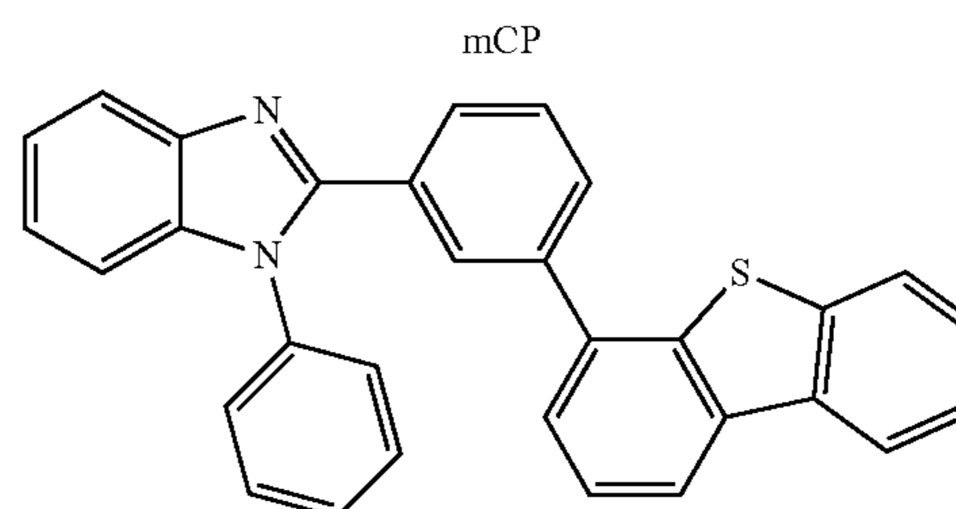
mDBTBlm-II
