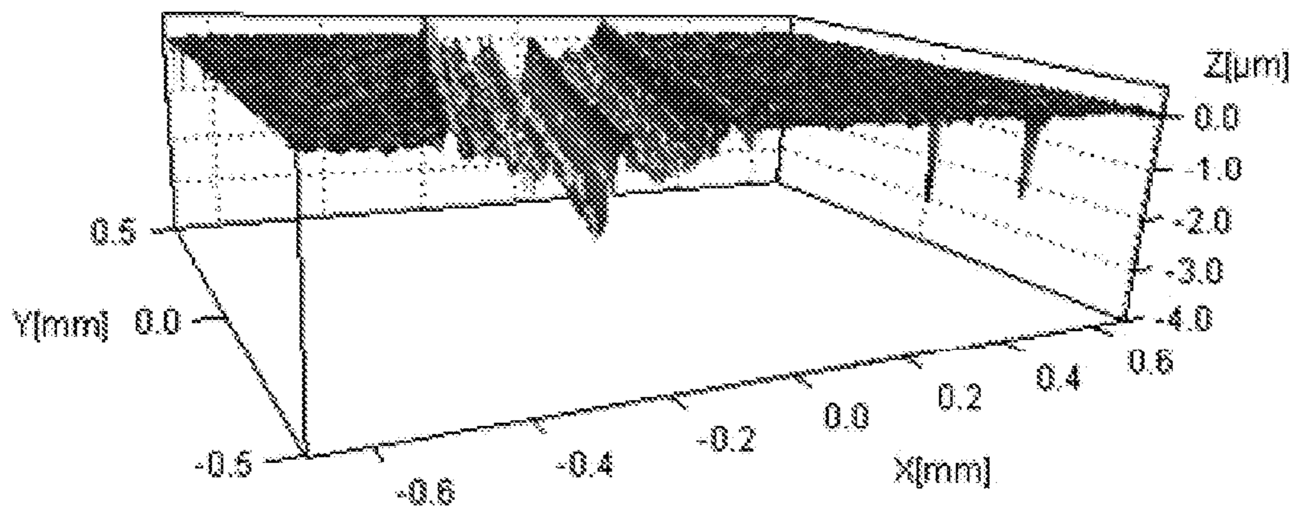
PAO4+2.5wt% CPCa
