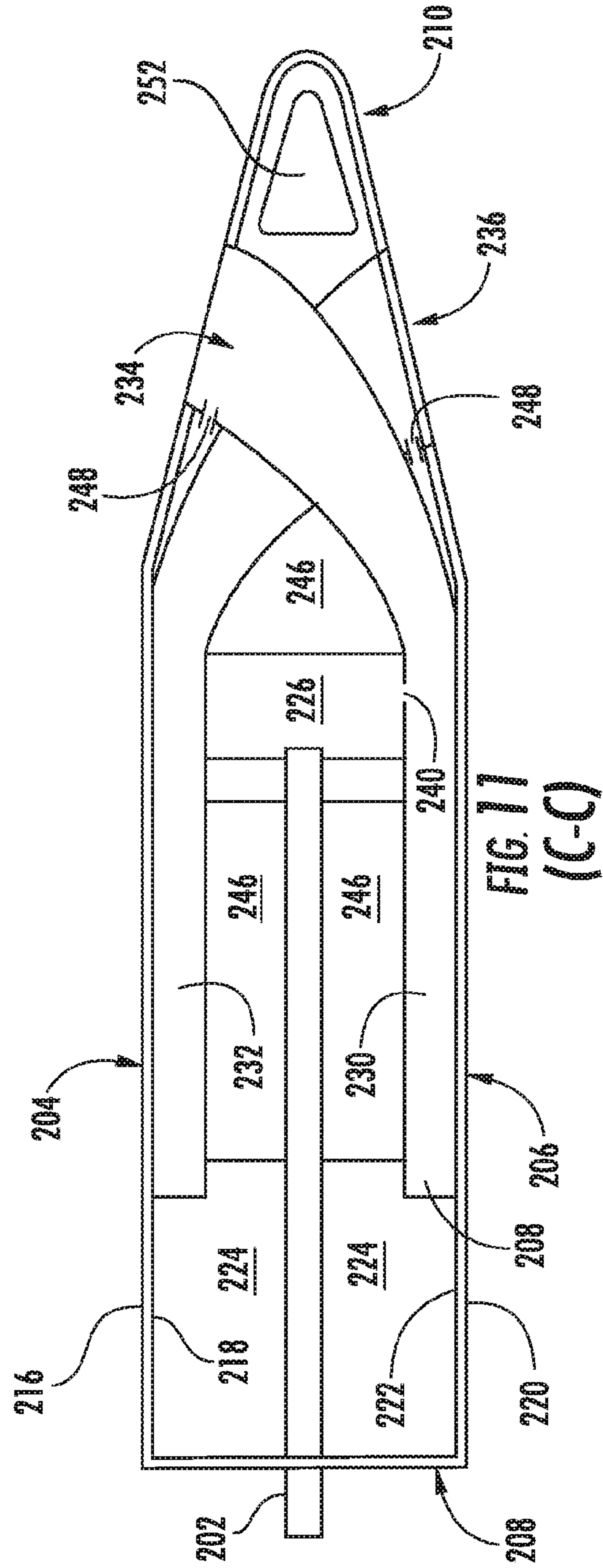
FIG. 10 (B-B)
