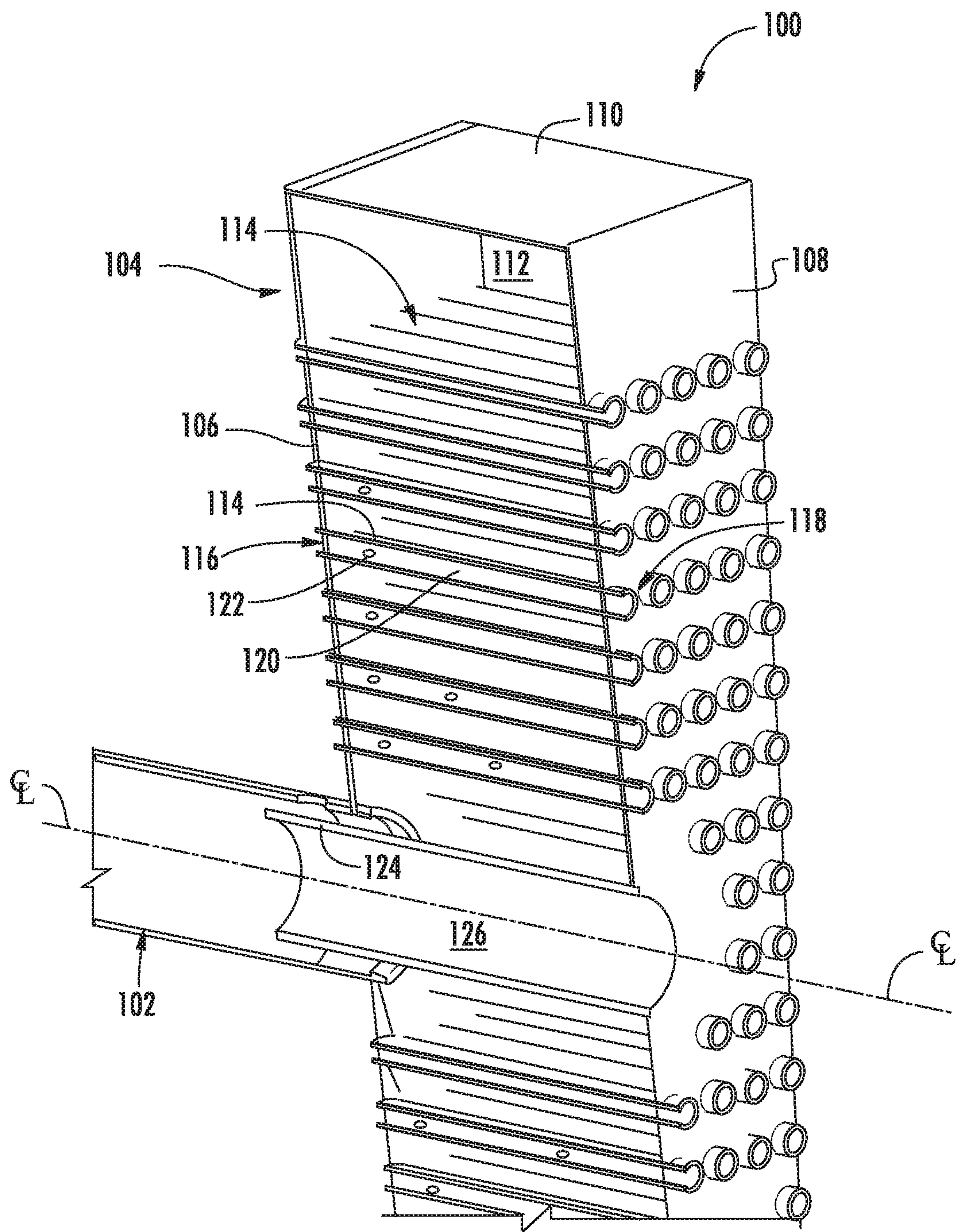
FIG. 6 (A-A)
