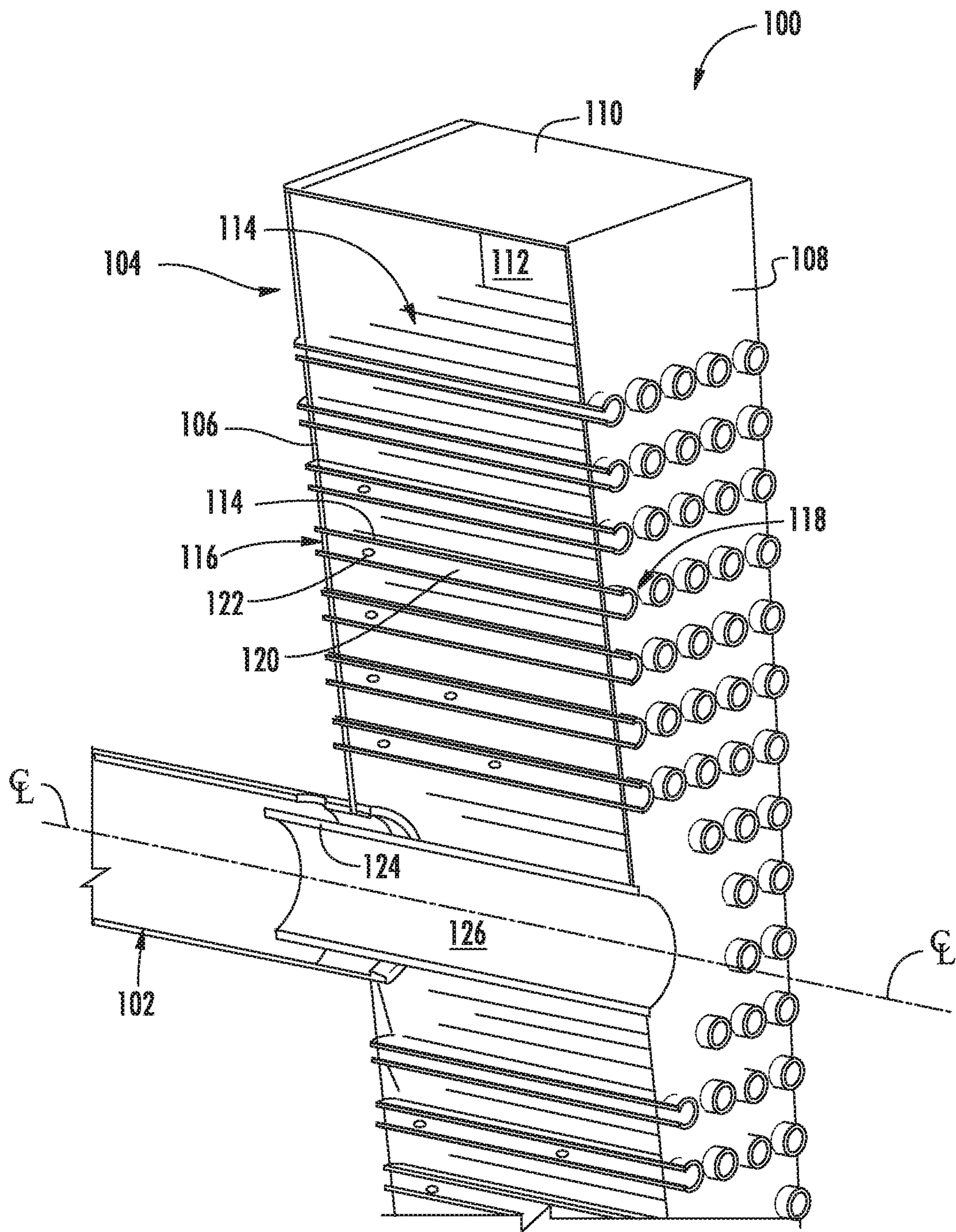
FIG. 6 (A-A)
