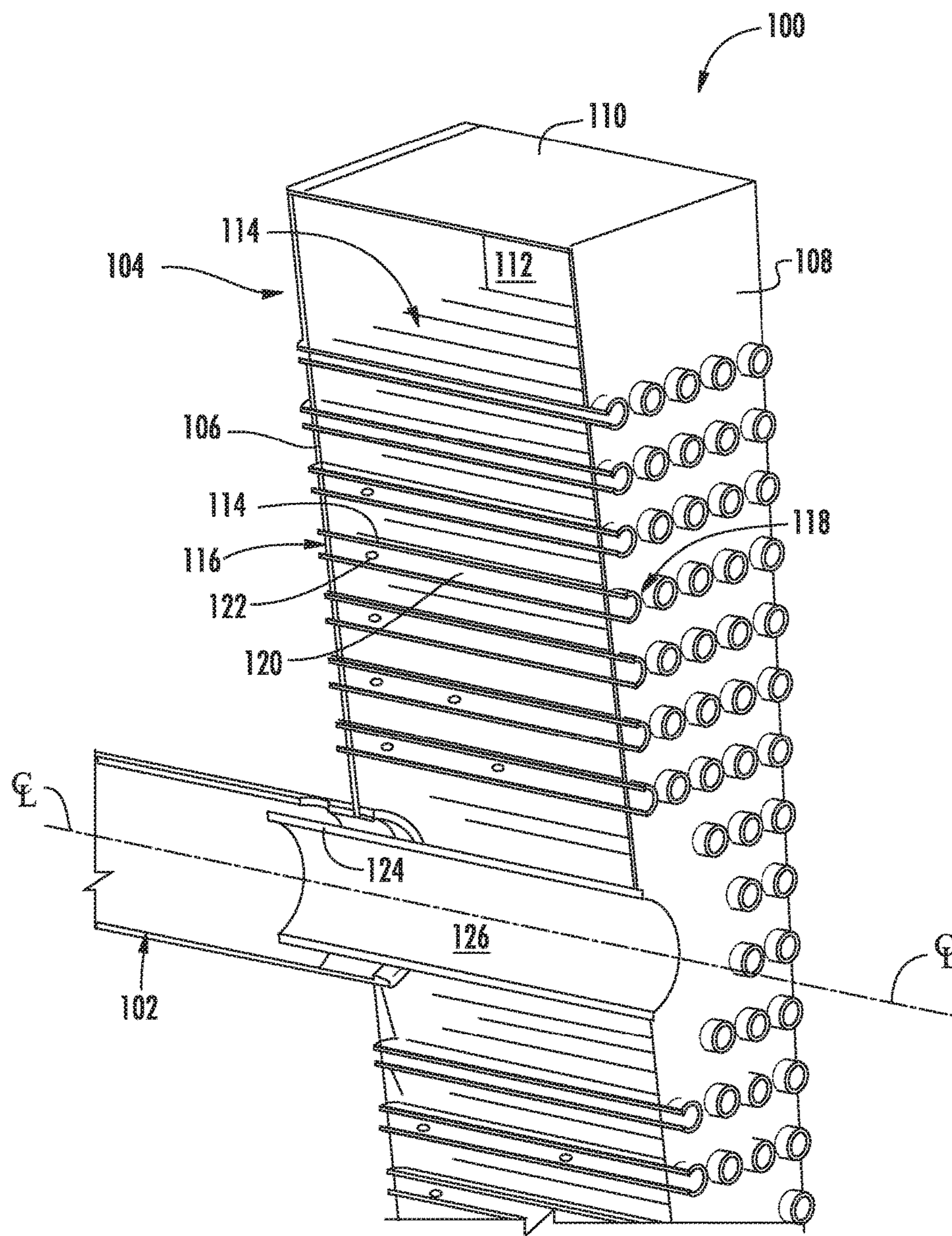
FIG. 6 (A-A)
