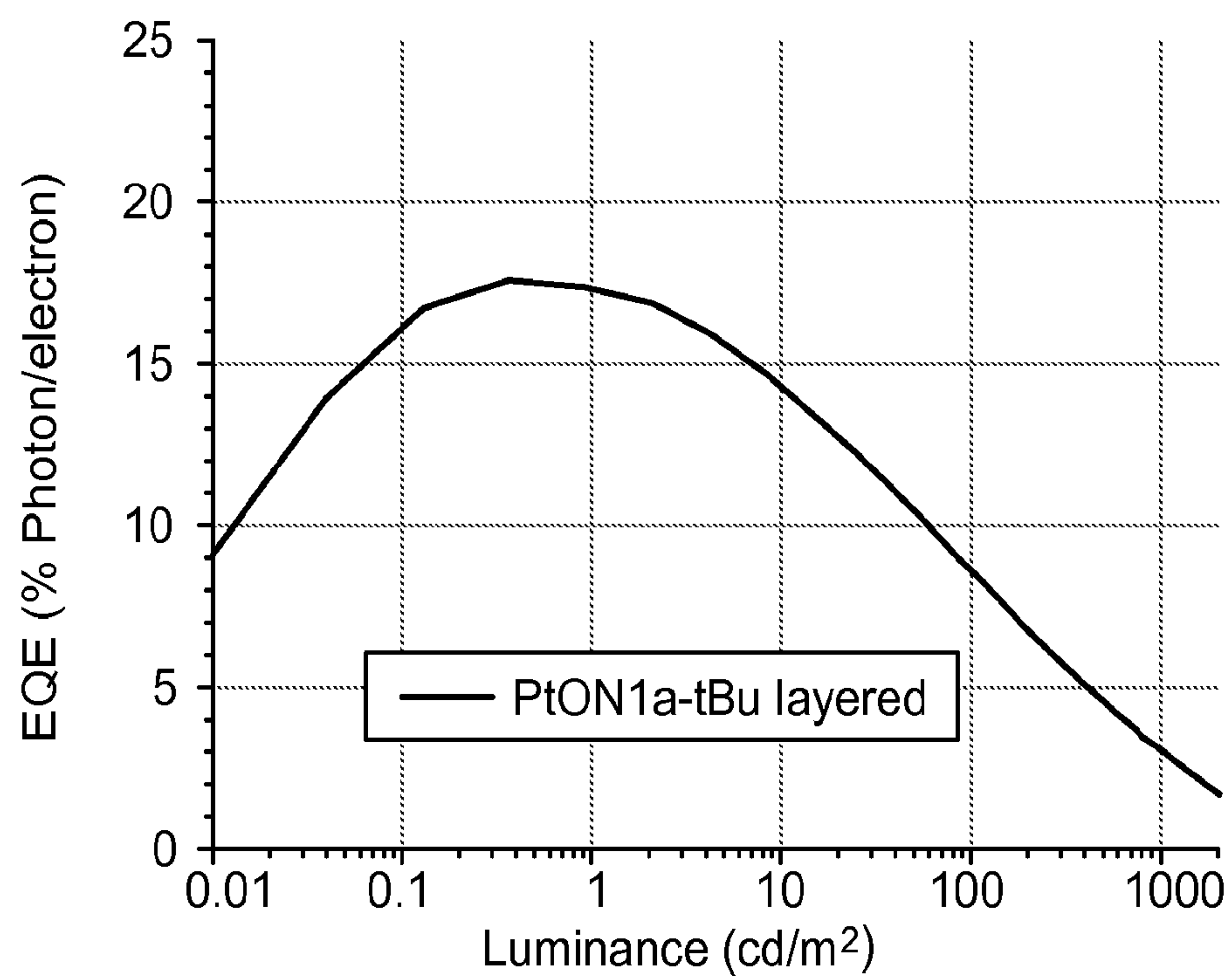
FIG. 7A
