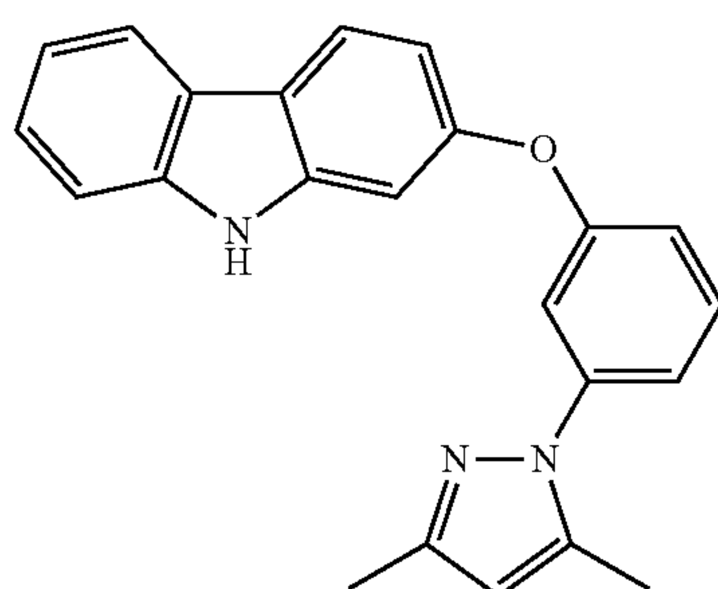
2-[3-(3,5-Dimethylpyrazol-1-yl)-phenoxy]- carbazole
