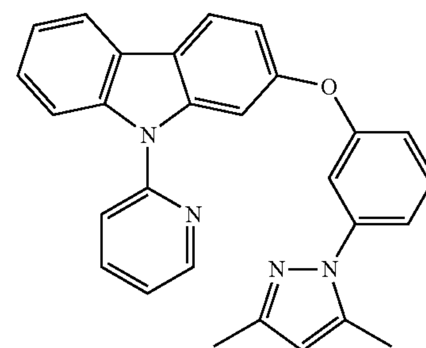
2-[3-(3,5-Dimethylpyrazol-1-yl)-phenoxy]- 9-pyridin-2-ylcarbazole
