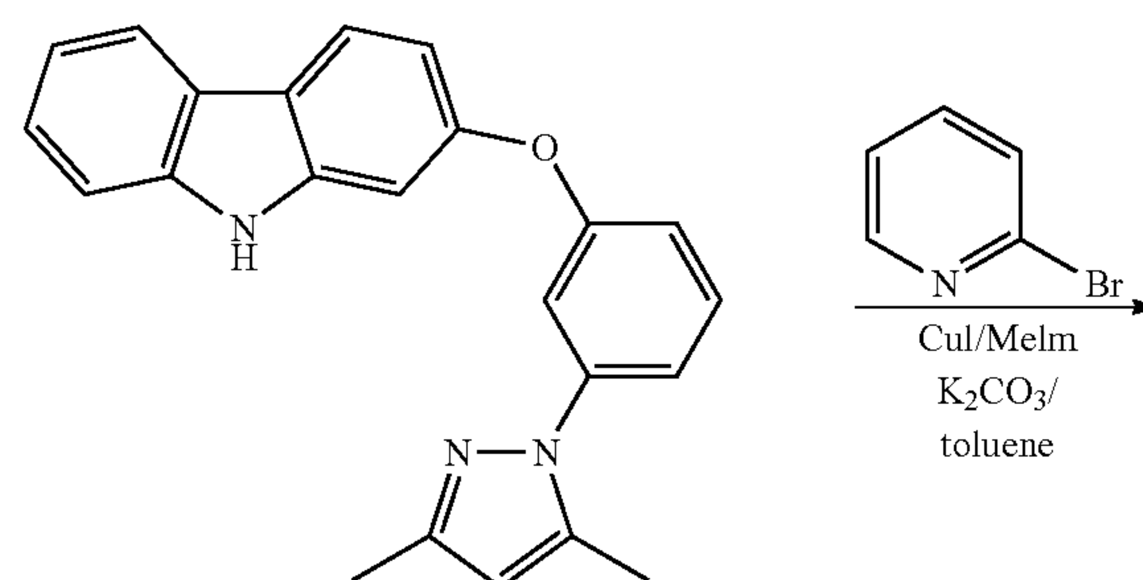
2-[3-(3,5-Dimethylpyrazol-1-yl)-phenoxy]- carbazole
