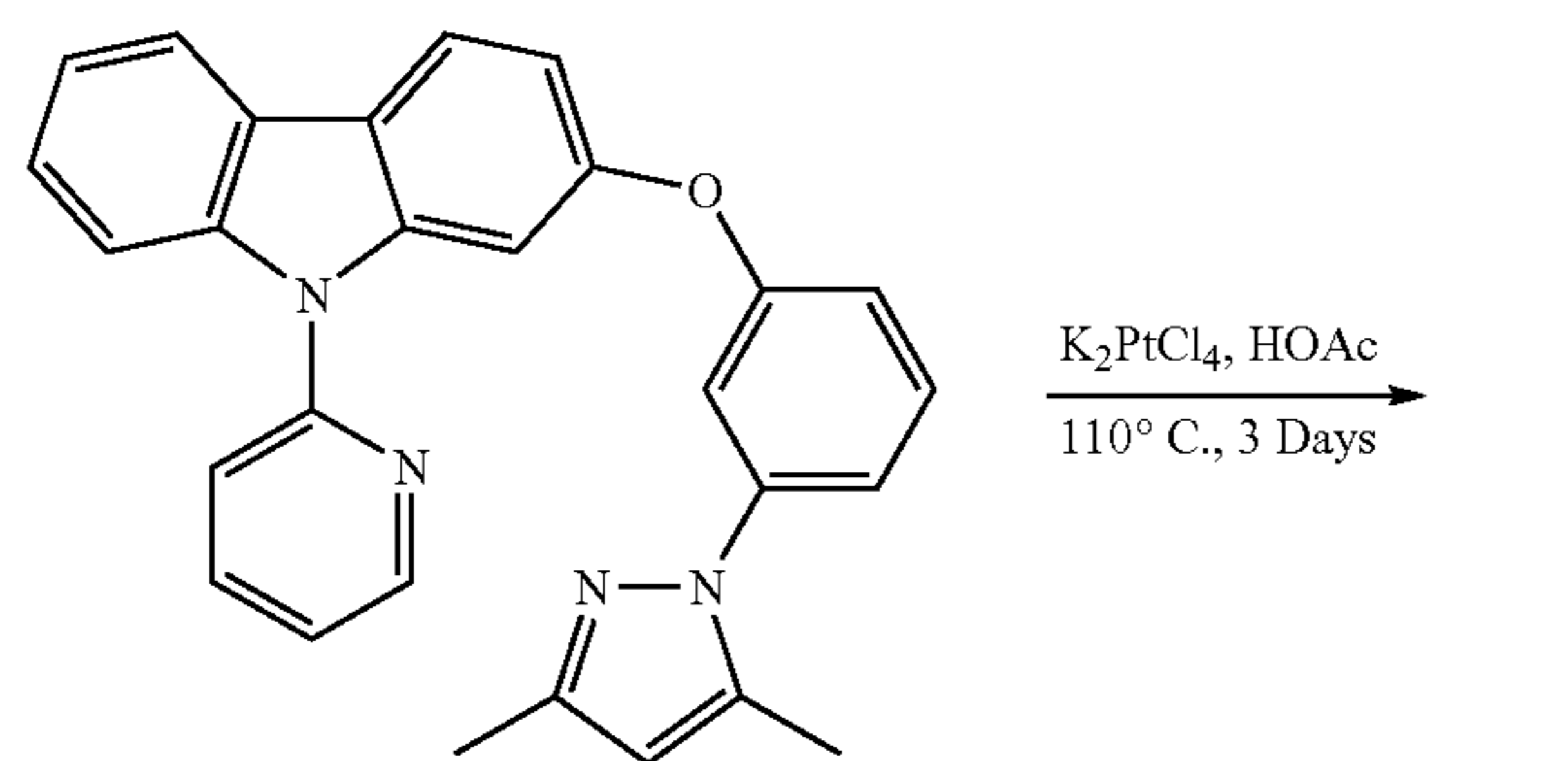
2-[3-(3,5-Dimethylpyrazol-1-yl)-phenoxy]-9-pyridin-2-ylcarbazole
