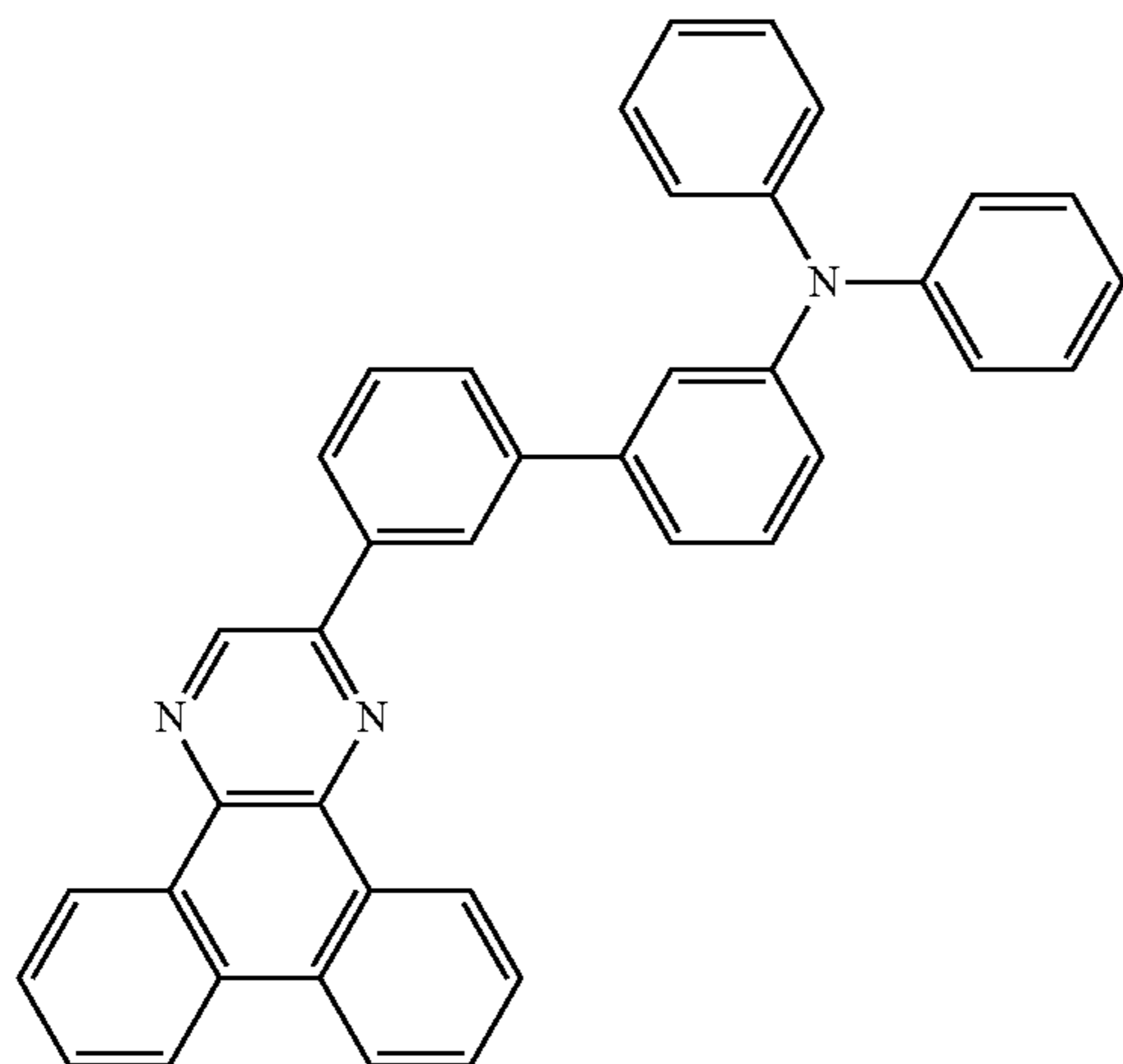
2mDPhABPDBq
