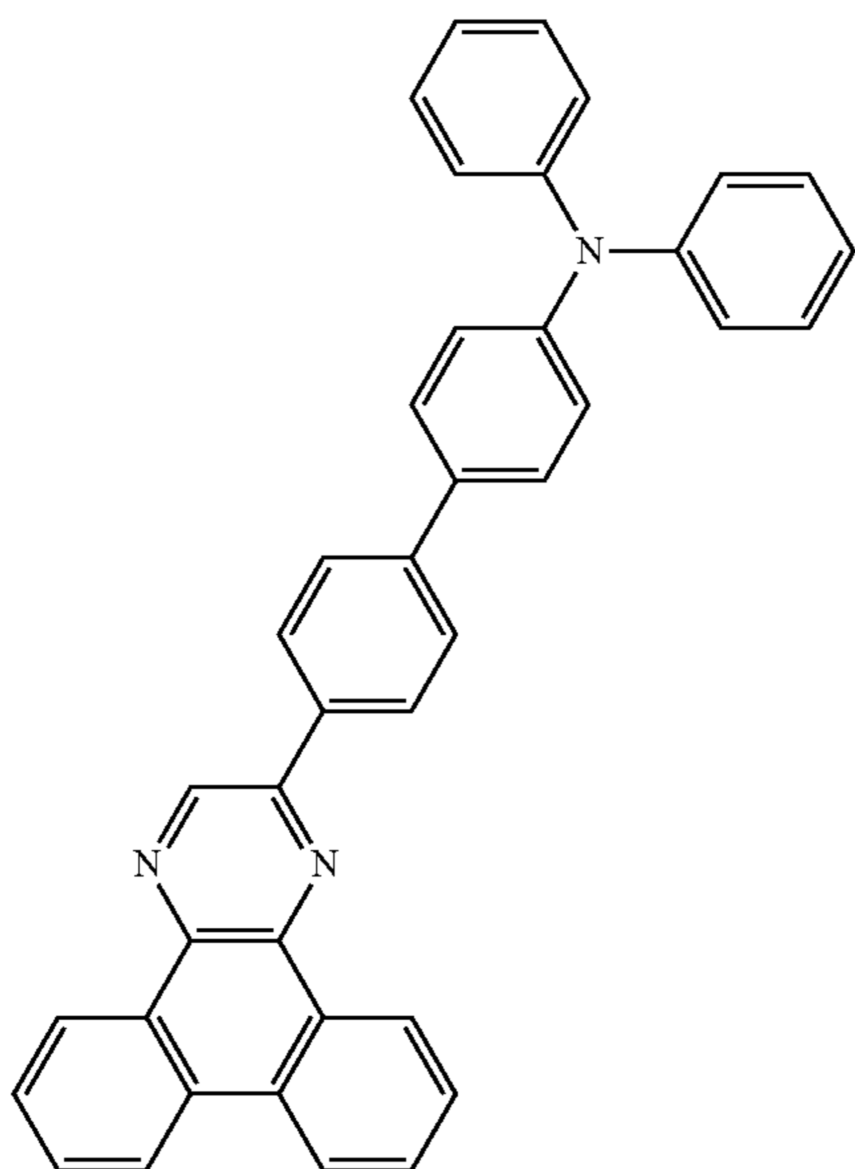
2DPhABPDBq
