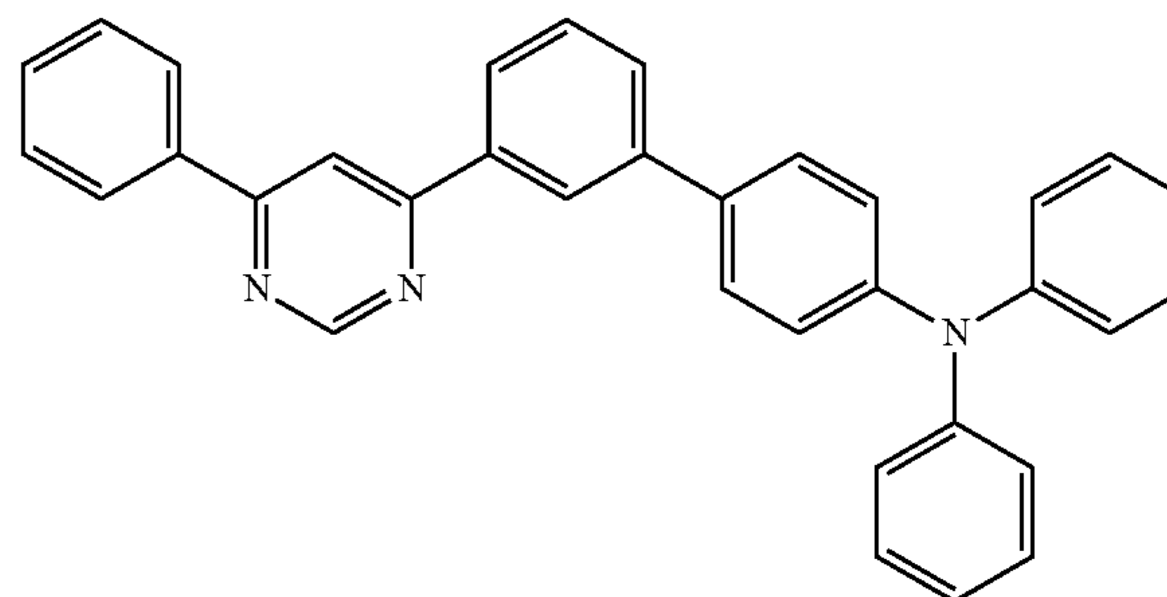
4mpDPhABPPm
