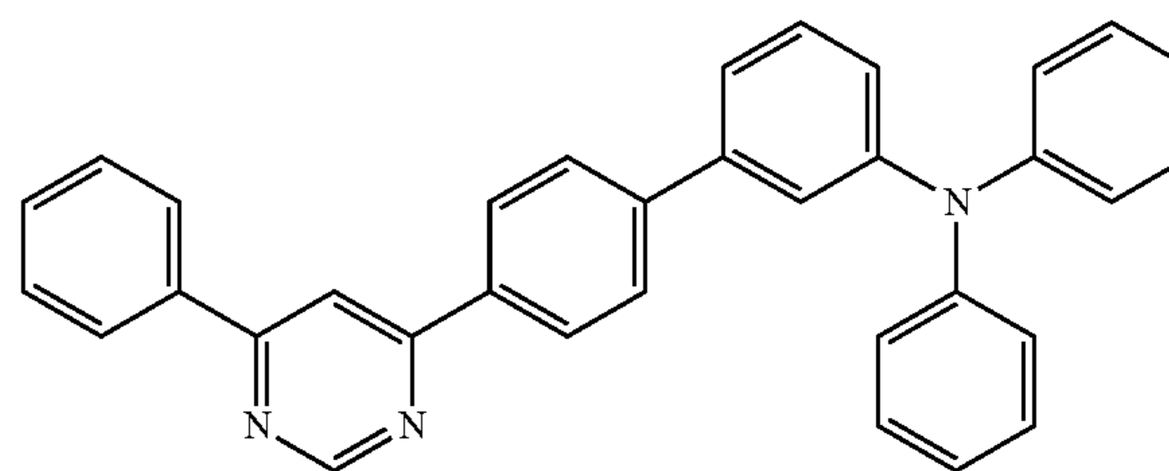
4pmDPhABPPm
