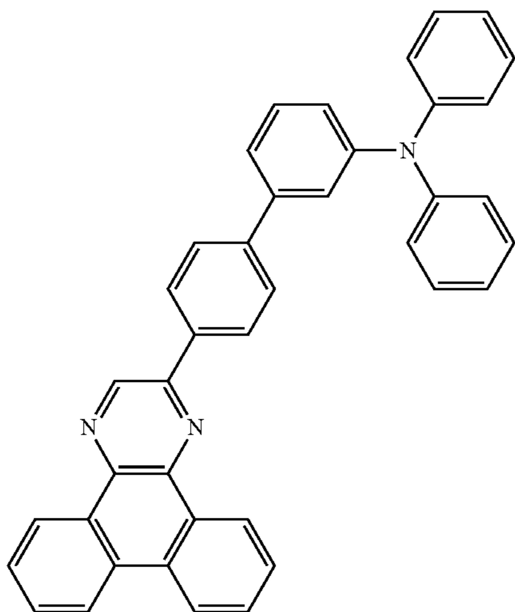
2pmDPhABPDBq
