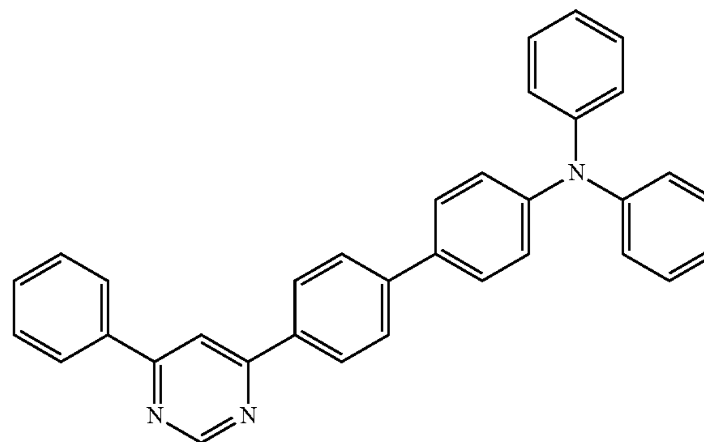
4DPhABPPm
