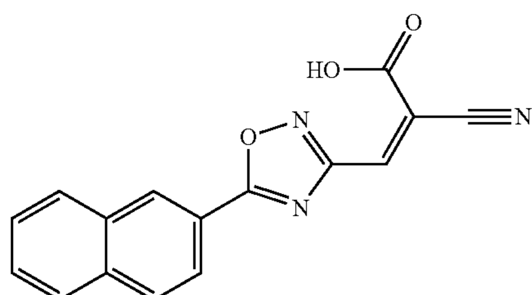
(Z)-2-cyano-3-(5-naphthalen-2-yl)-1,2,4-oxadiazol-3-yl)acrylic acid
