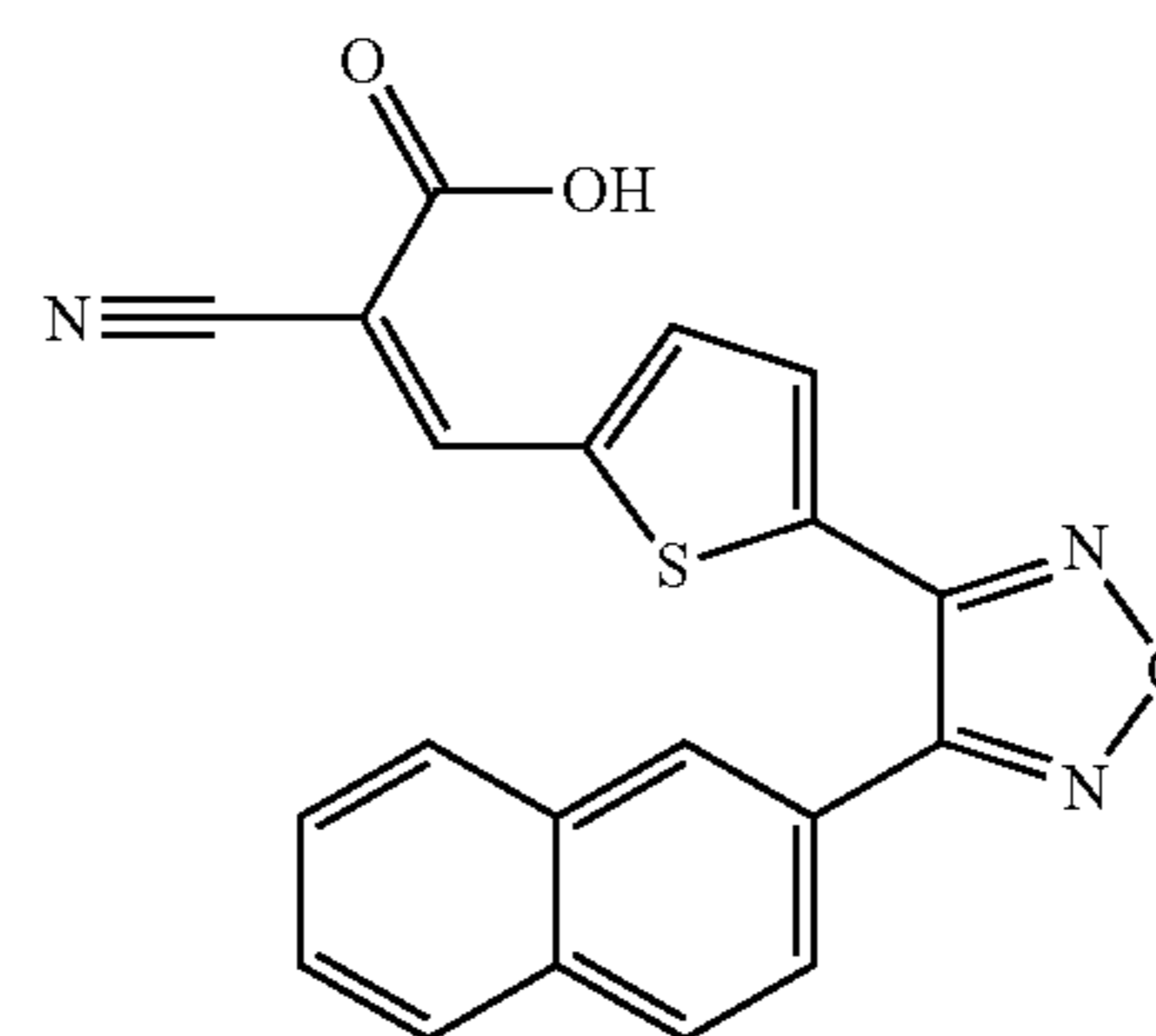
(Z)-2-cyano-3-(5-(4-(naphthalen-2-yl)-1,2,5-oxadiazol-3-yl)thiophen-2-yl)acrylic acid
