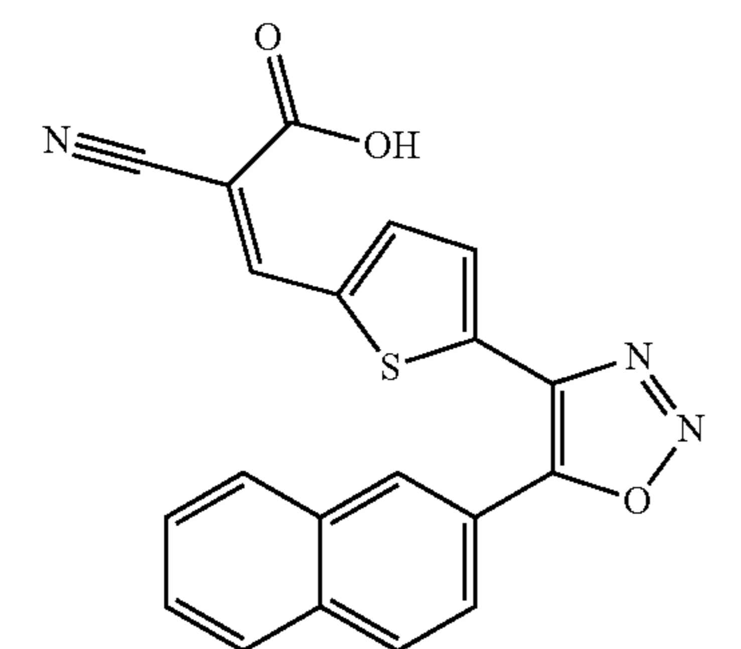
(Z)-2-cyano-3-(5-(5-(naphthalen-2-yl)-1,2,3-oxadiazol-4-yl)thiophen-2-yl)acrylic acid
