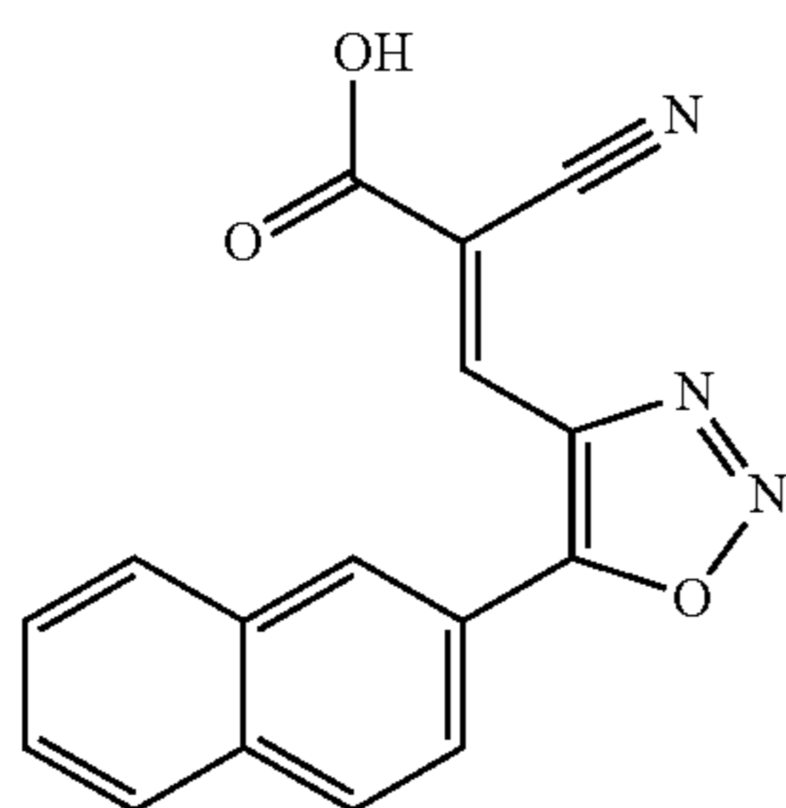
(E)-2-cyano-3-(5-(naphthalen-2-yl)-1,2,3-oxadiazol-4-yl)acrylic acid
