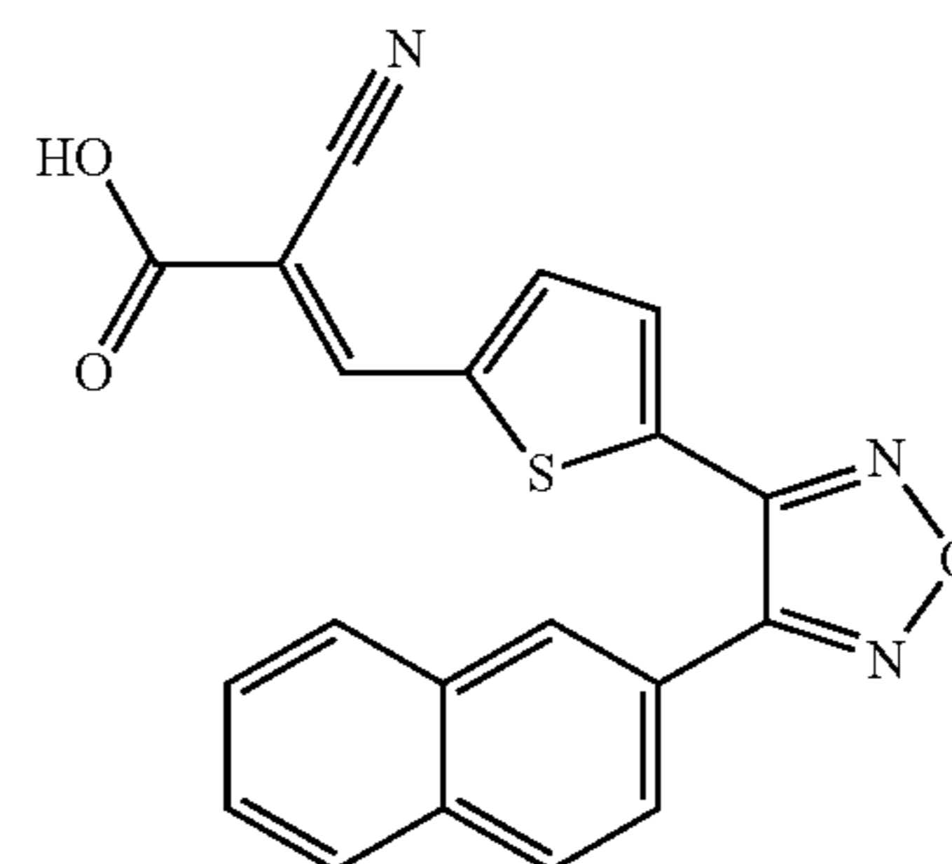
(E)-2-cyano-3-(5-(4-(naphthalen-2-yl)-1,2,5-oxadiazol-3-yl)thiophen-2-yl)acrylic acid
