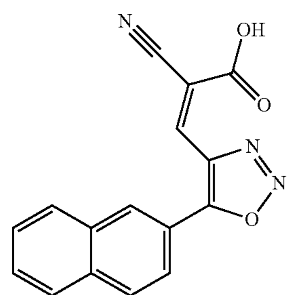
(Z)-2-cyano-3-(5-(naphthalen-2-yl)-1,2,3-oxadiazol-4-yl)acrylic acid
