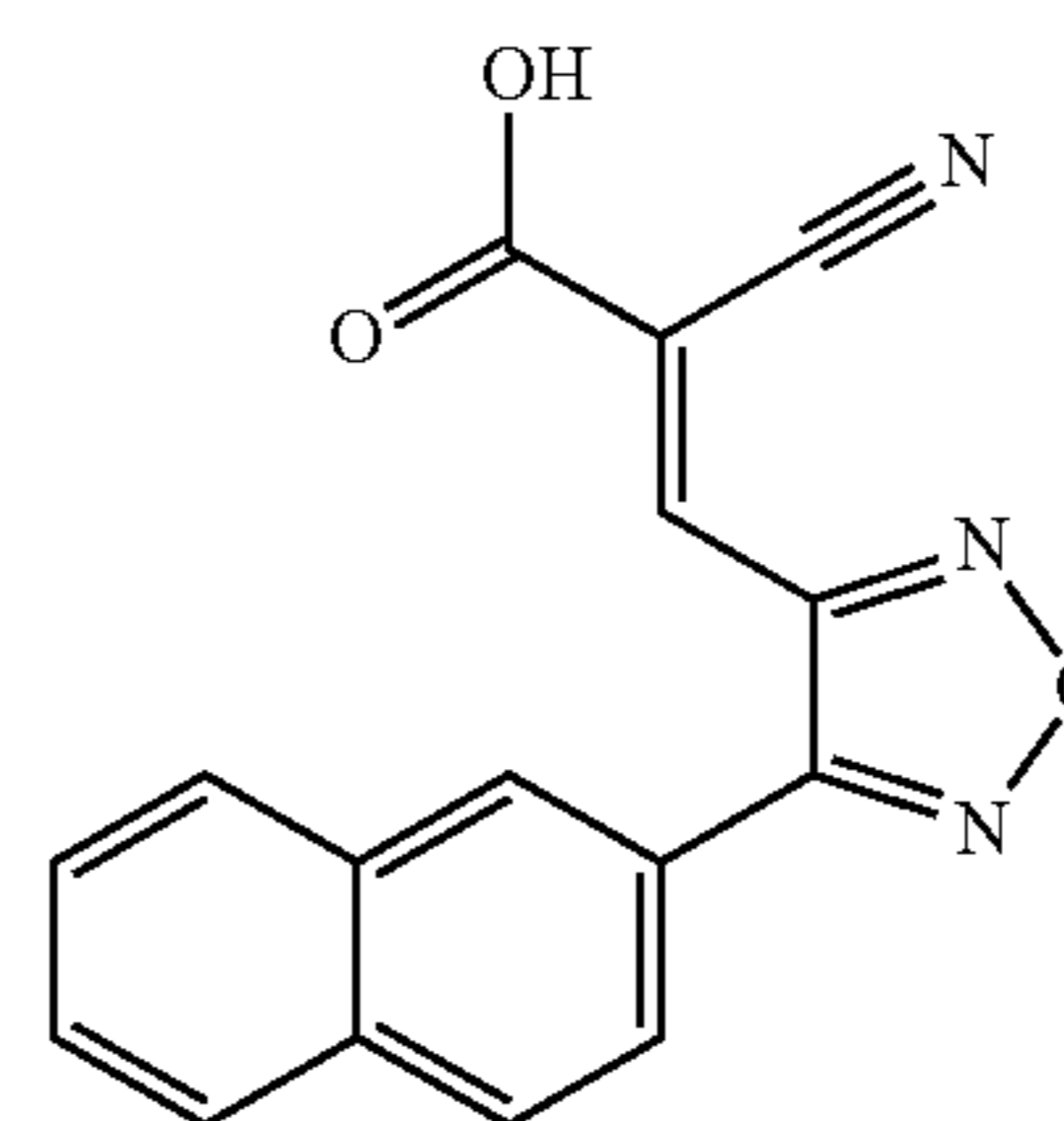
(E)-2-cyano-3-(4-(naphthalen-2-yl)-1,2,5-oxadiazol-3-yl)acrylic acid
