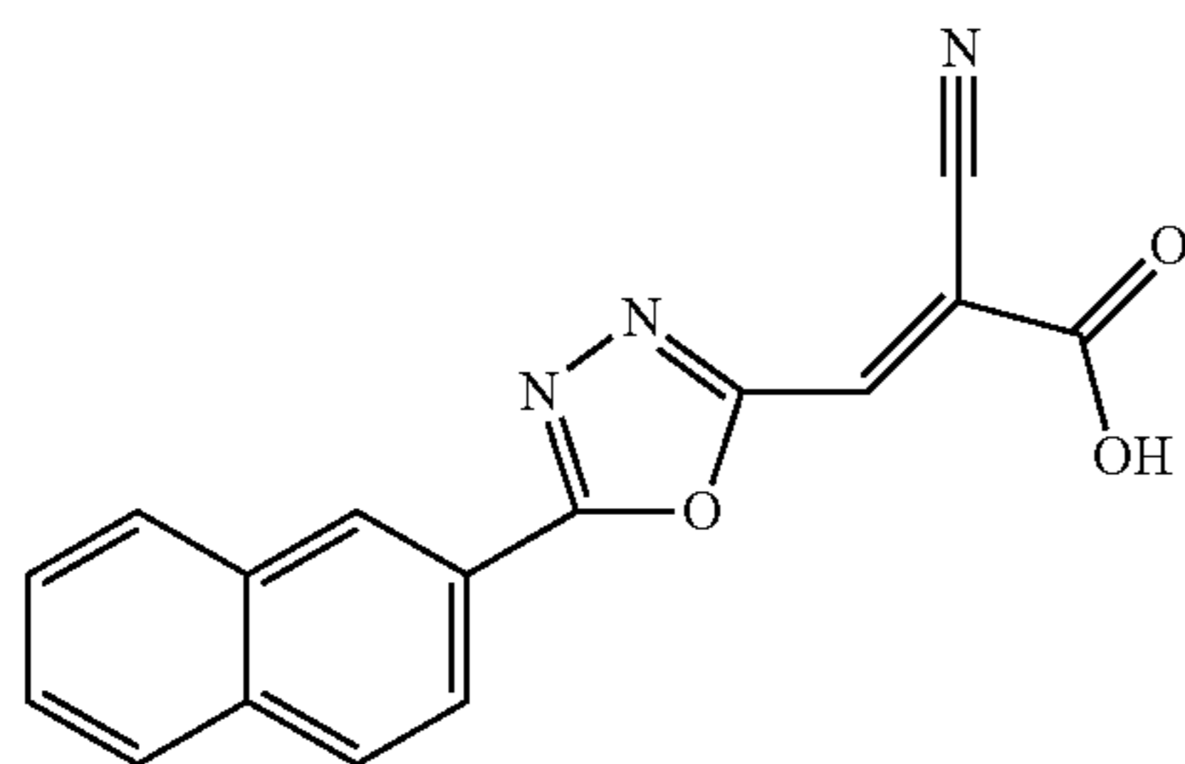
(E)-2-cyano-3-(5-(naphthalen-2-yl)-1,3,4-oxadiazol-2-yl)acrylic acid
