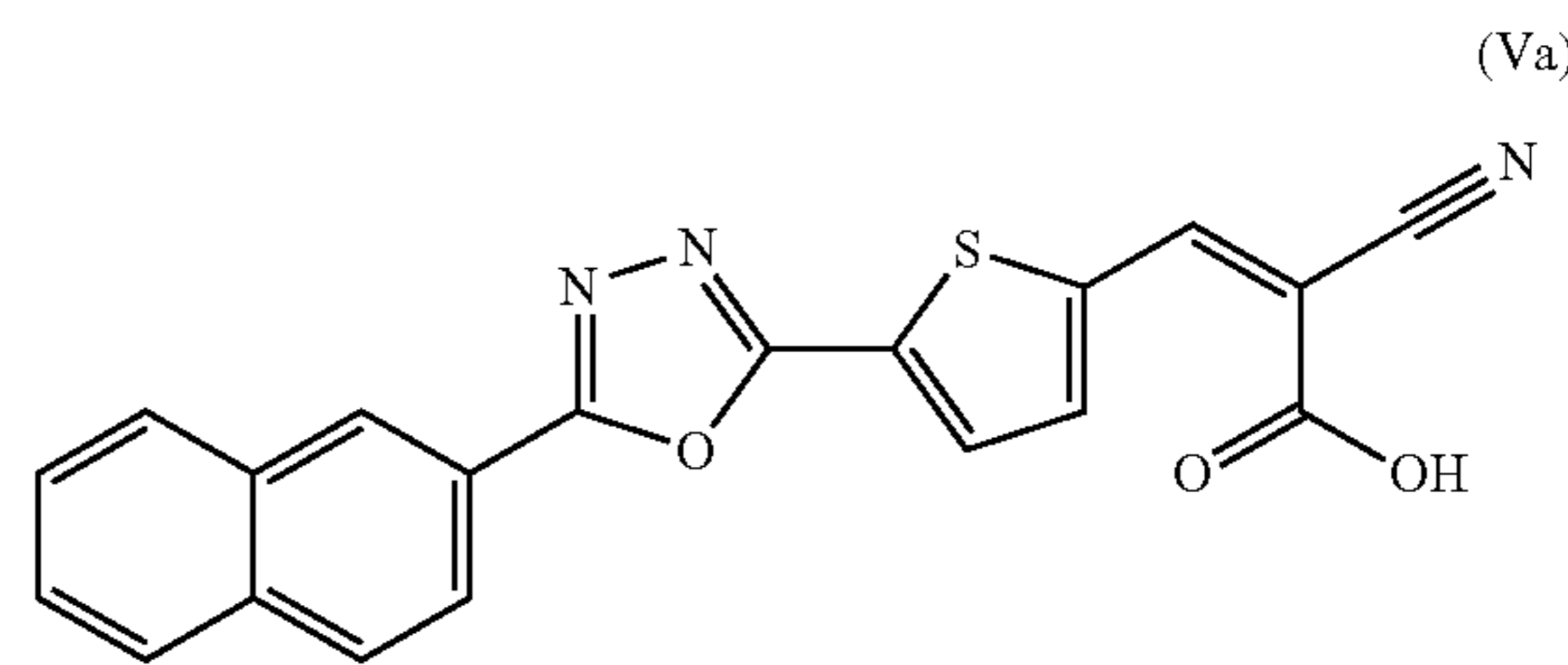
(Z)-2-cyano-3-(5-(5-(naphthalen-2-yl)-1,3,4-oxadiazol-2-yl)thiophen-2-yl)acrylic acid
