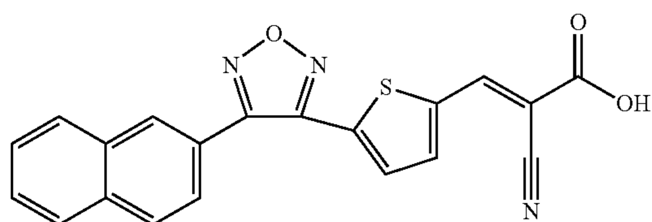
(E)-2-cyano-3-(5-(4-(naphthalen-2-yl)-1,2,5-oxadiazol-3-yl)thiophen-2-yl)acrylic acid
