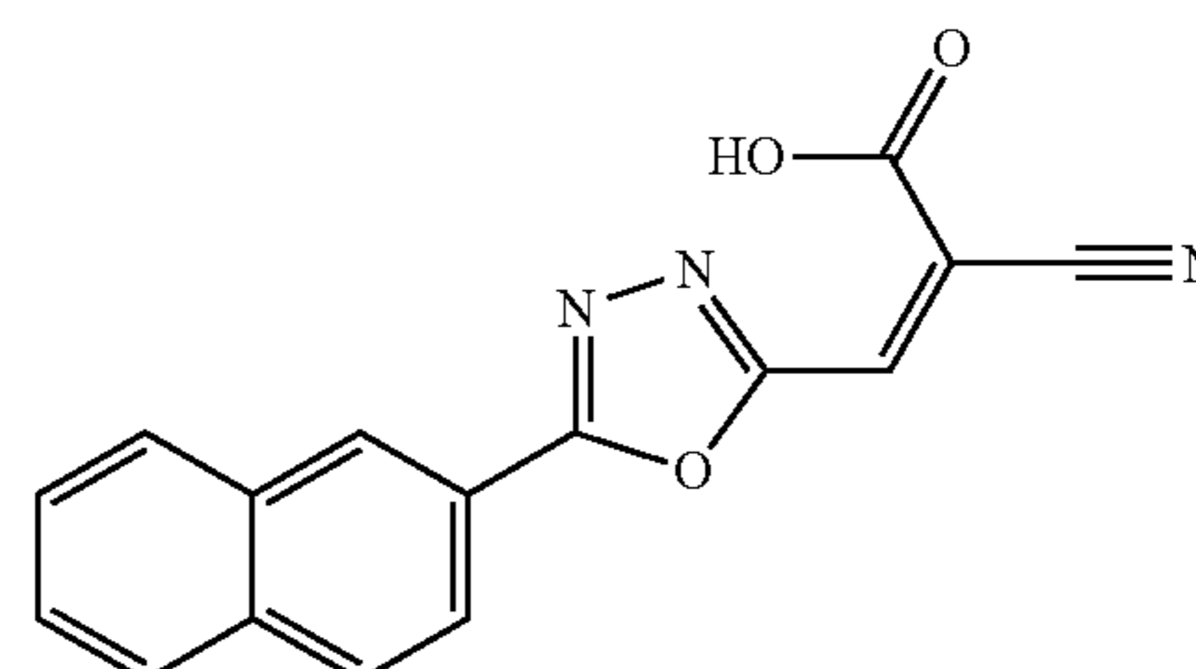
(Z)-2-cyano-3-(5-(naphthalen-2-yl)-1,3,4-oxadiazol-2-yl)acrylic acid
