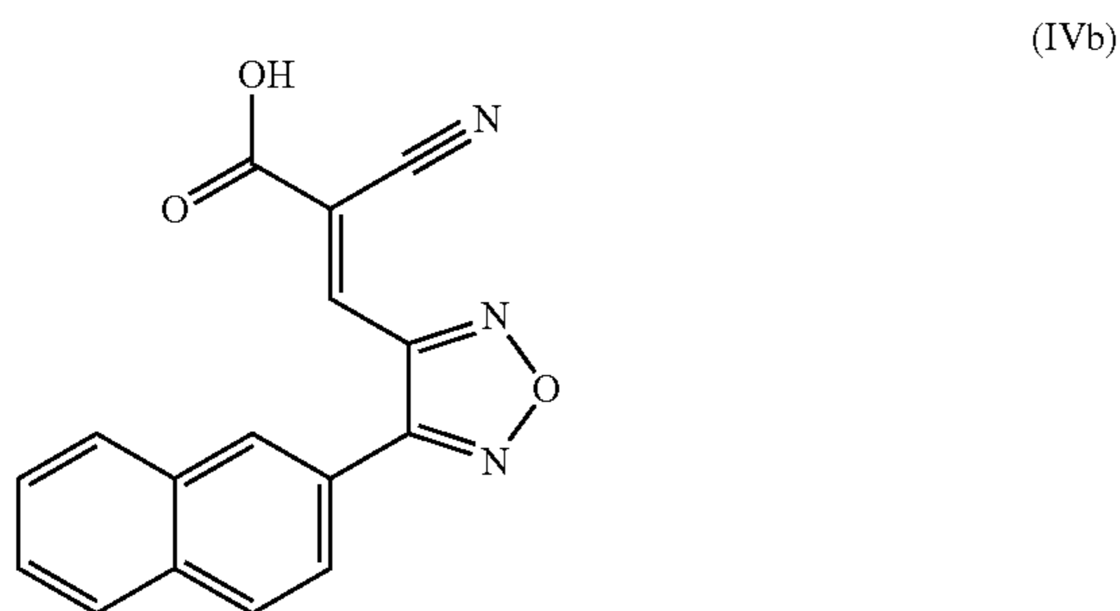
(E)-2-cyano-3-(4-(naphthalen-2-yl)-1,2,5-oxadiazol-3-yl)acrylic acid
