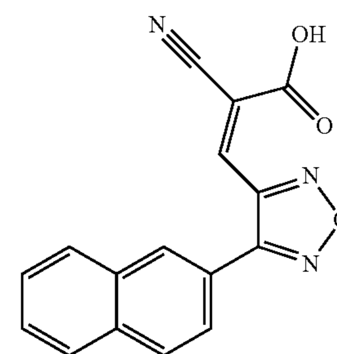
(Z)-2-cyano-3-(4-(naphthalen-2-yl)-1,2,5-oxadiazol-3-yl)acrylic acid
