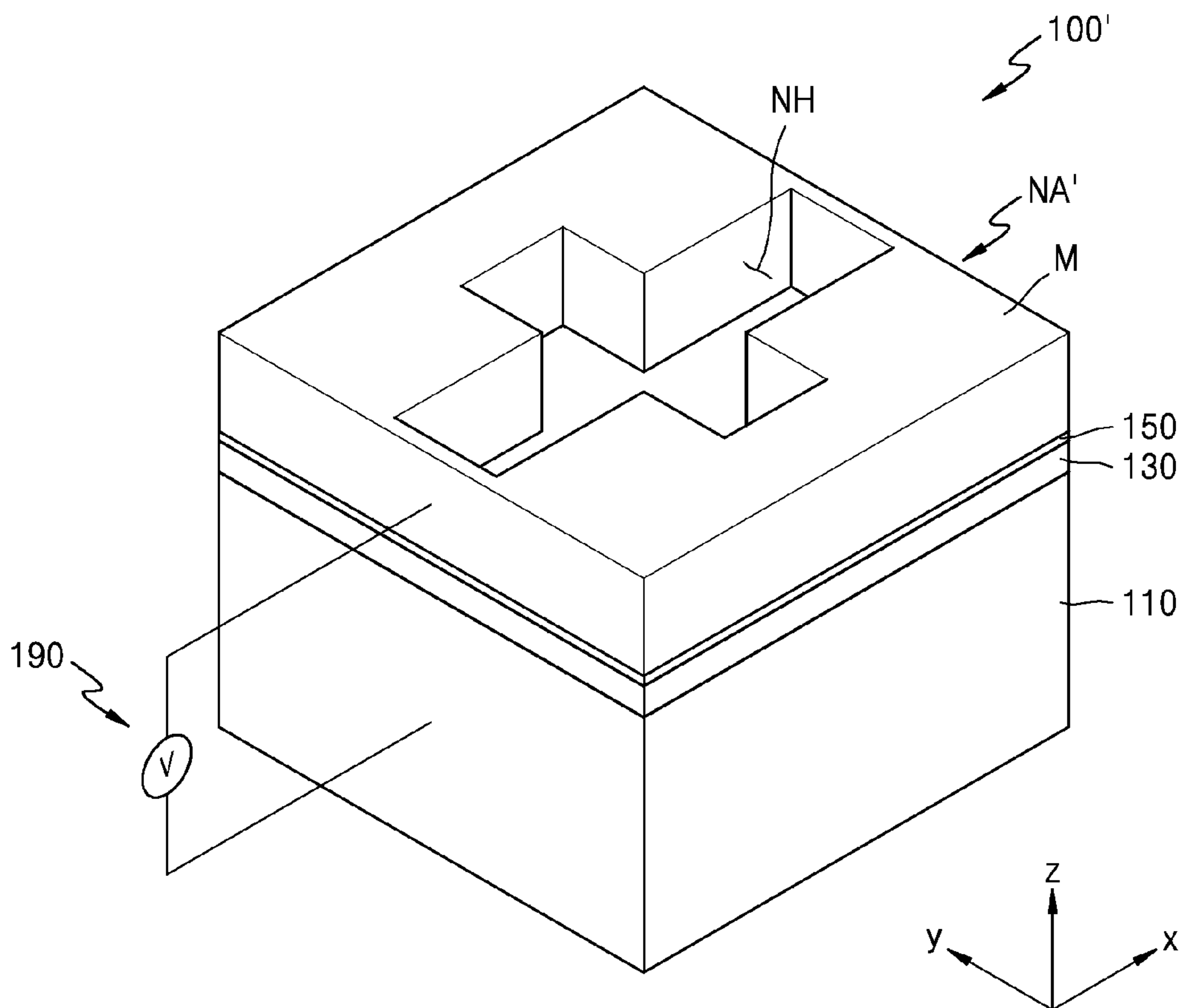
FIG. 16
