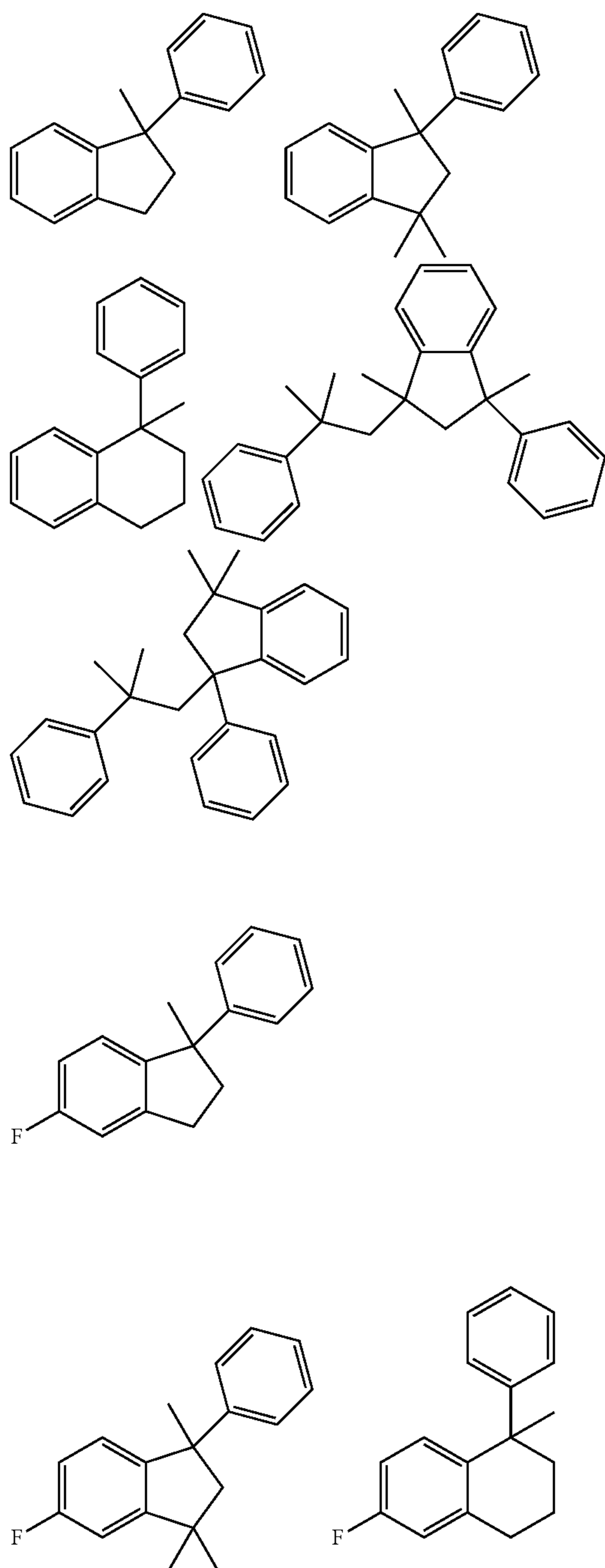
[Chem. 6]
