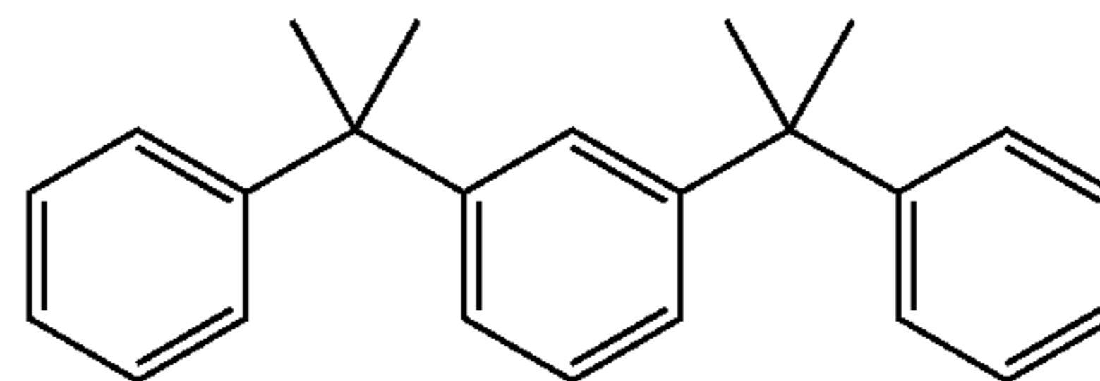
1,3-Bis(1-methyl-1-phenylethyl)-benzene
